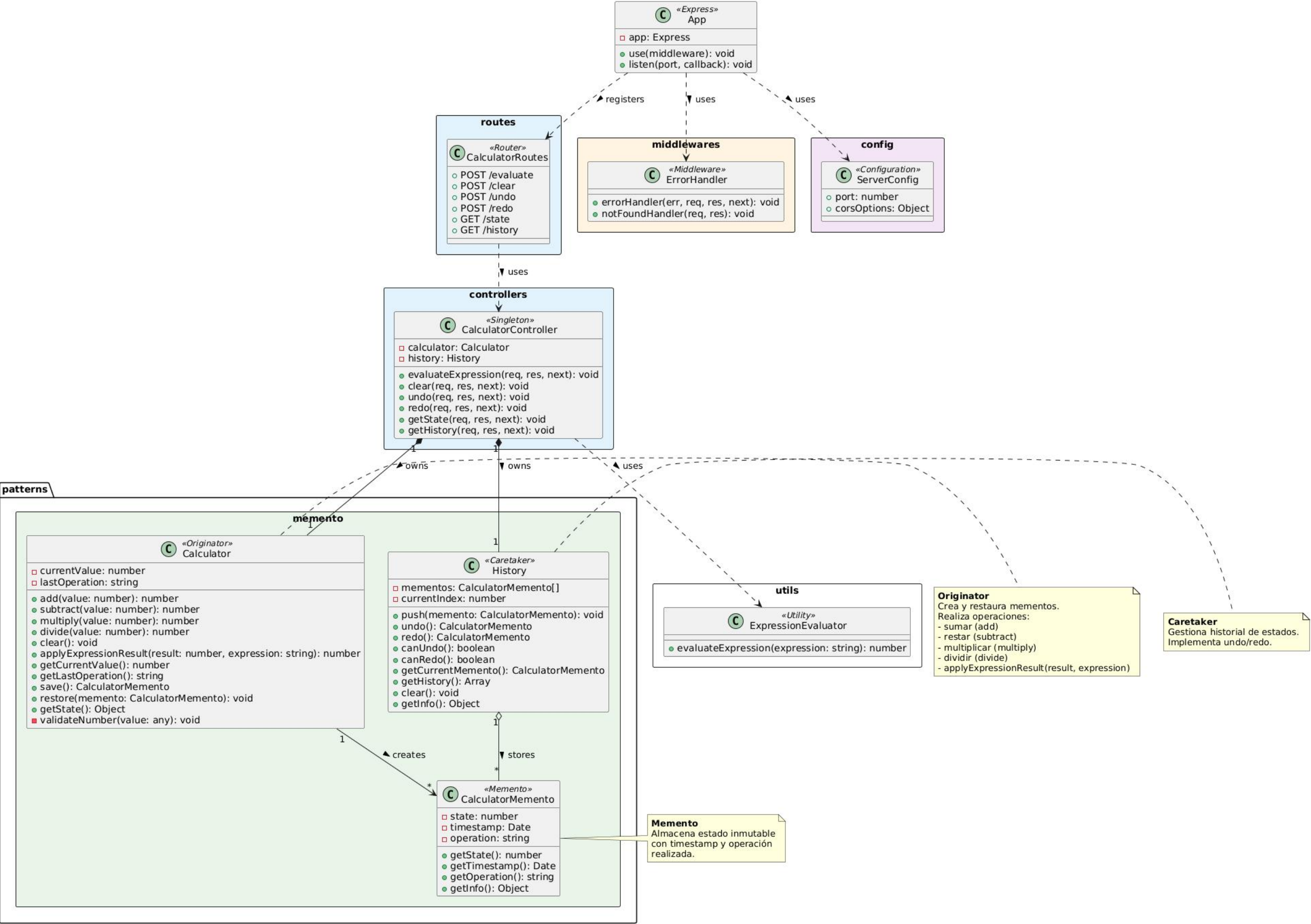
Diagrama de Clases - Calculadora con Patrón Memento
