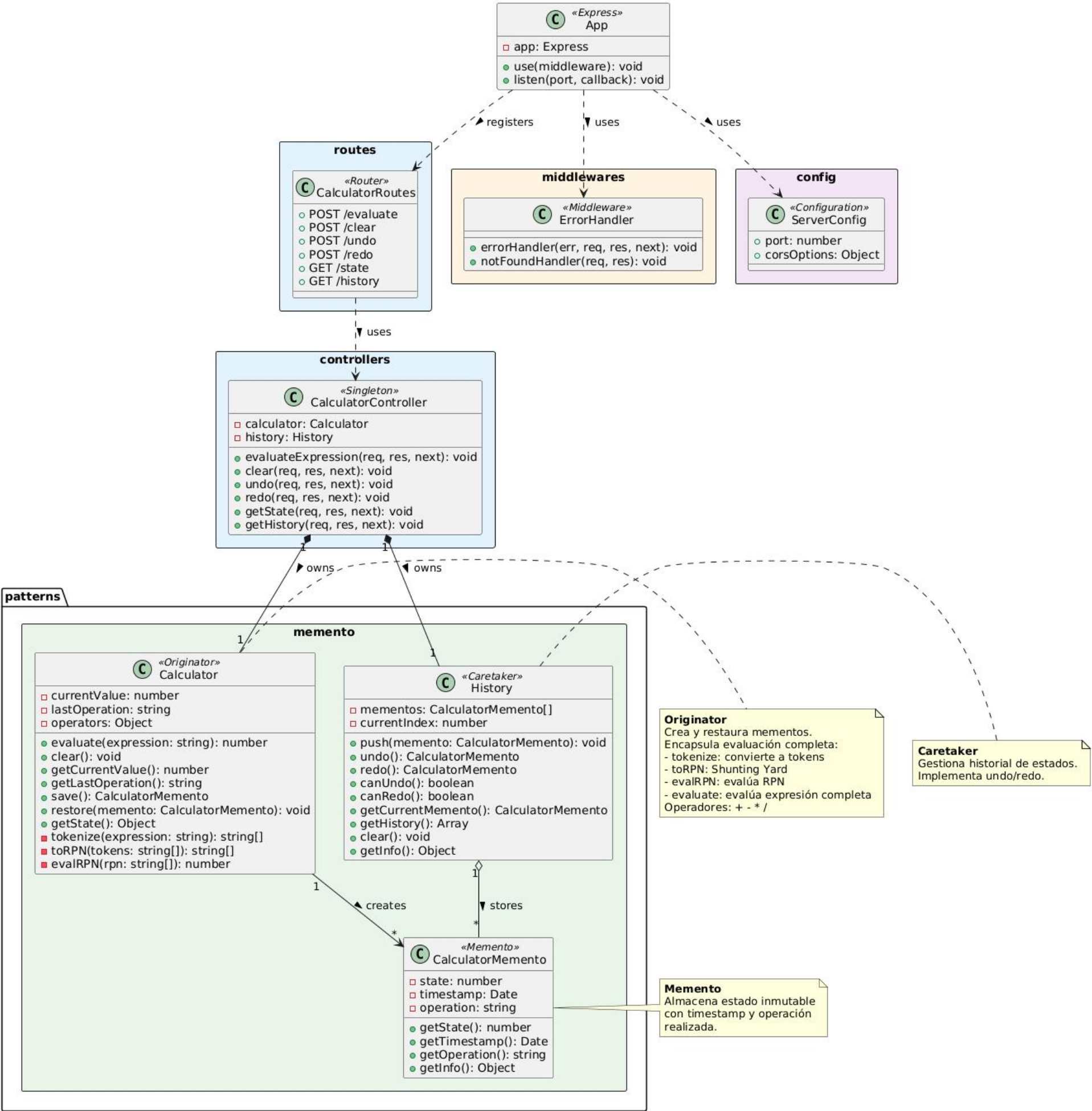
Diagrama de Clases - Calculadora con Patrón Memento
