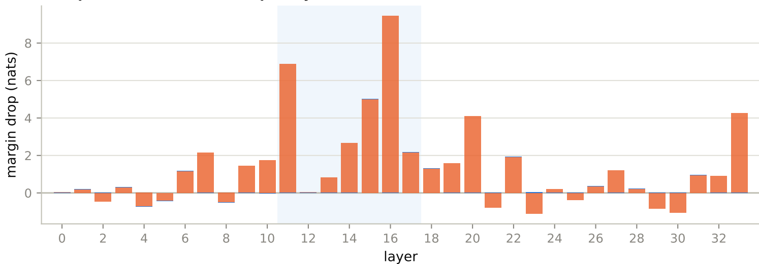
b. Top-200 feature ablation, per layer (n = 256)
