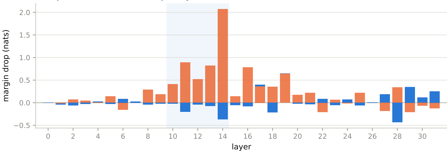
b. Top-200 feature ablation, per layer (n = 256)
