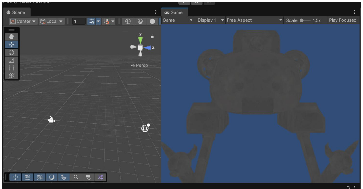
Рисунок 4 – Экспортированная модель
