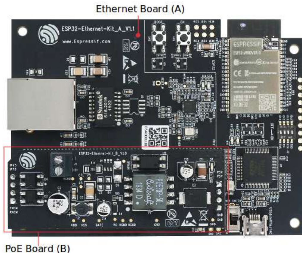
Fig. 12: ESP32-Ethernet-Kit v1.1
