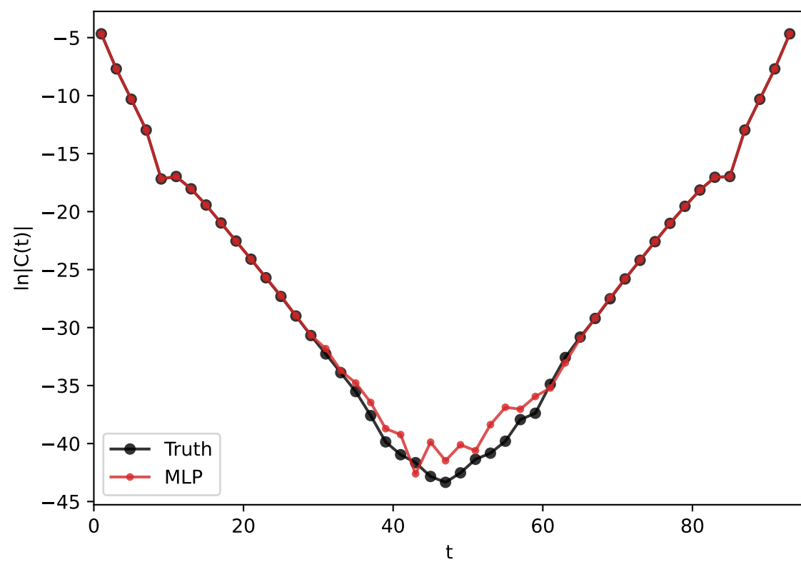
MLP: RM
