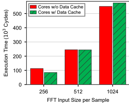
FFT
