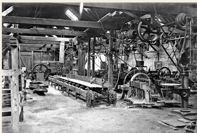
L'intérieur des ateliers de constructions mécaniques.
