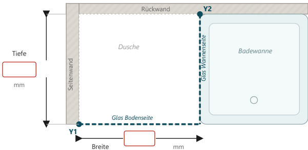
A · Grundriss von oben
