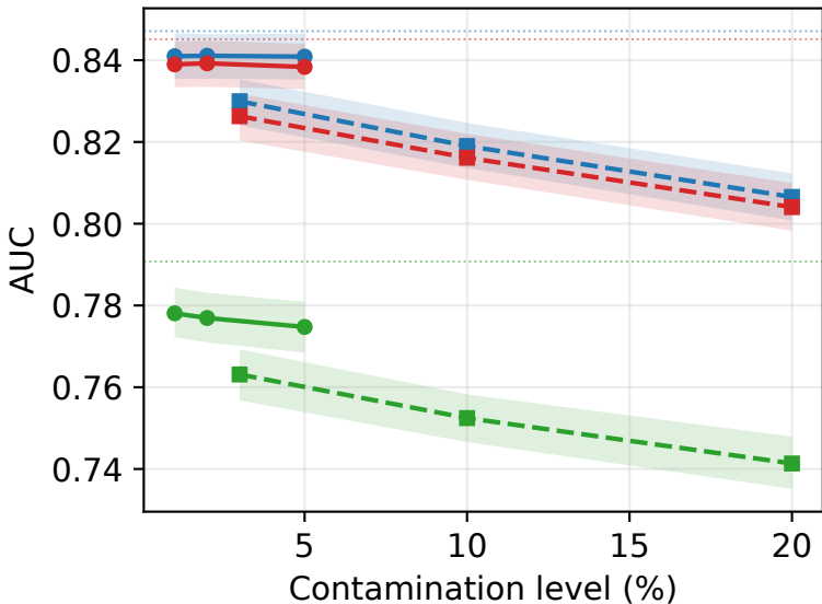
(a) AUC
