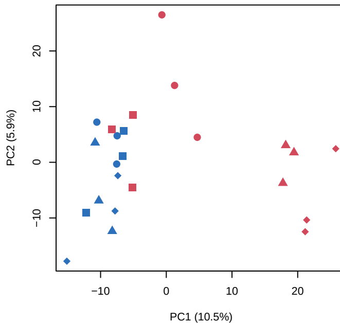
PCA: downshift
