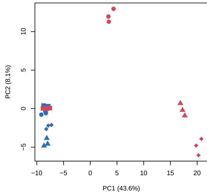
PCA: mixed
