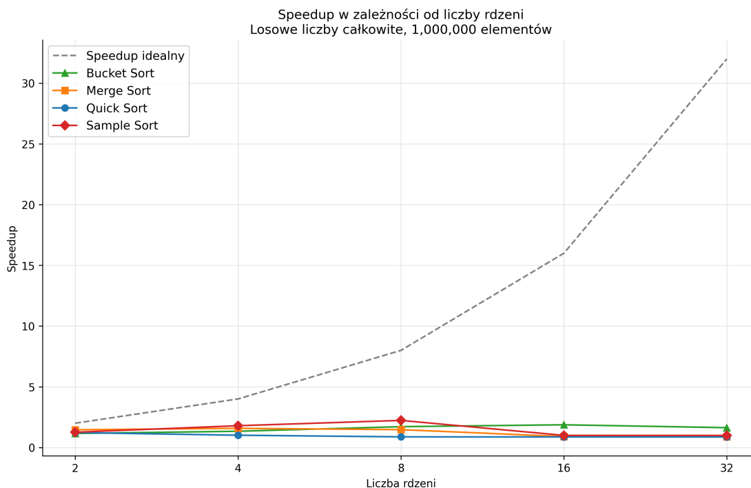
Rysunek 6.6: Przyspieszenie badanych algorytmów dla zbioru random_int o rozmiarze 1 000 000 elementów w zależności od liczby jednostek wykonawczych. Źródło: opracowanie własne.
