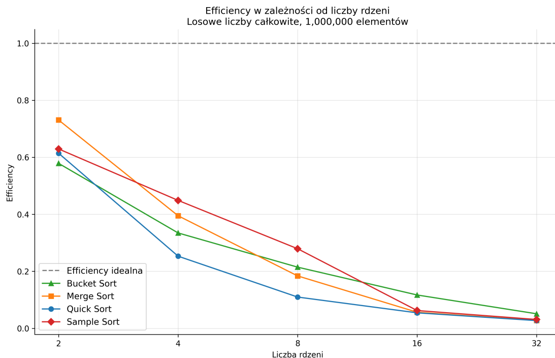
Rysunek 6.7: Efektywność badanych algorytmów dla zbioru random_int o rozmiarze 1 000 000 elementów w zależności od liczby jednostek wykonawczych. Źródło: opracowanie własne.
