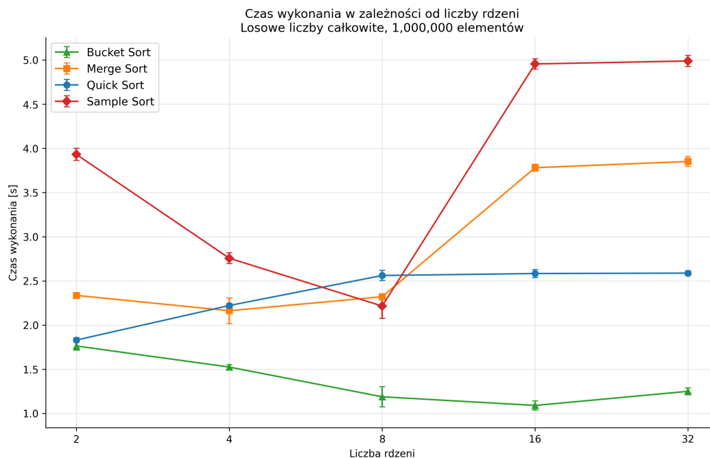
Rysunek 6.2: Średni czas wykonania wariantów równoległych dla zbioru random_int o rozmiarze 1 000 000 elementów w zależności od liczby jednostek wykonawczych. Źródło: opracowanie własne.
