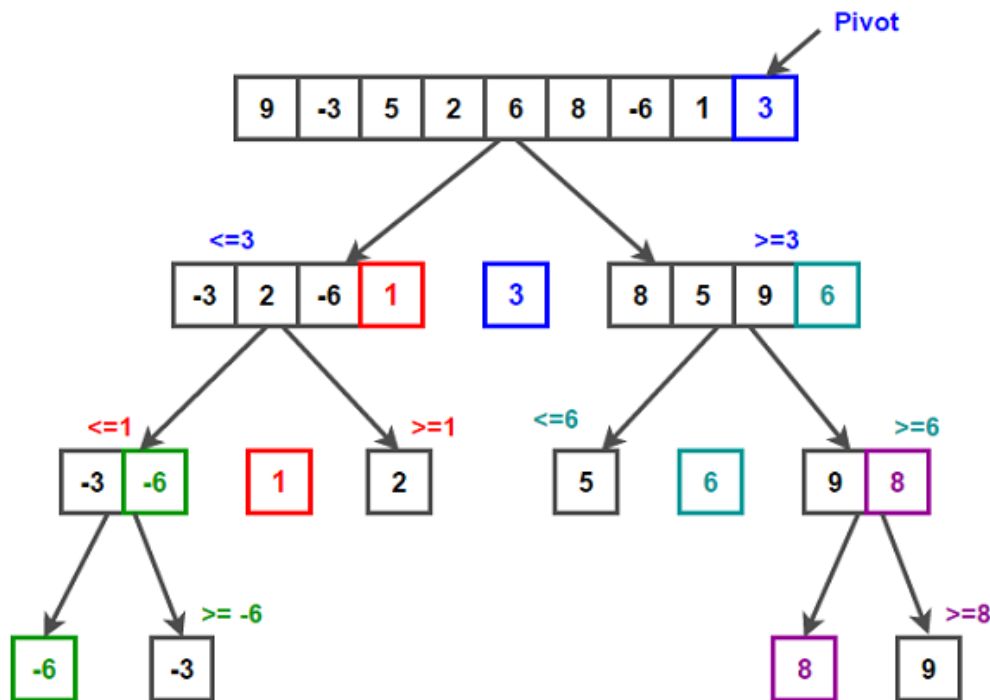
Rysunek 3.1: Schemat działania Quick Sort. Źródło: https://medium.com/@lucky_rydar/parallel-quick-sort-on-c-a3526ba8b532 .
