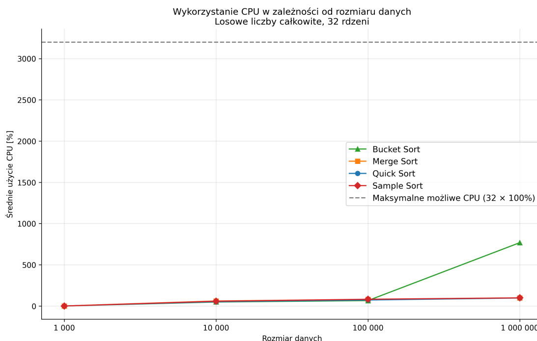
Rysunek 6.4: Średnie wykorzystanie CPU w zależności od rozmiaru zbioru random_int dla 32 jednostek wykonawczych. Źródło: opracowanie własne.
