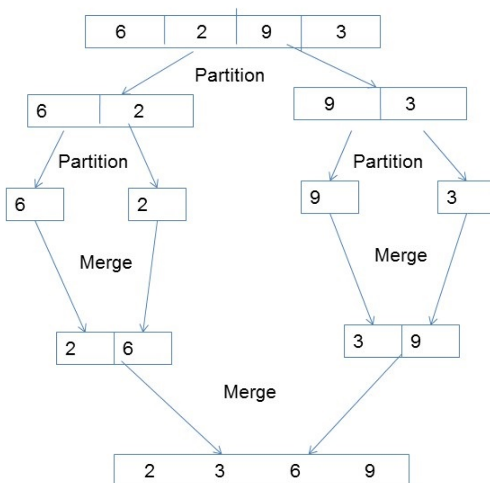
Rysunek 3.2: Schemat działania Merge Sort. Źródło: https://www.tutorialspoint.com.cache3.com/parallel_algorithm/parallel_algorithm_quick_guide.htm .
