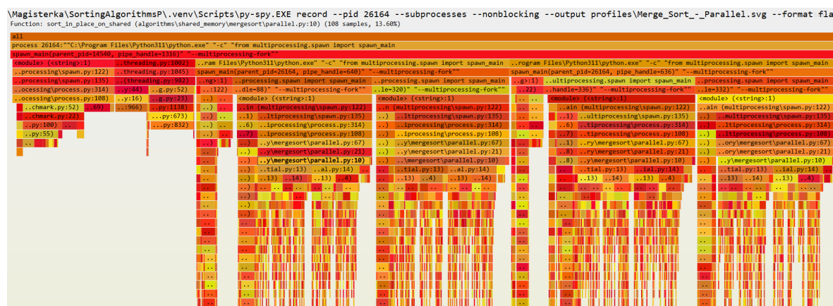
Rysunek 7.1: Wykres płomieni dla równoległej implementacji Merge Sort uzyskany za pomocą narzędzia py-spy
