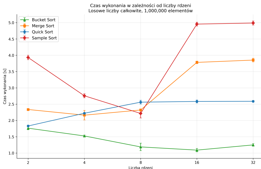
Rysunek 6.2: Średni czas wykonania wariantów równoległych dla zbioru random_int w zależności od liczby jednostek wykonawczych.
