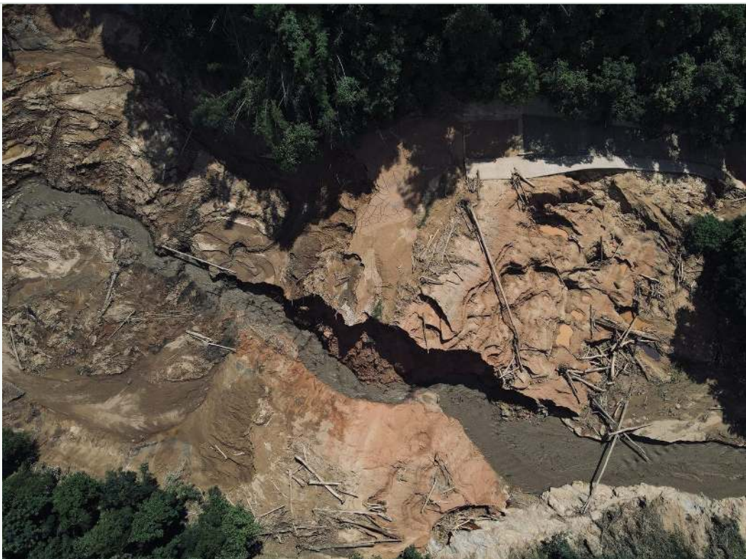
DRONE SURVEY · 08.09.2568 ร่องน้ำกัดเซาะต่อเนื่องสันทำนบอ่างเก็บน้ำห้วยโป่ง
