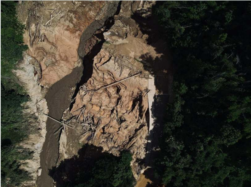
DRONE SURVEY · 08.09.2568 จุดที่เสียหายสันทำนบอ่างเก็บน้ำห้วยโป่ง
