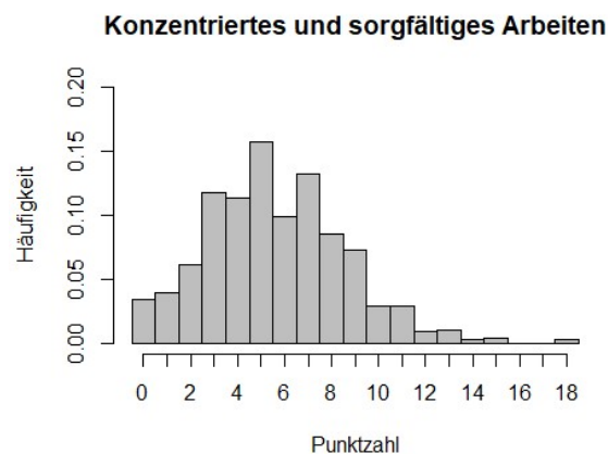
Histogramm 10: Verteilung der erreichten Punktzahlen bei konzentriertes und sorgfältiges Arbeiten (von 742 Resultaten)
