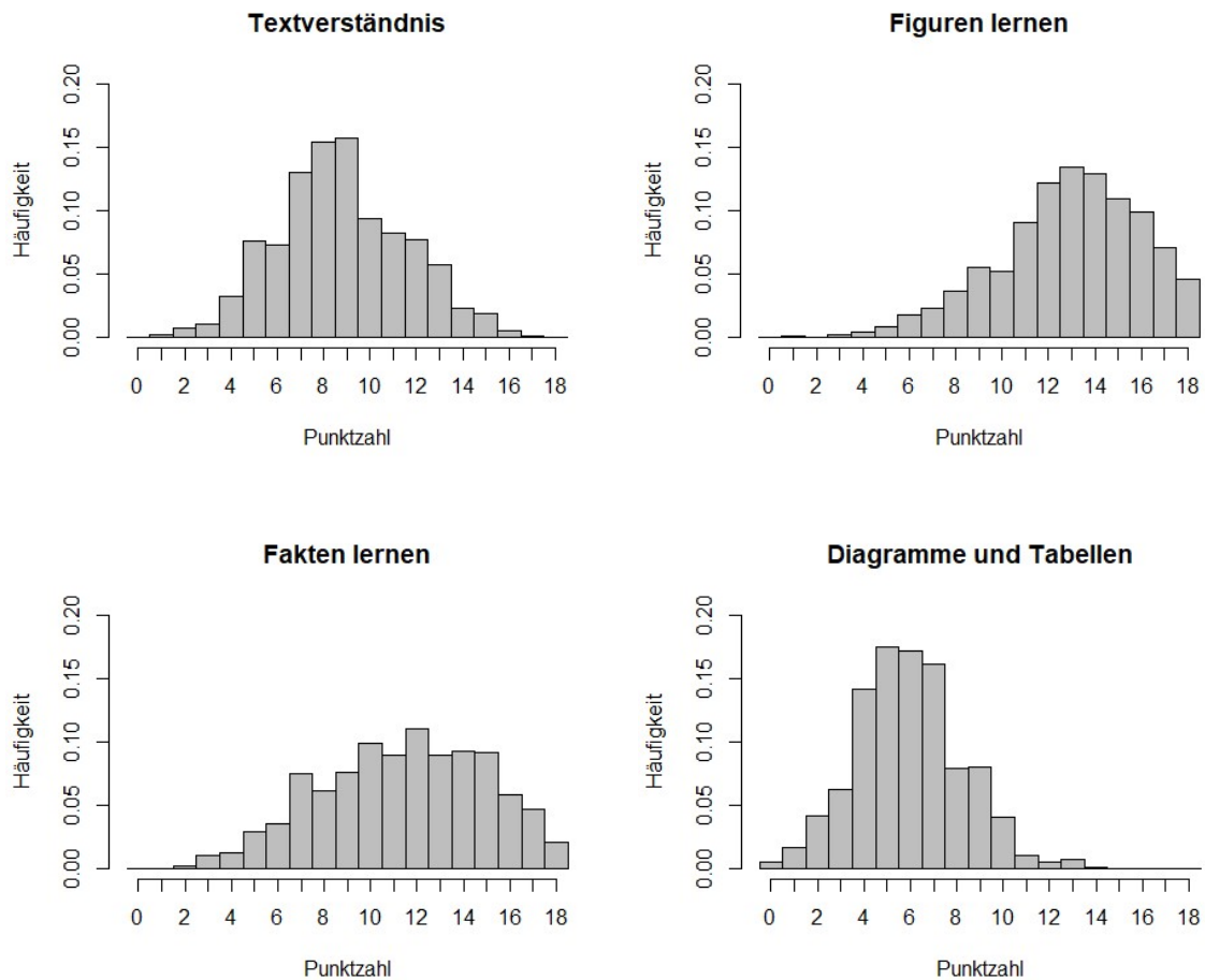
Histogramme 2-9: Verteilungen der erreichten Punktzahlen bei den einzelnen Untertests (von 1048 Resultaten)
