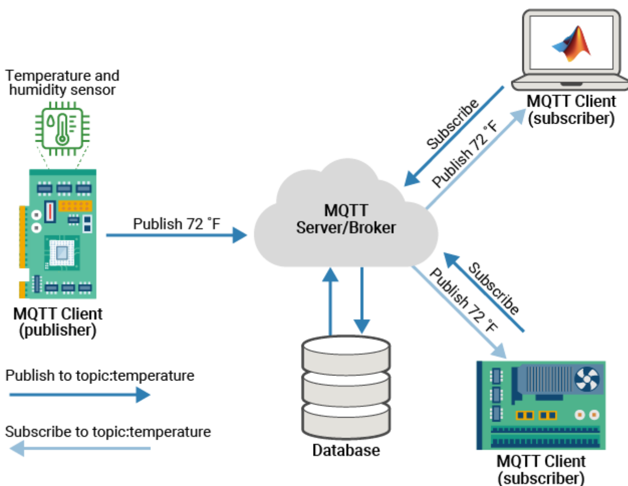
Рисунок 2.1 – Архитектура системы
