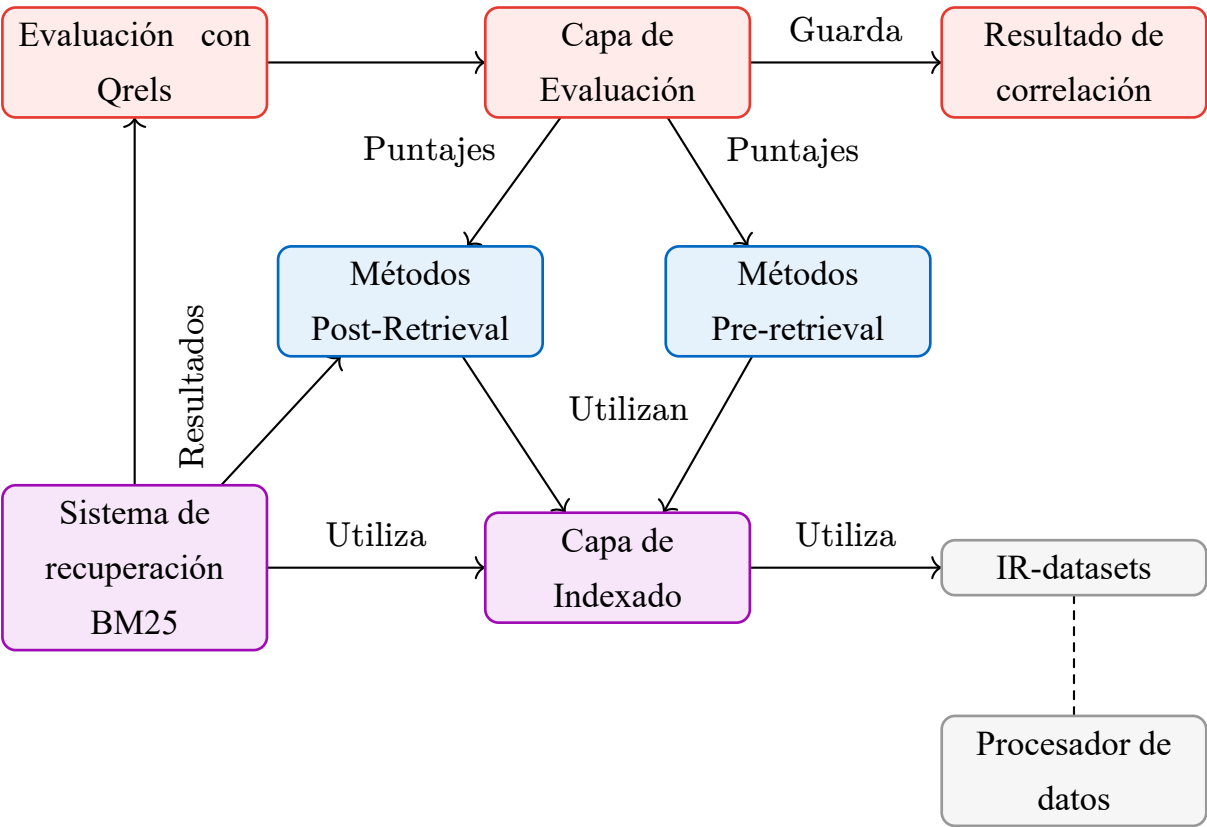
Figura 5.1: Diagrama de componentes del entorno de evaluación
