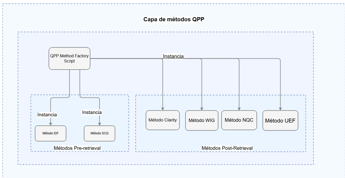
Figura 5.5: Diagrama de la capa de métodos QPP
