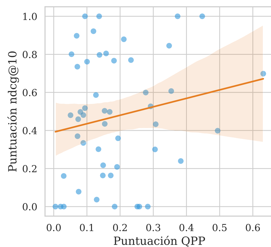
UEF-NQC \tau = 0.1082
