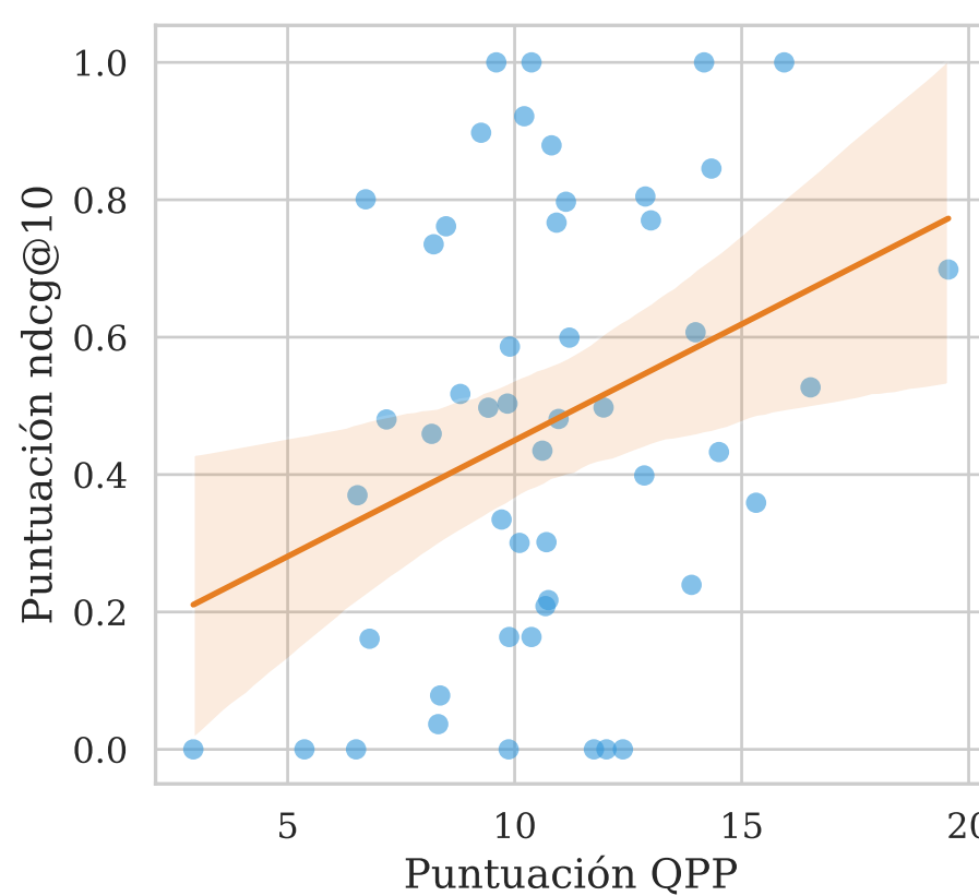
WIG \tau = 0.2007
