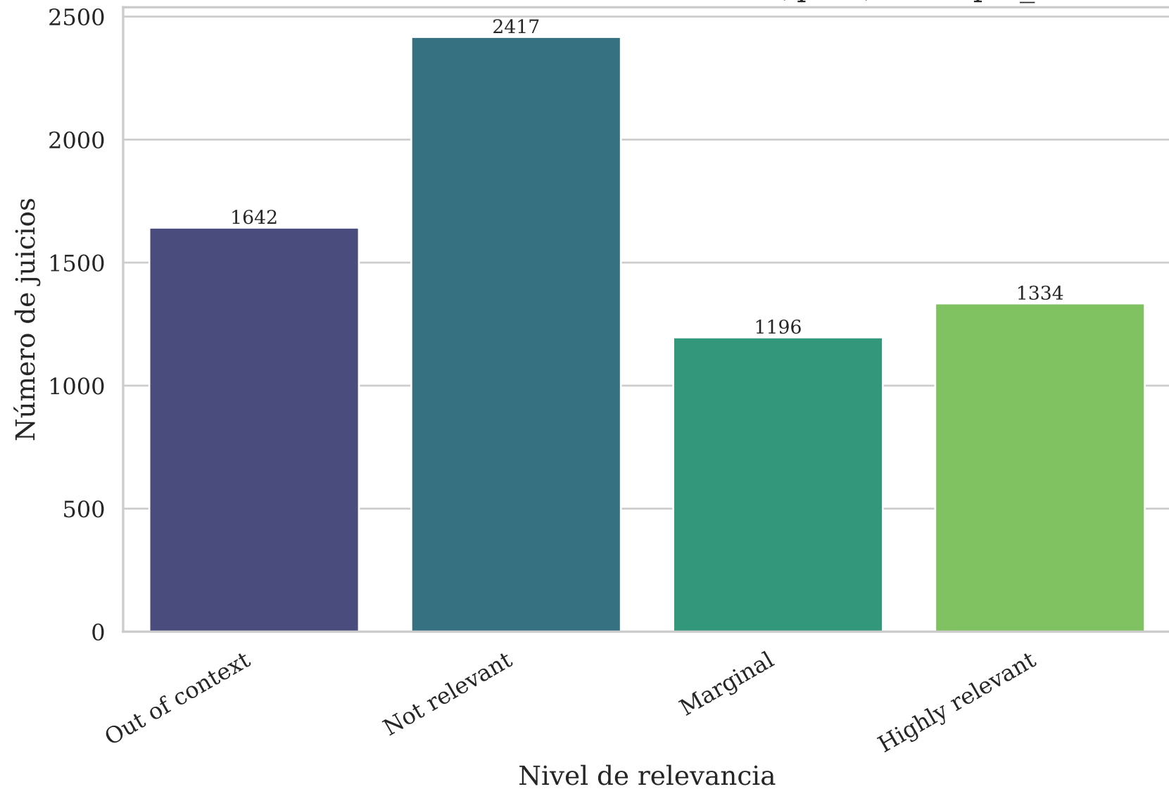
Distribución de niveles de relevancia (qrels) - antique_test
