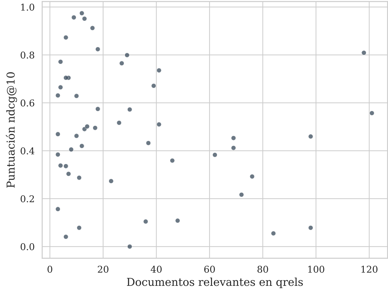
Número de documentos relevantes vs. rendimiento (ndcg@10) por consulta
