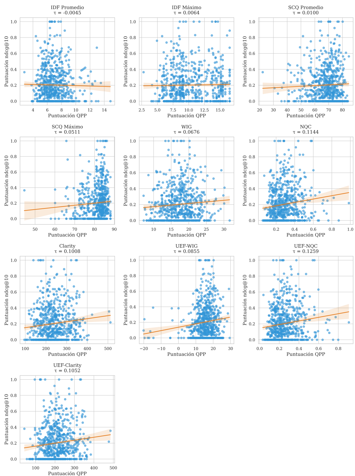
Figura 6.6: Diagramas de dispersión QPP vs nDCG@10 en CAR.
