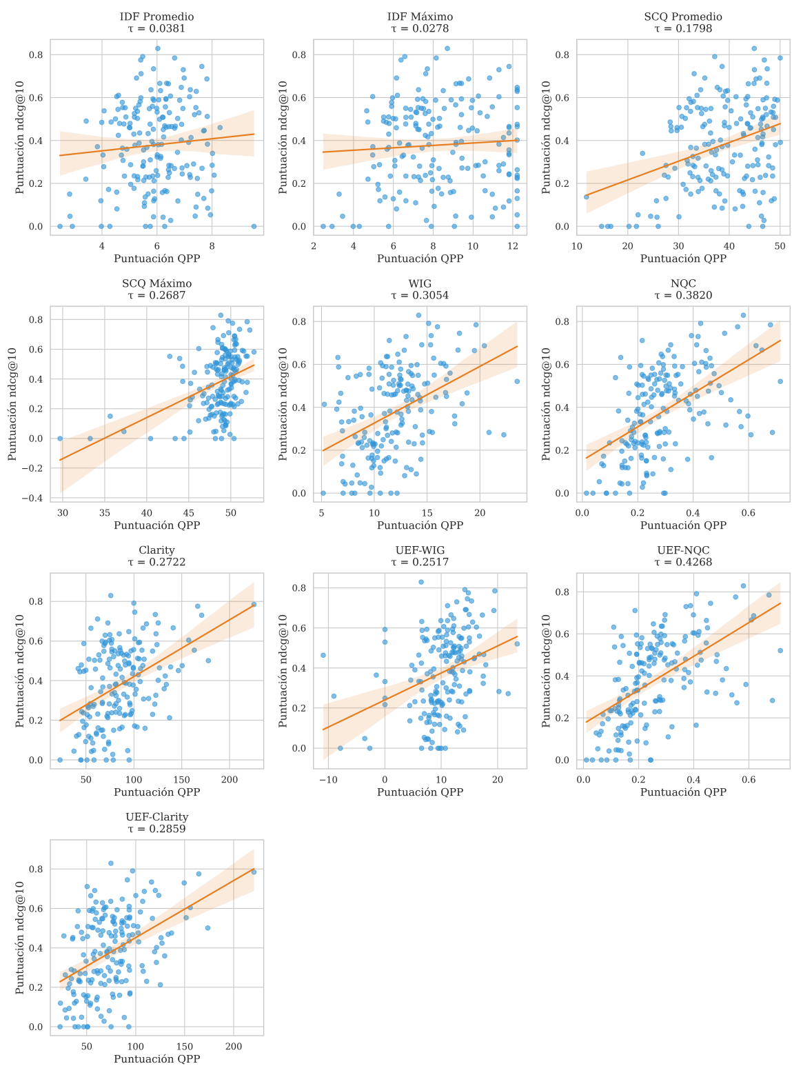
Figura 6.5: Diagramas de dispersión QPP vs nDCG@10 en Antique/Test.
