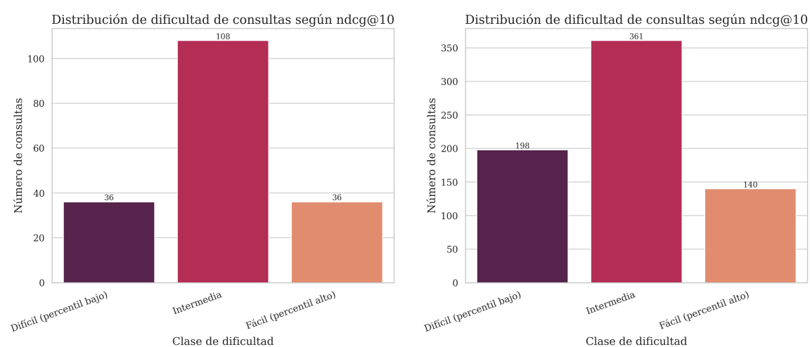
Figura 6.3: Distribución de dificultad de consultas: Antique/Test (izq.) vs CAR (der.).
