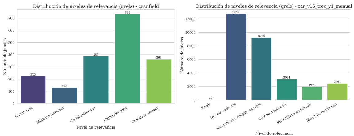
Figura 6.2: Contraste en distribución de relevancia: Cranfield (izq.) vs CAR (der.).
