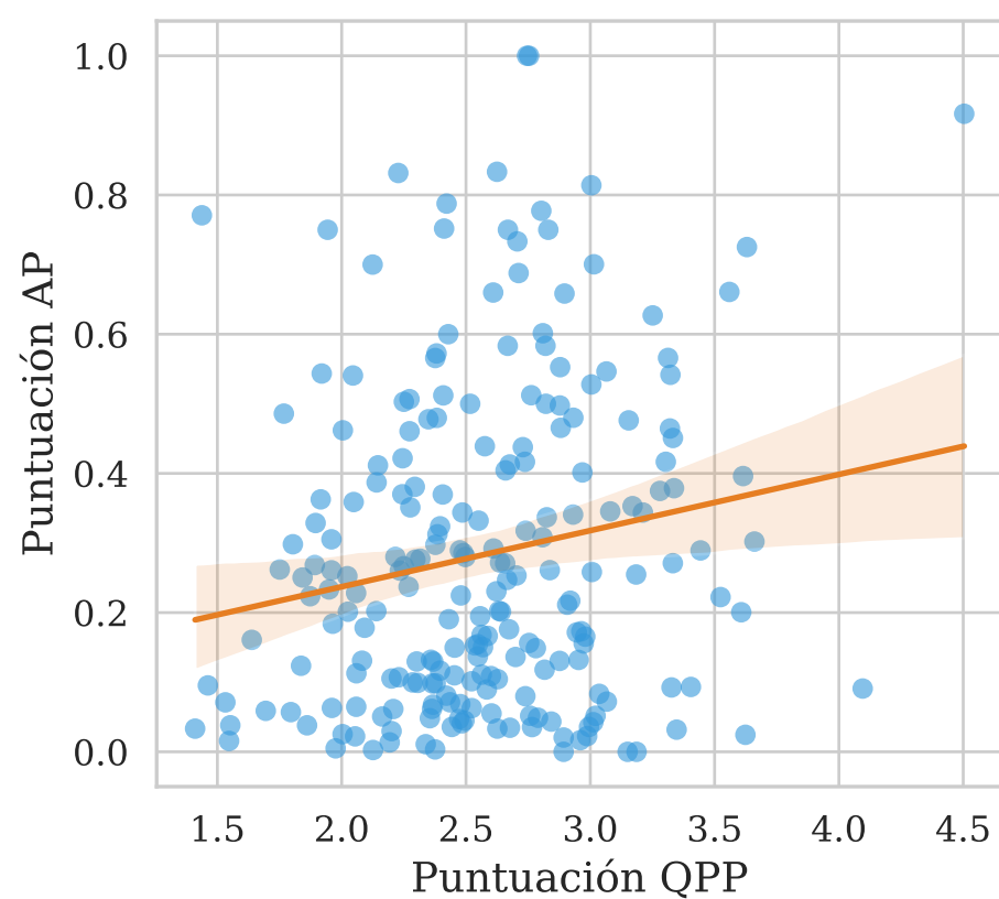
SCQ Máximo \tau = 0.1829
