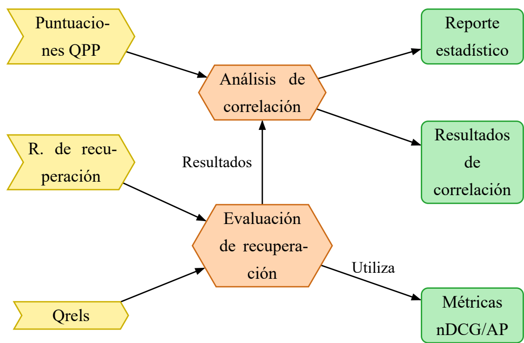
Figura 6.7: Diagrama de flujo del análisis de resultados
