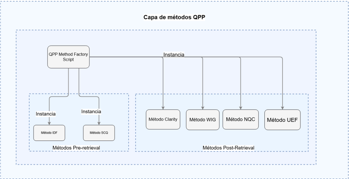
Figura 5.5: Diagrama de la capa de métodos QPP
