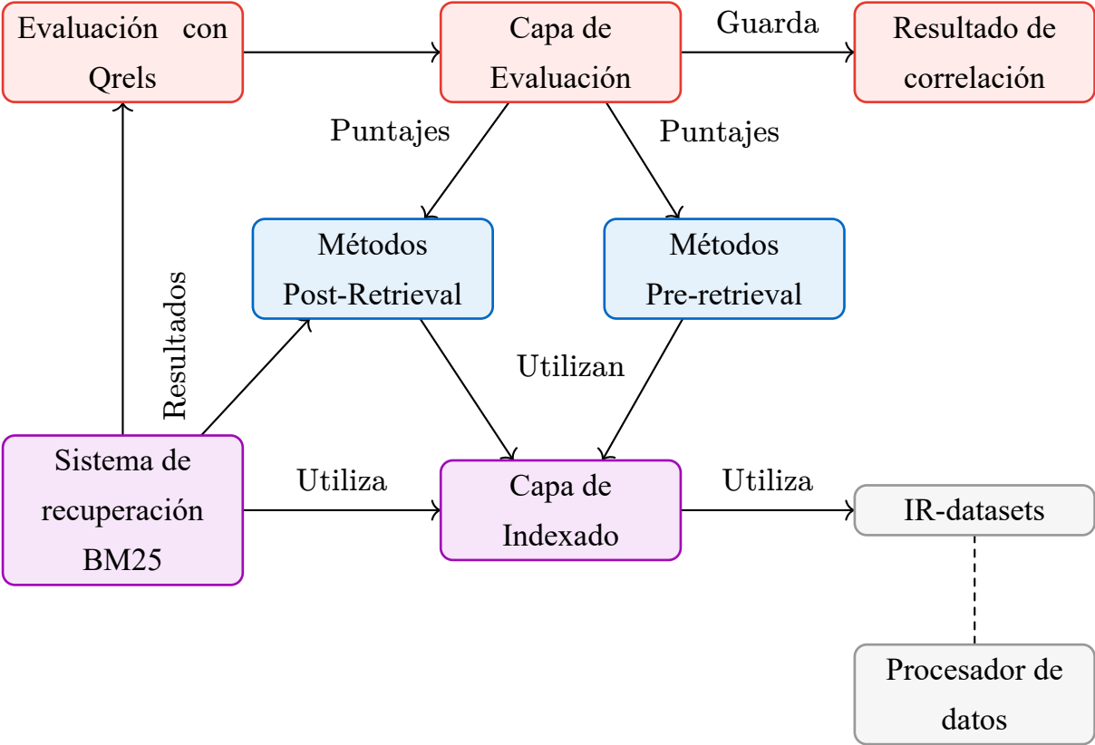
Figura 5.1: Diagrama de componentes del entorno de evaluación
