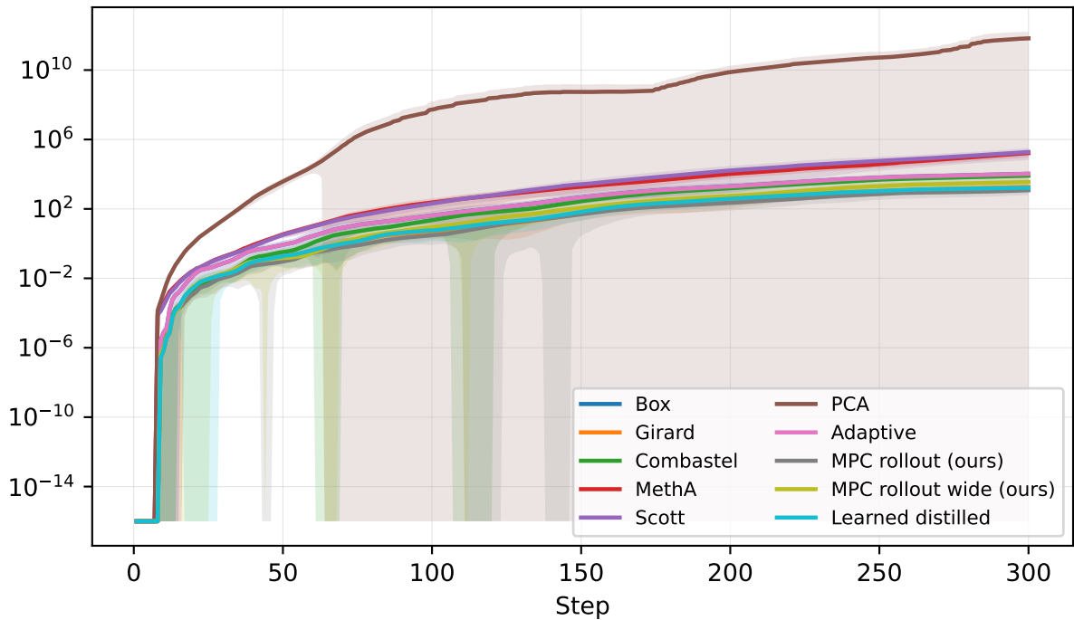
Interval-hull MSE
