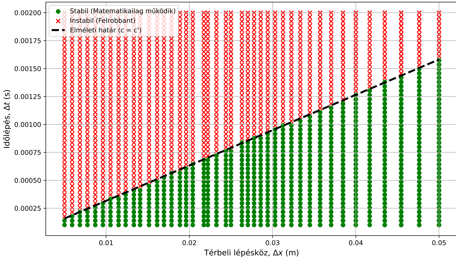
A numerikus hullámgyenlet stabilitási térképe
