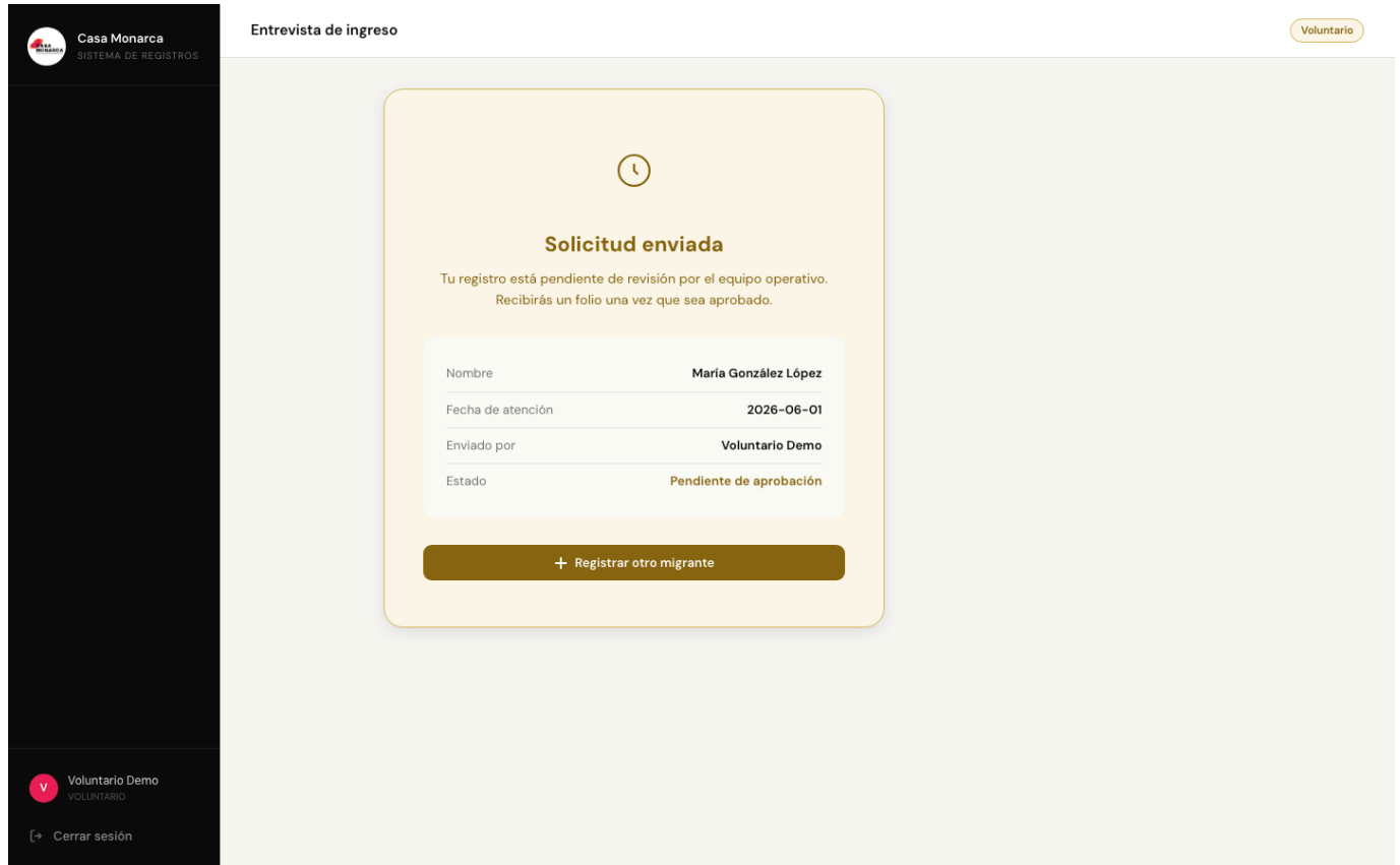
Figura 7 — Pantalla de confirmación (registro pendiente de revisión)
