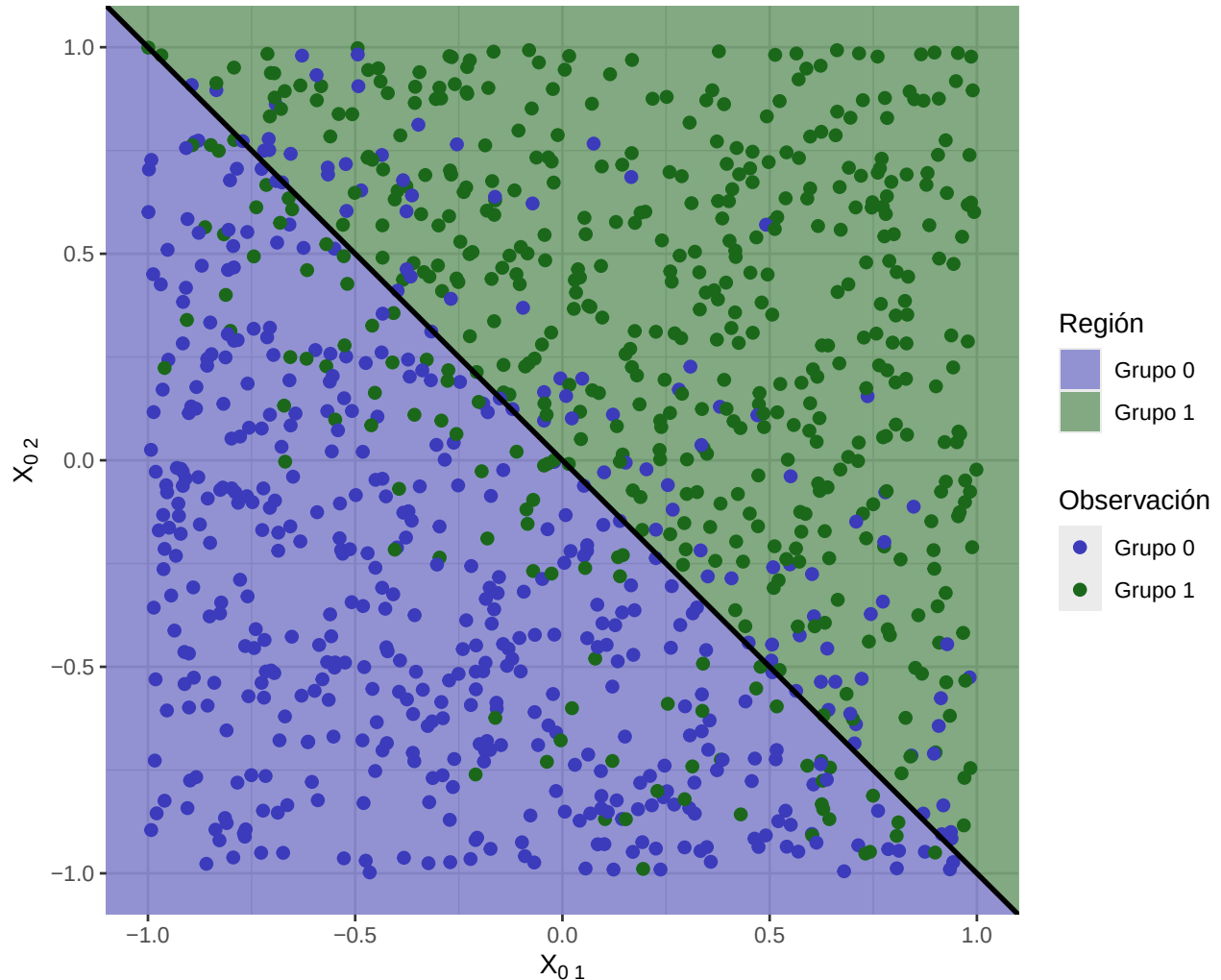
Figura 8.3: Muestra simulada con el clasificador logístico. Se usan 1,000 observaciones con X_{01} y X_{02} uniformes en [-1, 1] . La frontera de decisión X_{02} = -X_{01} aparece en negro; y las regiones correspondientes aparecen sombreadas. Notemos que la clasificación no es perfecta, pero el número de errores decrece de manera exponencial a medida que nos alejamos de la frontera de decisión
