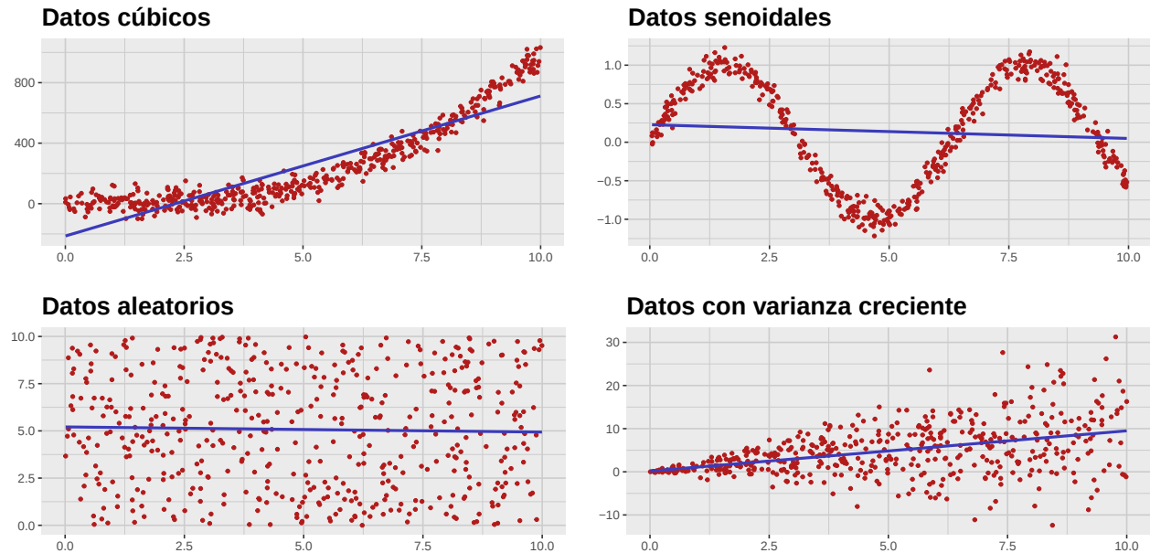
Figura 4.1: Ajuste por mínimos cuadrados para diferentes conjuntos de datos.
