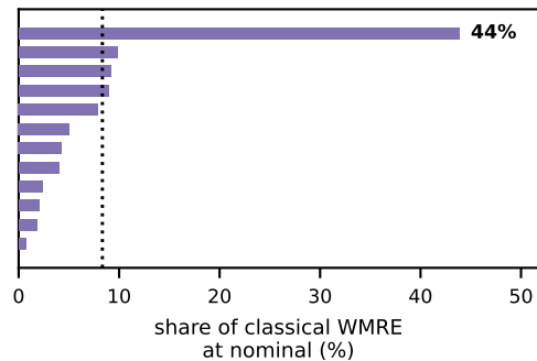
n-heptane
