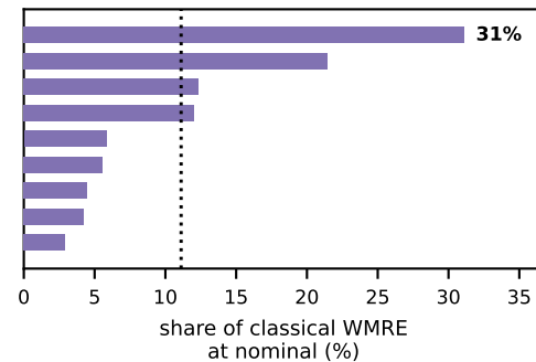
1,3-Butadiene
