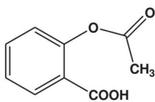
Aspirin (prodrug)
