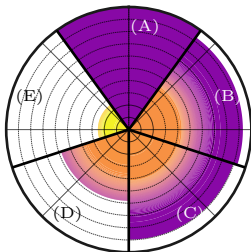
Helium
