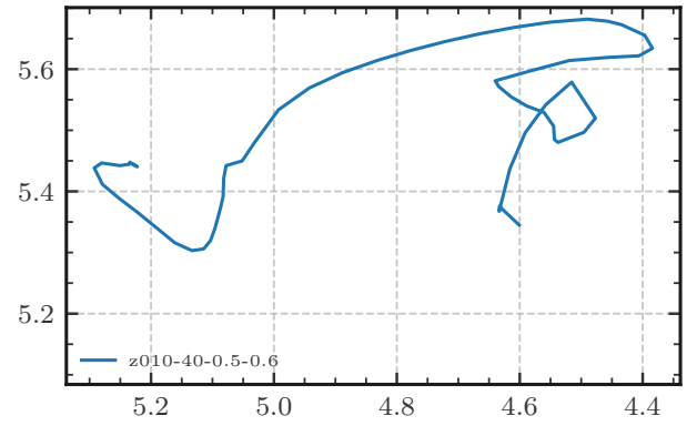
(f) VFTS 352
