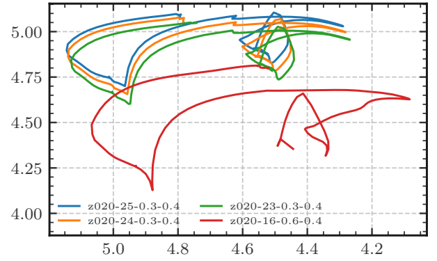
(d) TU Muscae
