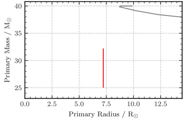
(f) VFTS 352
