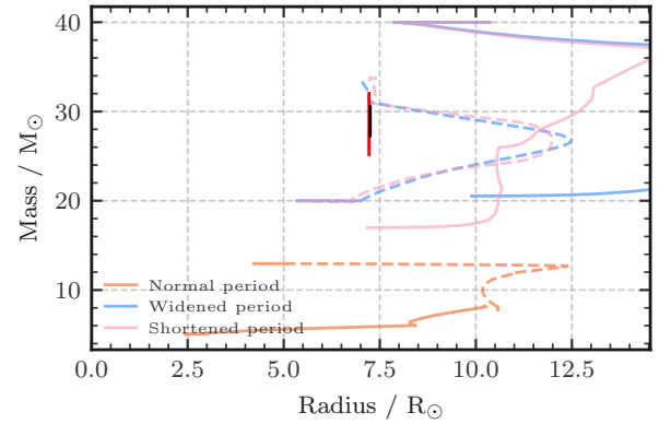
(f) VFTS 352
