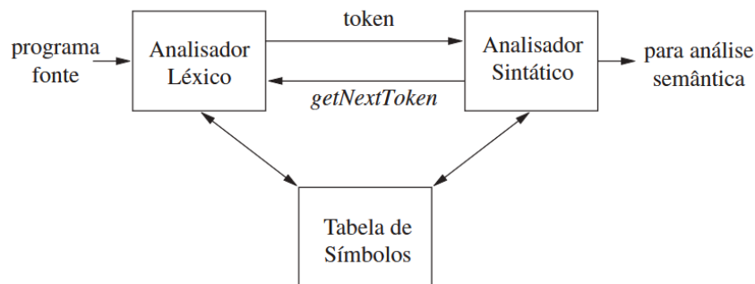
FIGURA 6 – INTERAÇÕES ENTRE O ANALISADOR LÉXICO E O ANALISADOR SINTÁTICO
