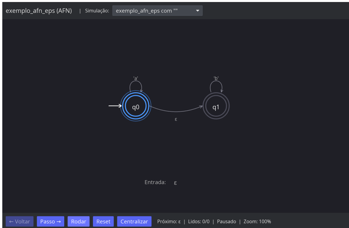
FIGURA 10 – INTERFACE DA FERRAMENTA AUTOSIM RENDERIZANDO O AFN- \varepsilon DA LISTAGEM 6.2
