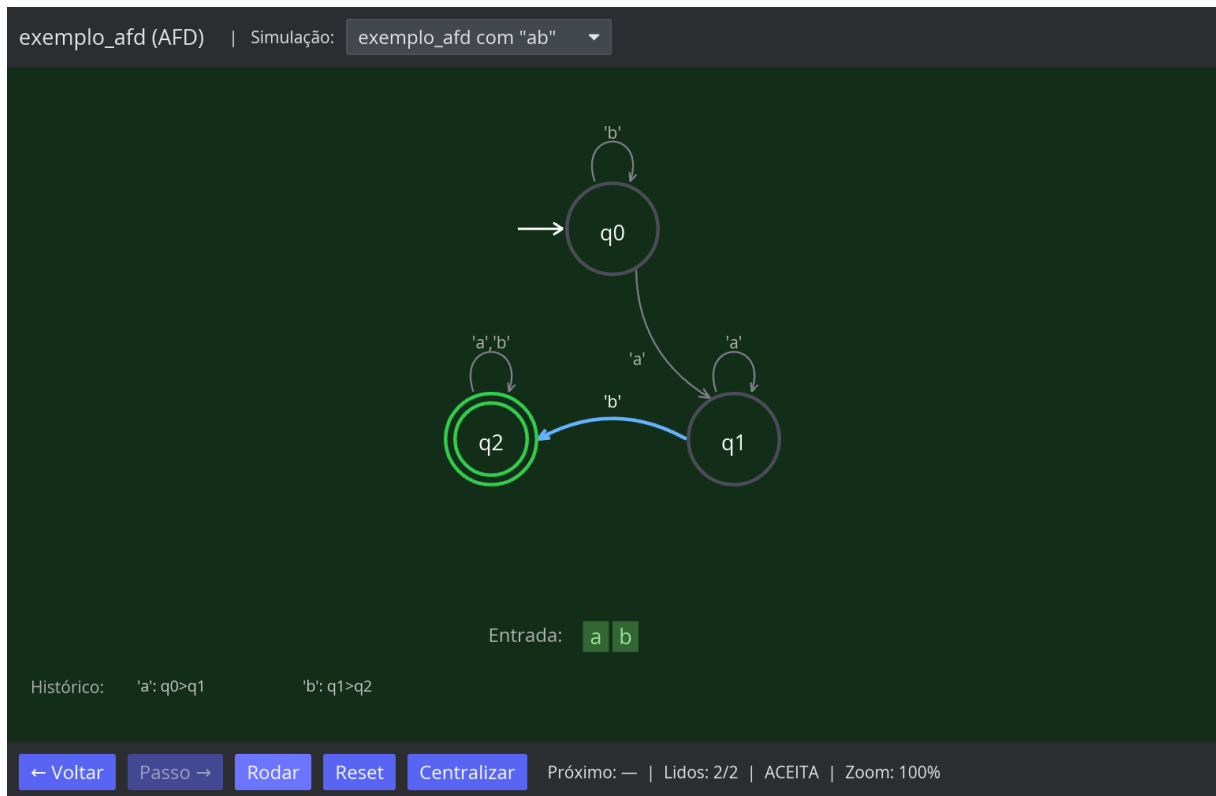
FIGURA 14 – SIMULAÇÃO CONCLUÍDA COM VEREDITO DE ACEITAÇÃO
