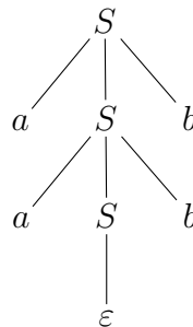
FIGURA 1 – ÁRVORE DE DERIVAÇÃO DA PALAVRA aabb NA GRAMÁTICA G
