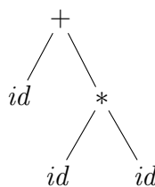
FIGURA 8 – ÁRVORE SINTÁTICA ABSTRATA DA EXPRESSÃO id + id * id
