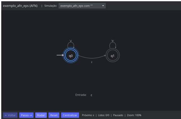
AFN com transições \epsilon
