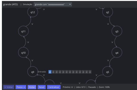
AFD de 14 estados — pan e zoom
