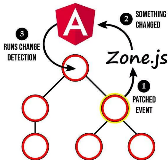
Rysunek 1.10: Tradycyjny model detekcji zmian w Angularze oparty na Zone.js (sprawdzanie od góry drzewa). [49]
