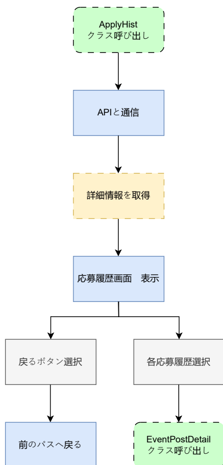
図 42: apply_hist.dart の状態遷移図
