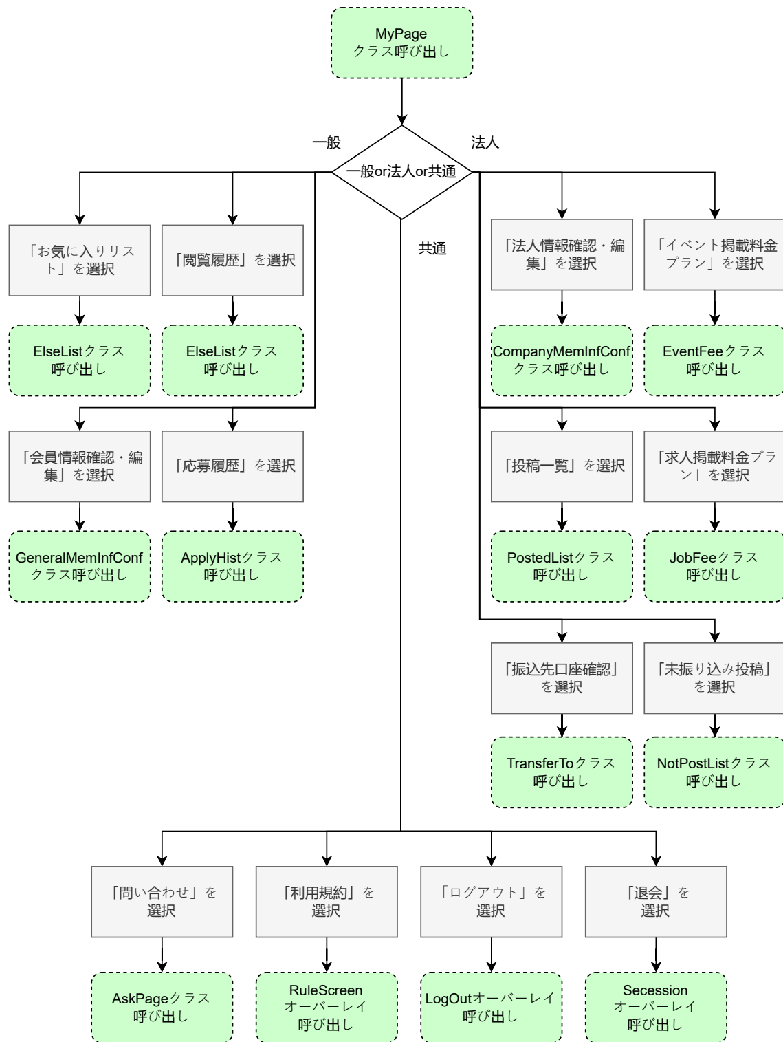
図 18: mypage.dart の状態遷移図
