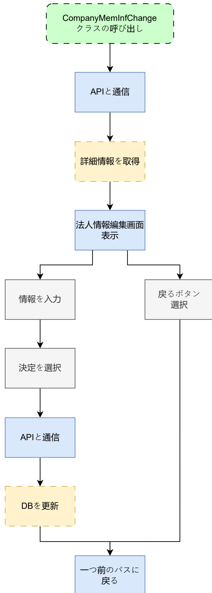
図 24: company_mem_inf_change.dart の状態遷移図
