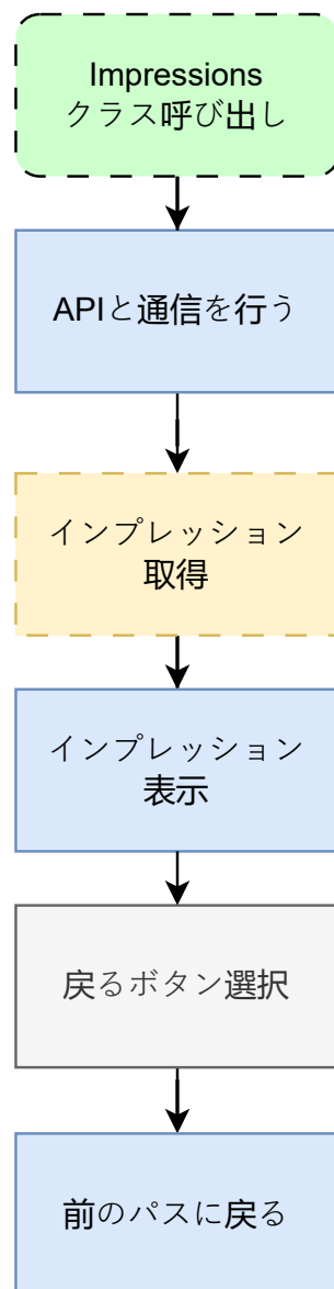
図 30: impressions.dart の状態遷移図
