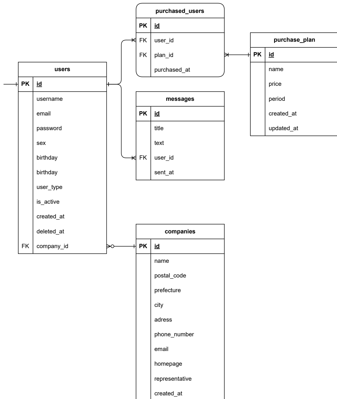
図 115: ER 図 (2)
