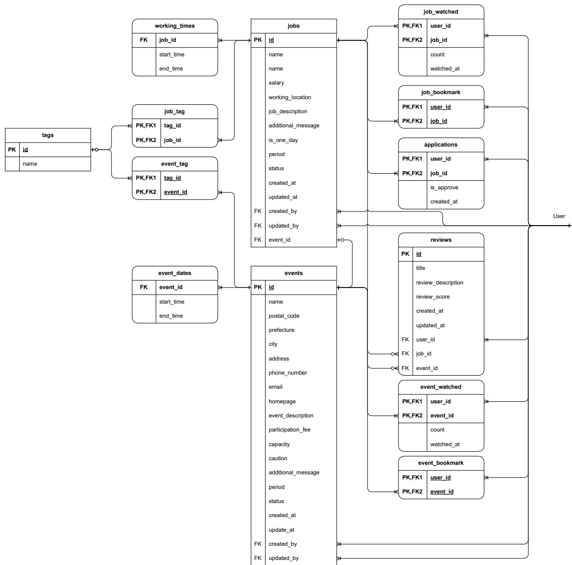
図 114: ER 図 (1)
