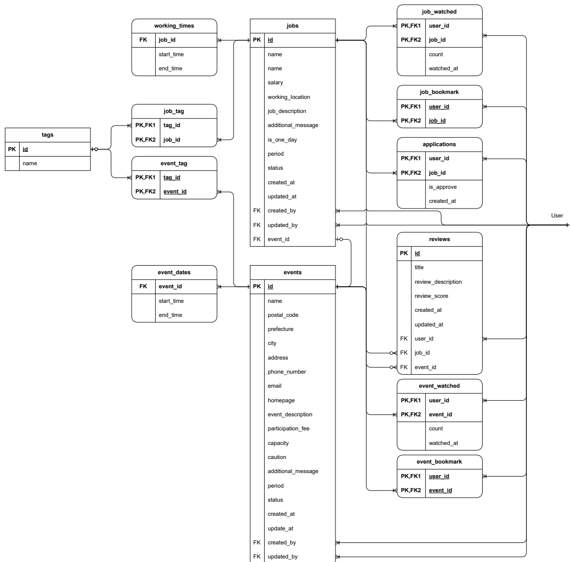
図 133: ER 図 (1)
