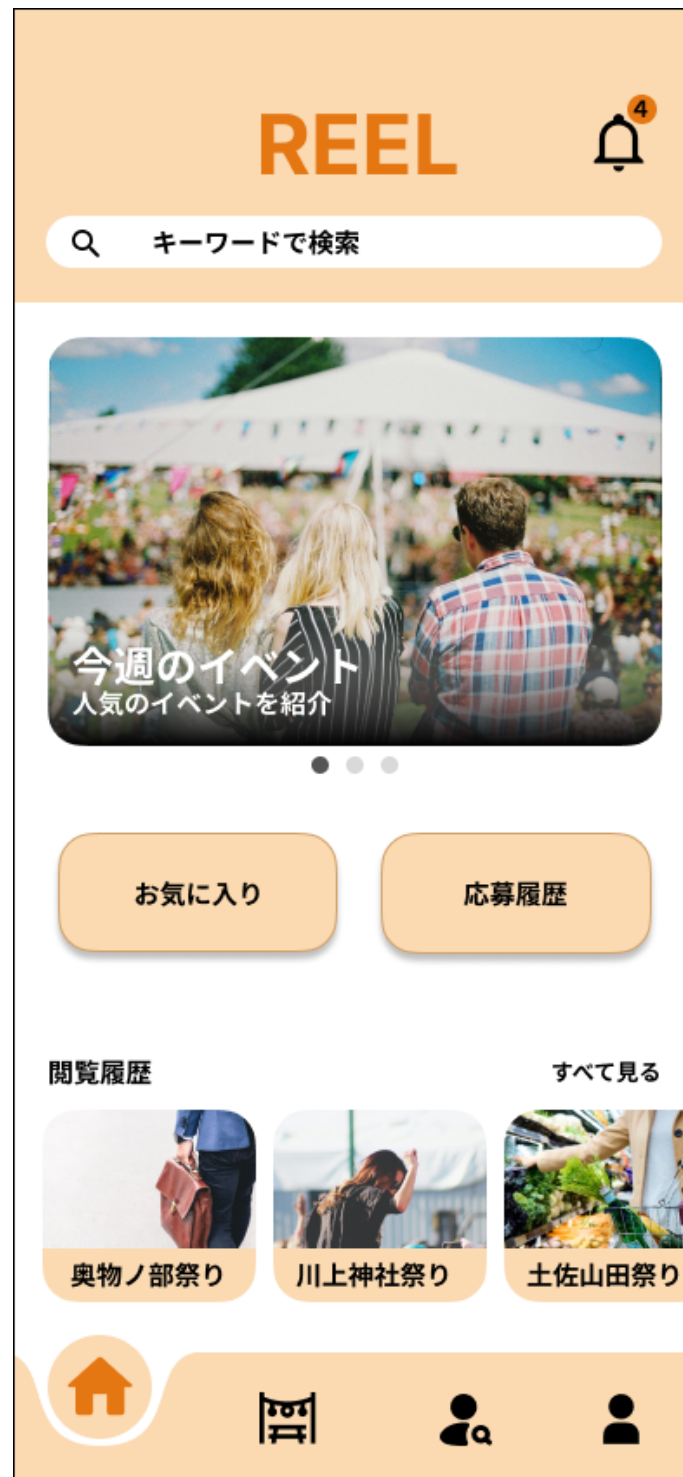
図 51: ホーム画面
