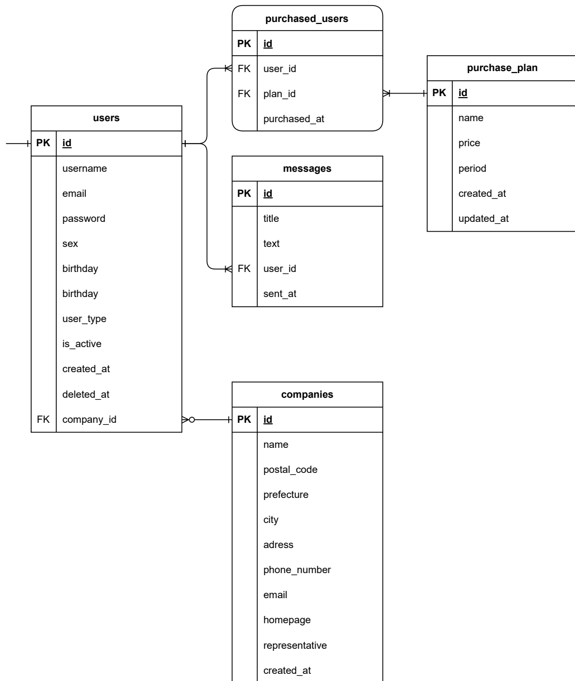
図 134: ER 図 (2)
