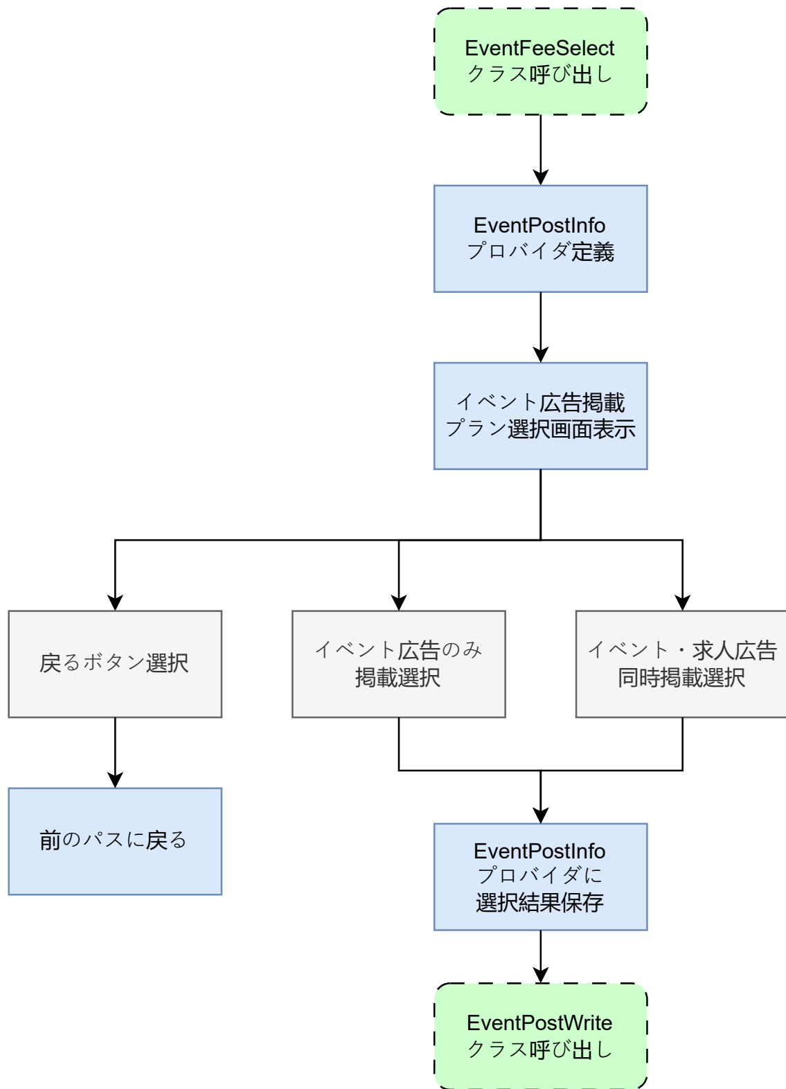
図 22: event_fee_select.dart の状態遷移図
