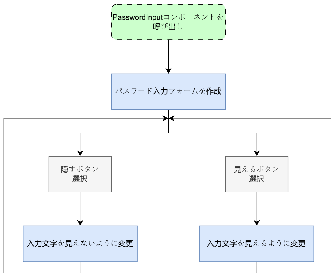
図 46: password_input.dart の状態遷移図
