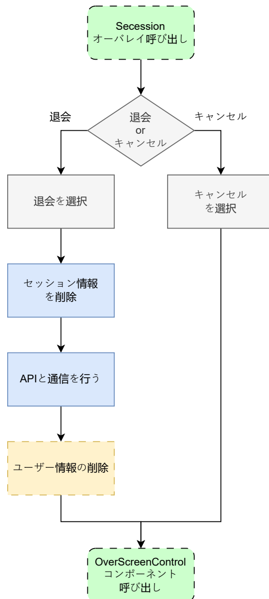
図 3: secession.dart の状態遷移図
