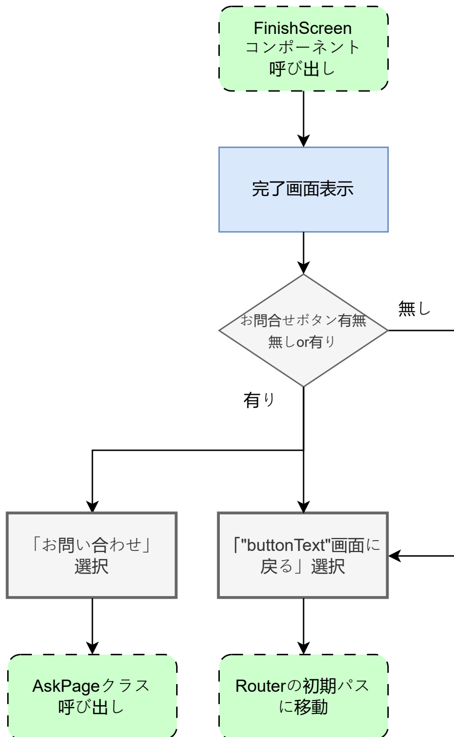
図 47: finish_screen.dart の状態遷移図
