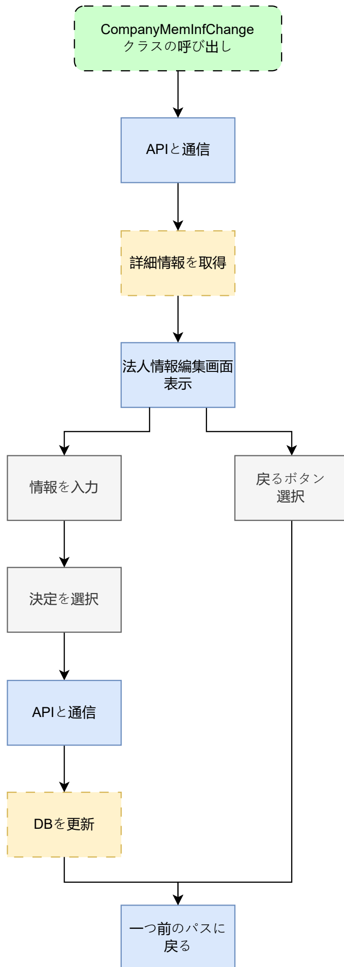
図 20: company_mem_inf_change.dart の状態遷移図
