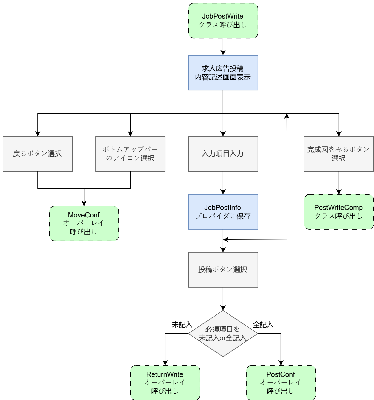
図 33: job_post_write.dart の状態遷移図
