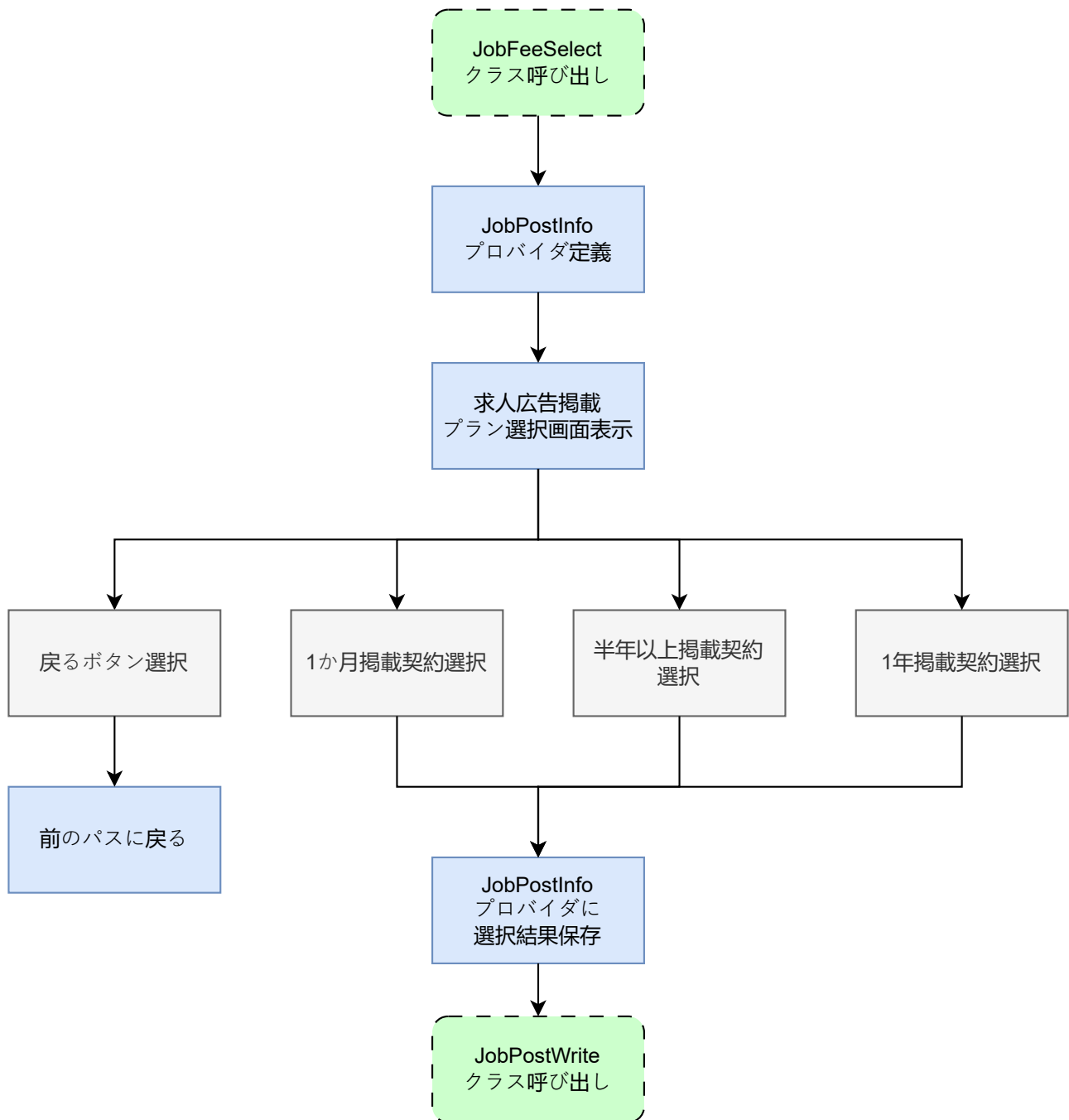
図 24: job_fee_select.dart の状態遷移図
