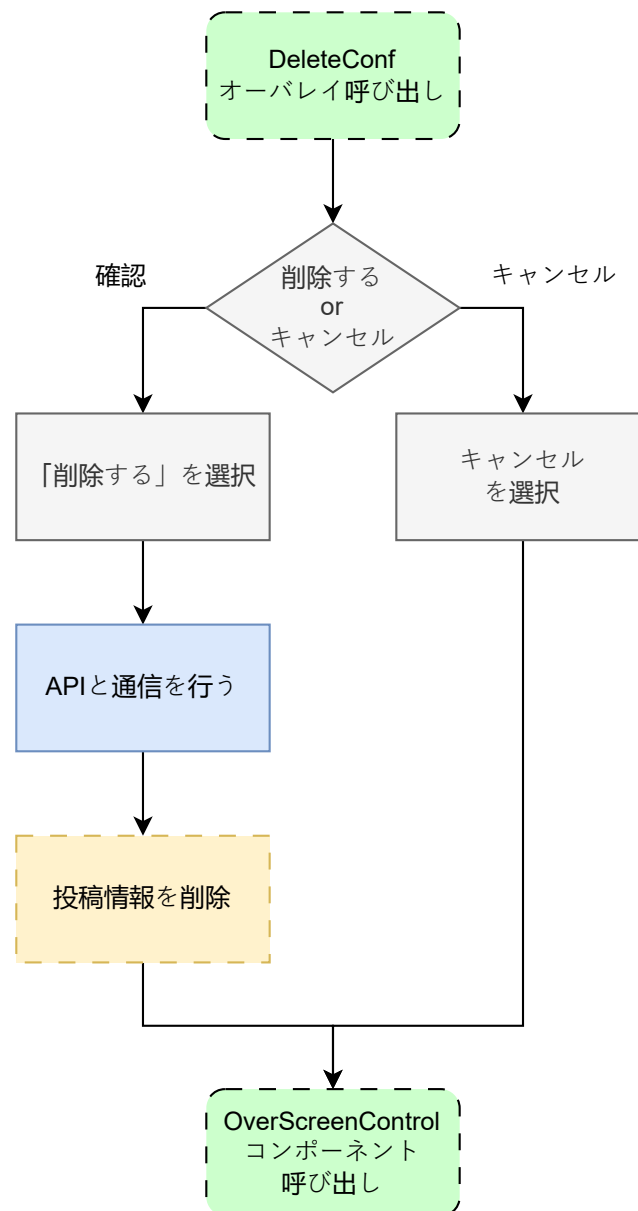
図 5: delete_conf.dart の状態遷移図
