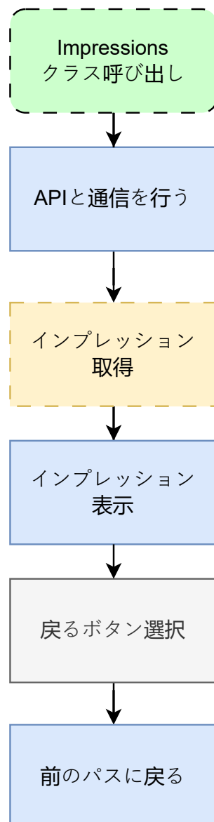
図 26: impressions.dart の状態遷移図
