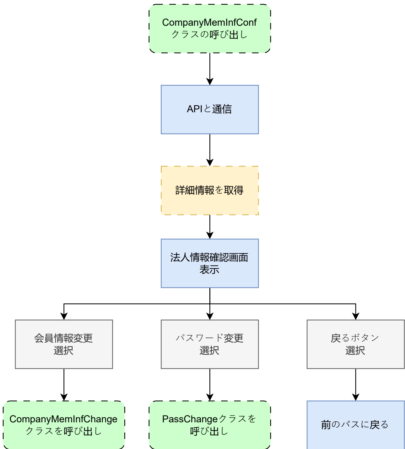
図 19: company_mem_inf_conf.dart の状態遷移図
