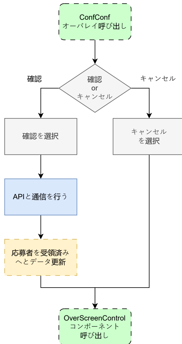
図 4: conf_conf.dart の状態遷移図
