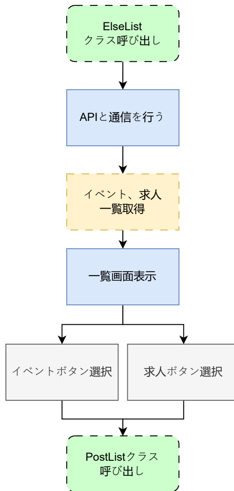
図 39: else_list.dart の状態遷移図
