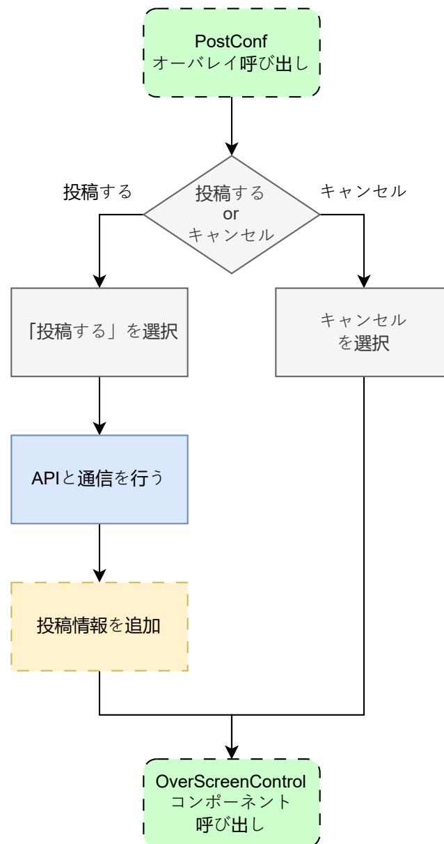
図 6: post_conf.dart の状態遷移図
