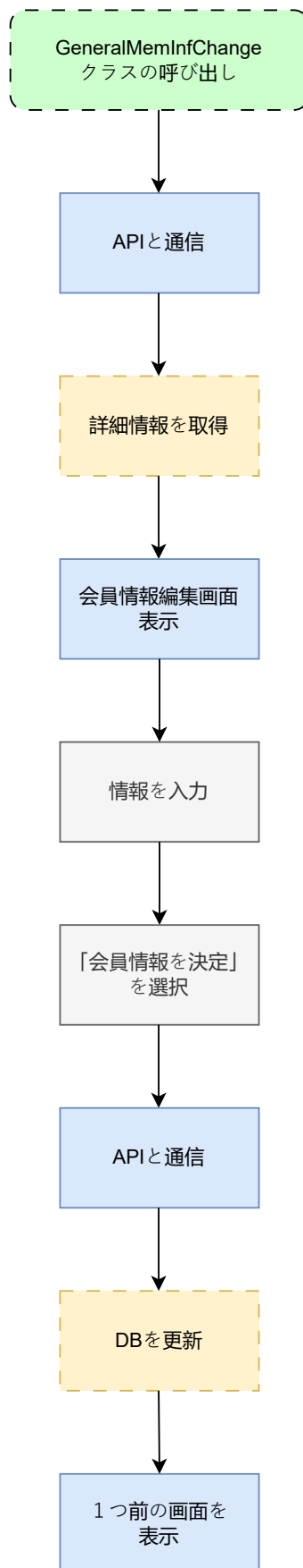
図 16: general_mem_inf.change.dart の状態遷移図
