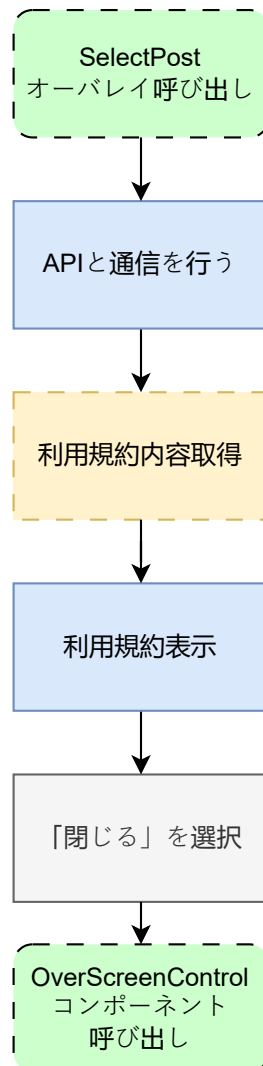
図 1: rule.screen.dart の状態遷移図
