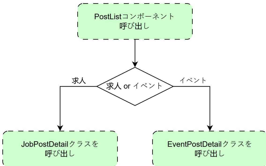
図 45: post_list.dart の状態遷移図
