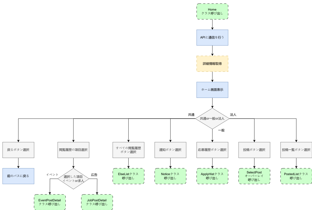
図 35: home.dart の状態遷移図
