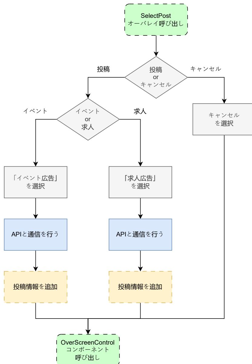
図 10: select_post.dart の状態遷移図
