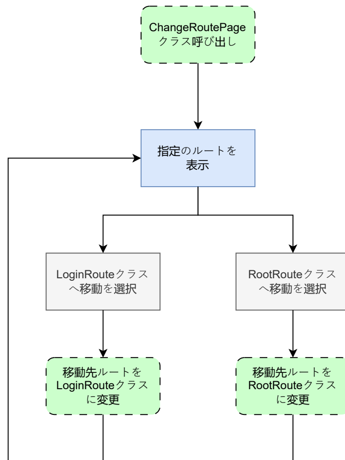
図 13: change_root_page.dart の状態遷移図
