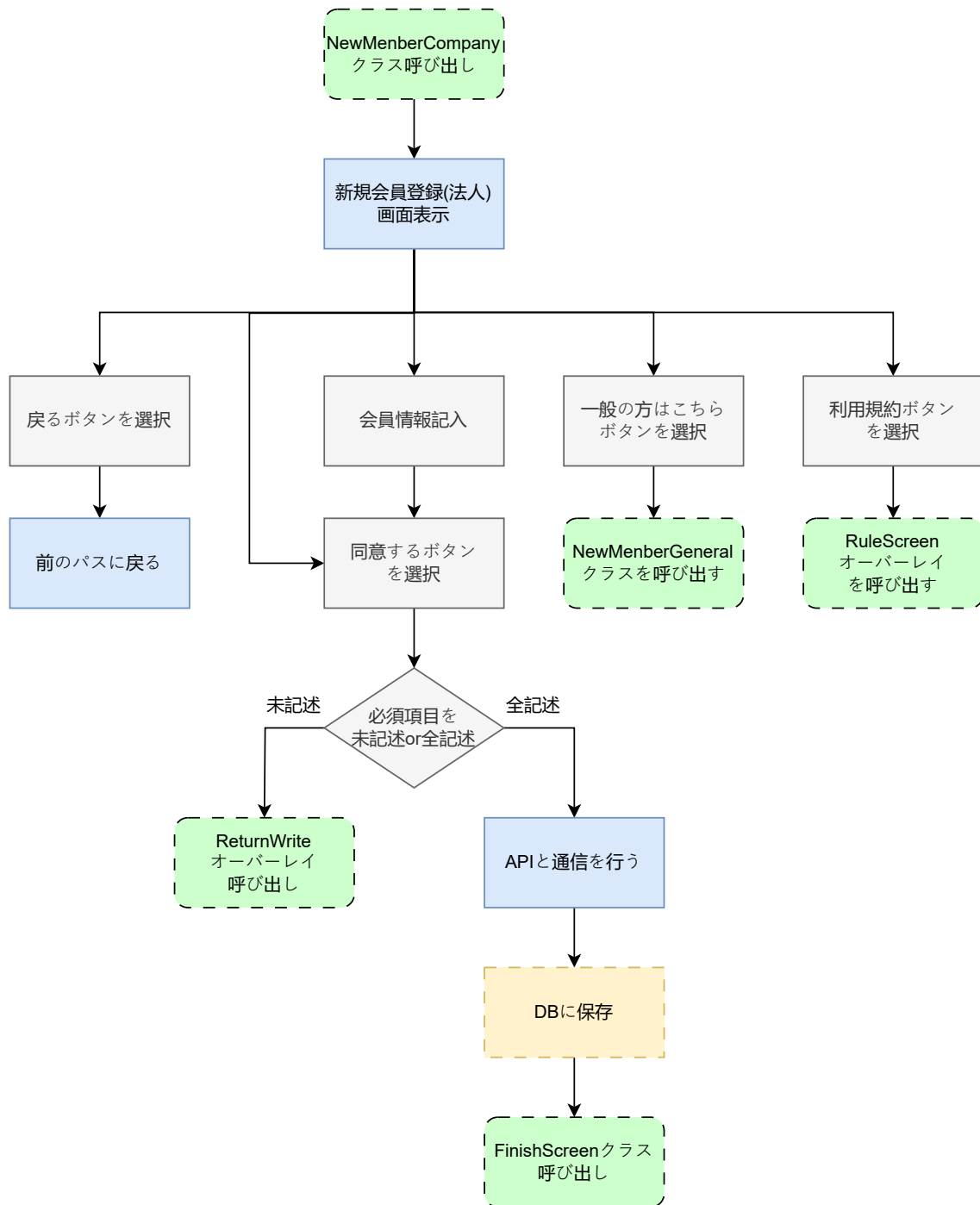
図 28: new_member_company.dart の状態遷移図
