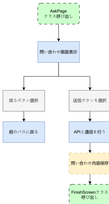
図 31: ask_page.dart の状態遷移図
