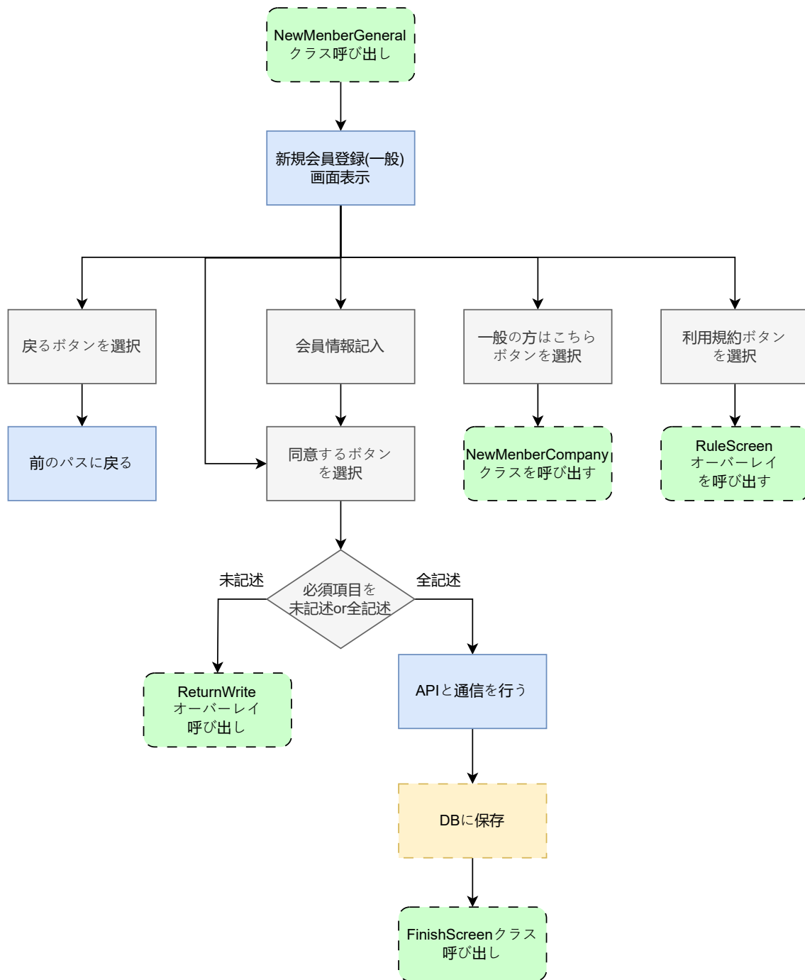
図 3: new_member_general.dart の状態遷移図
