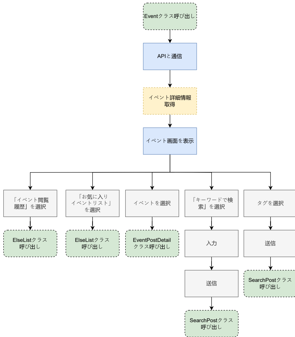
図 12: event.dart の状態遷移図
