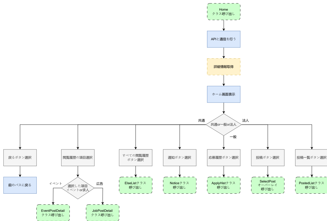
図 6: home.dart の状態遷移図
