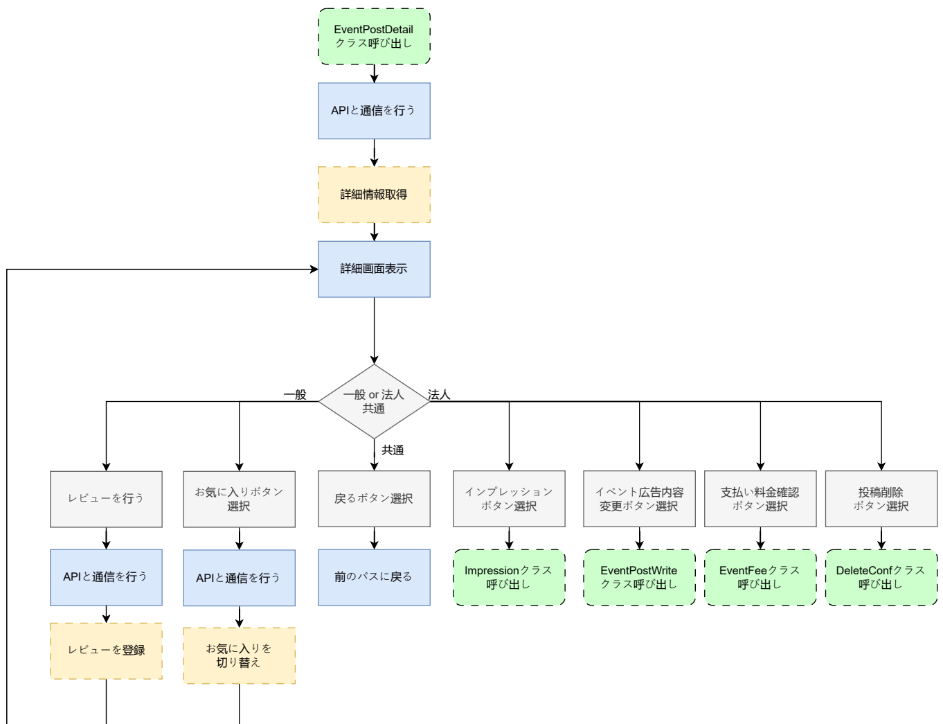
図 11: event_post_detail.dart の状態遷移図
