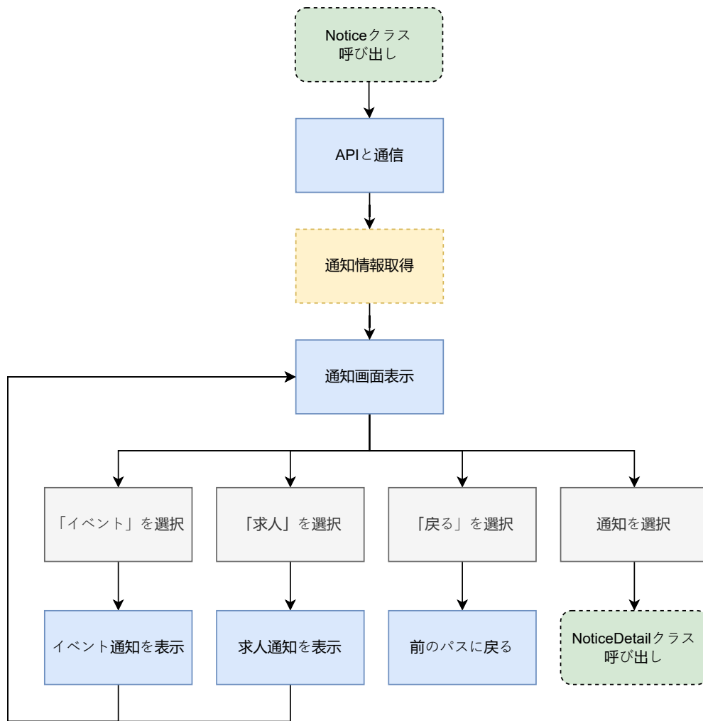
図 7: notice.dart の状態遷移図
