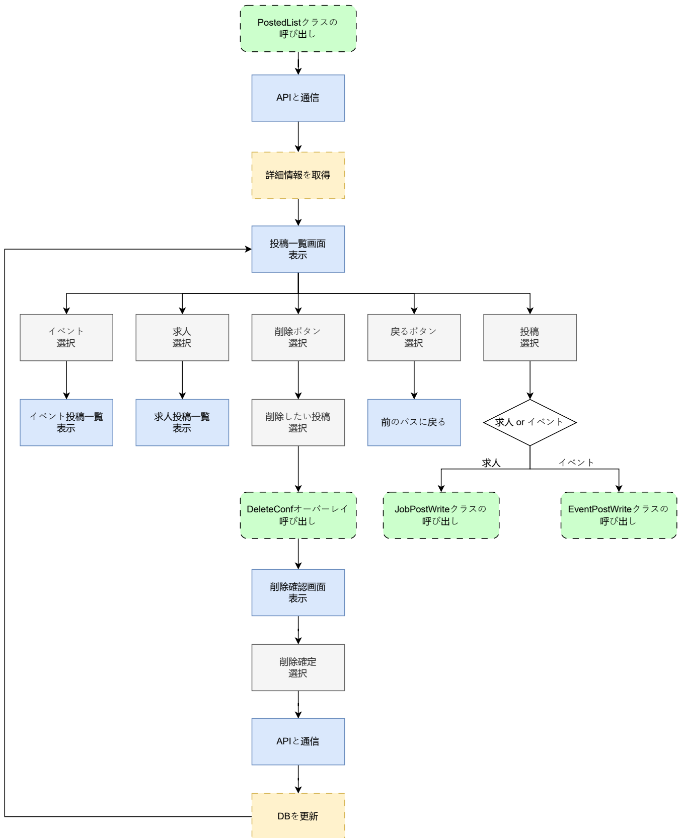
図 13: posted.list.dart の状態遷移図
