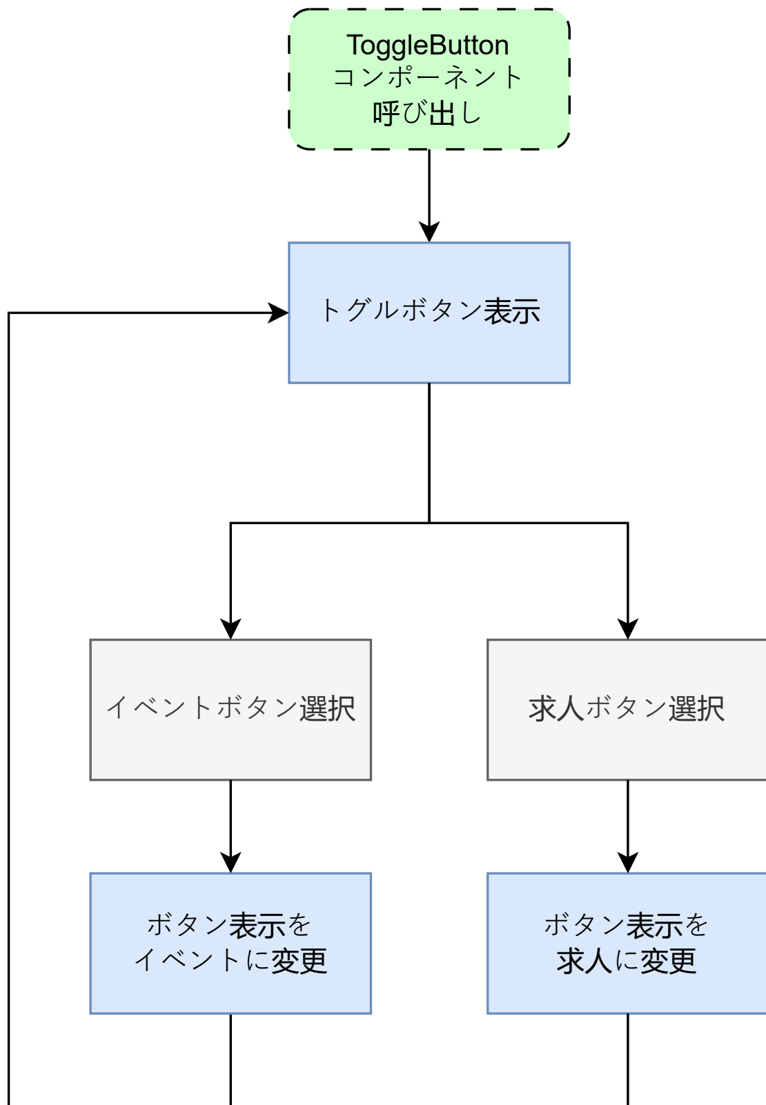
図 20: toggle_button.dart の状態遷移図
