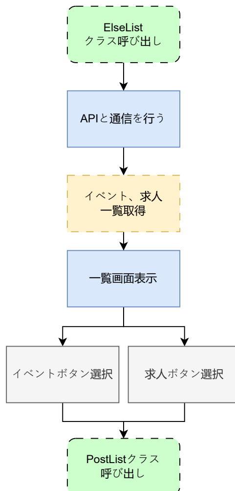
図 10: else_list.dart の状態遷移図
