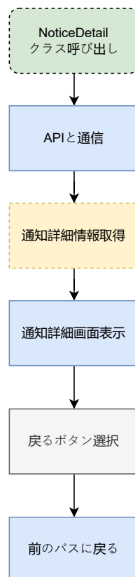
図 8: notice_detail.dart の状態遷移図
