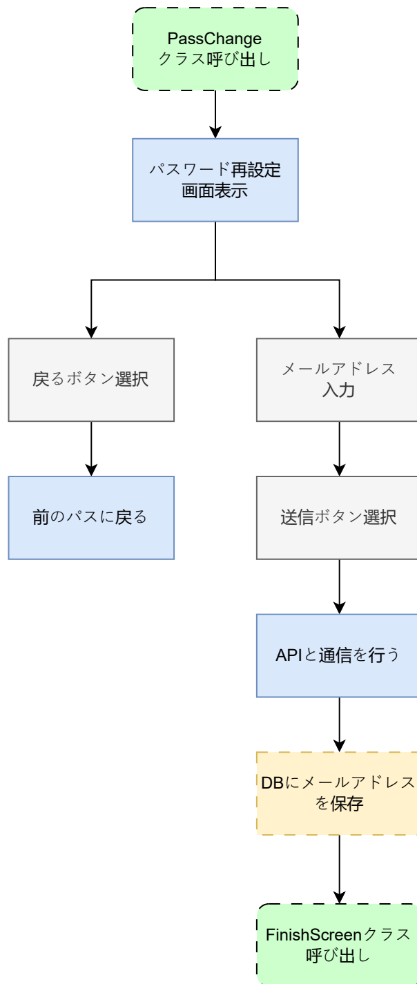
図 4: pass_change.dart の状態遷移図
