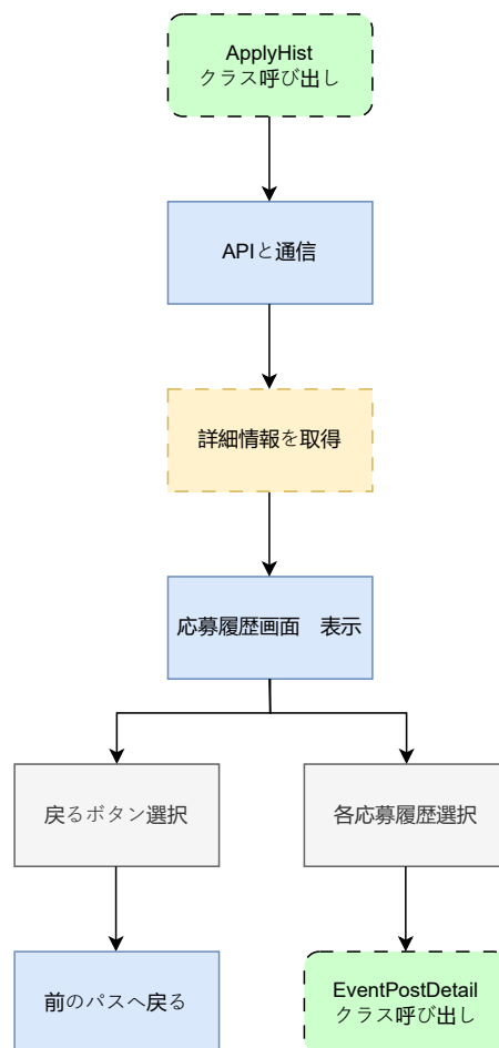
図 9: apply_hist.dart の状態遷移図
