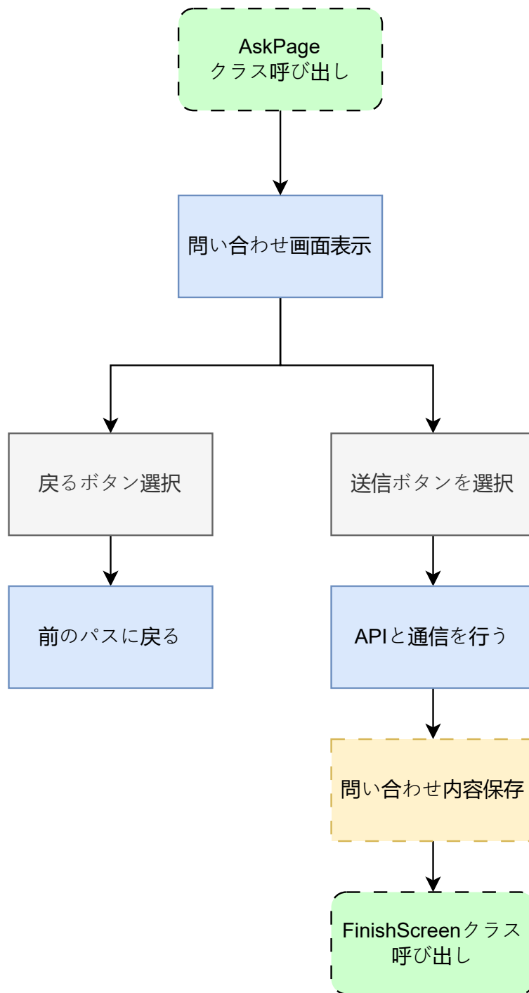
図 5: ask_page.dart の状態遷移図
