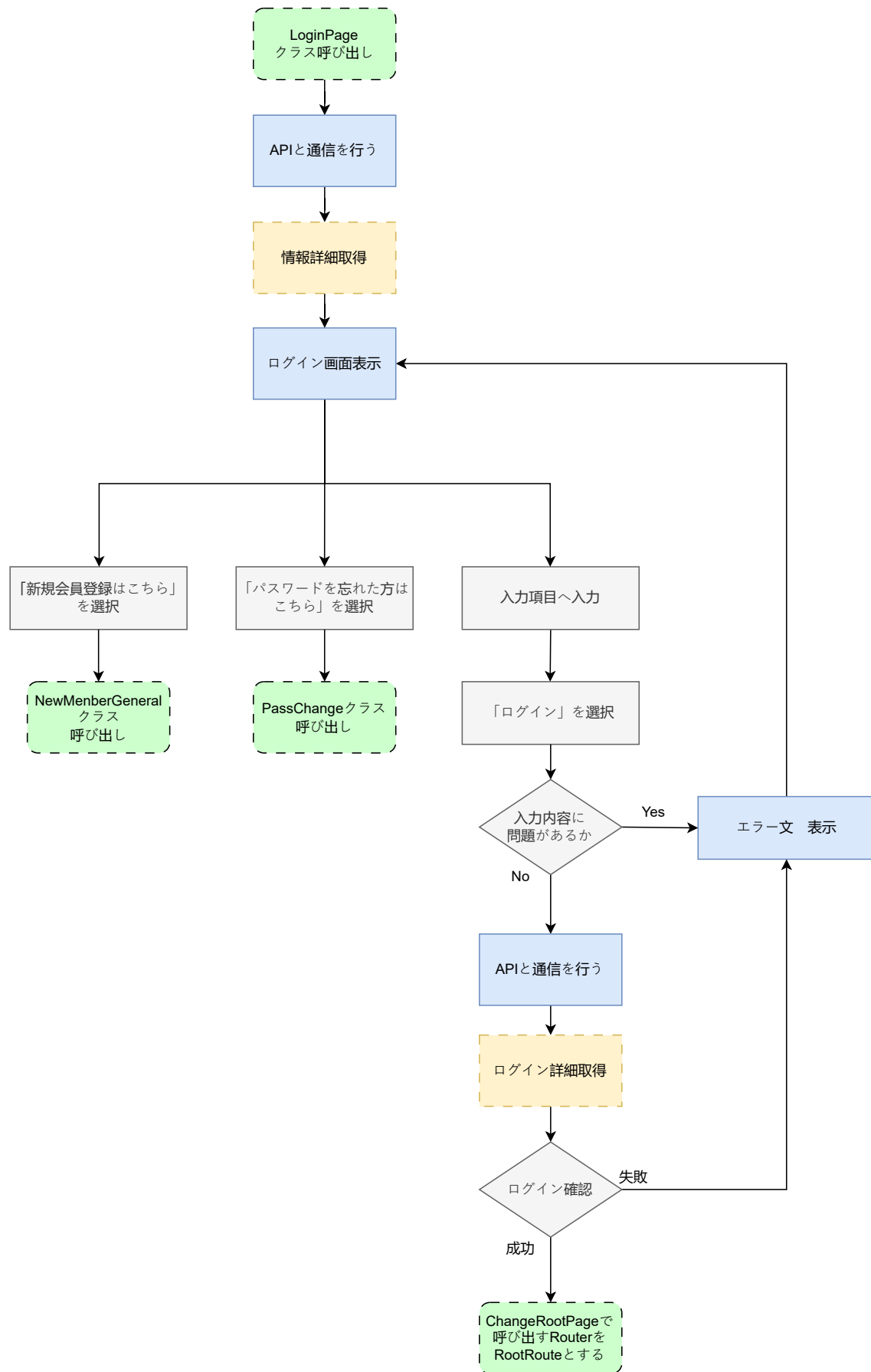
図 1: login_page.dart の状態遷移図
