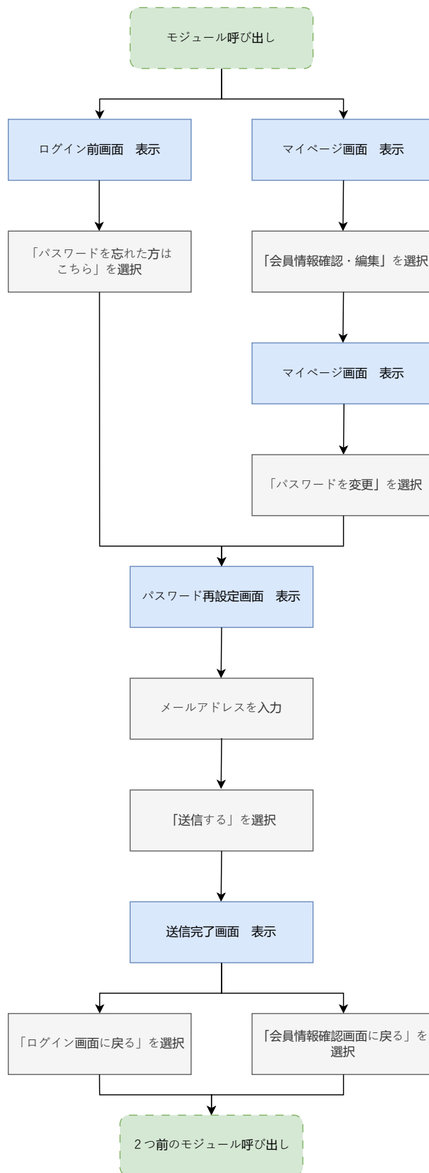
図 4: pass_change.dart の状態遷移図
