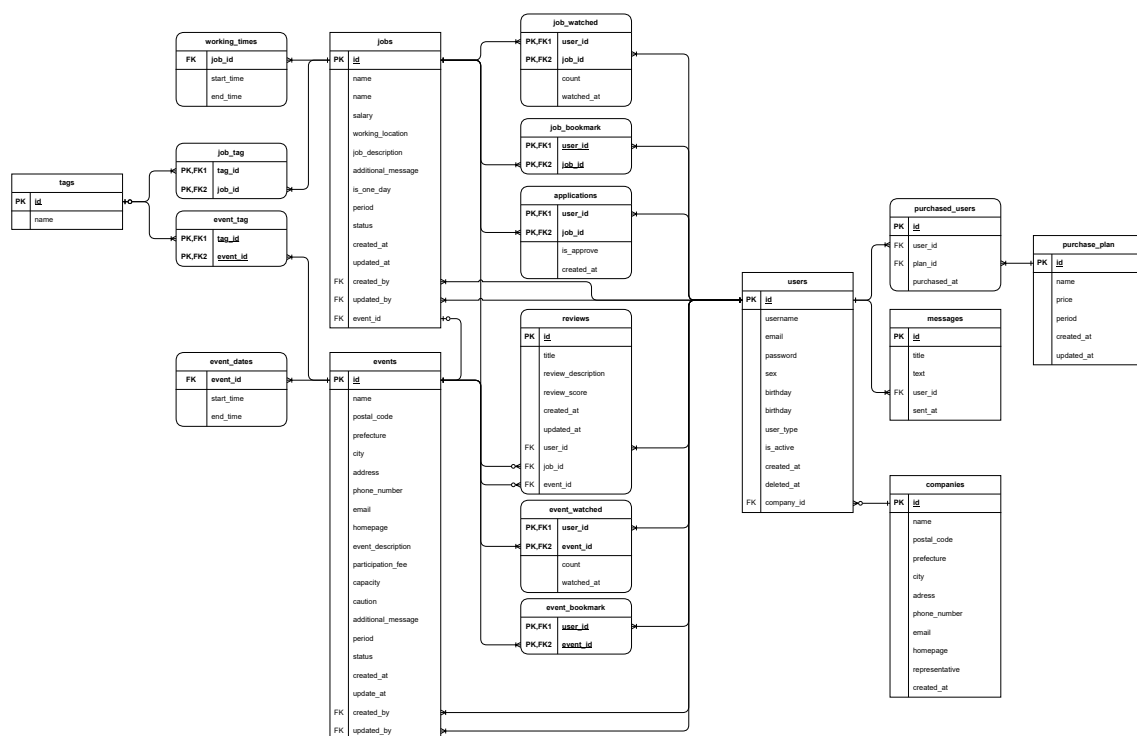
図 113: ER 図
