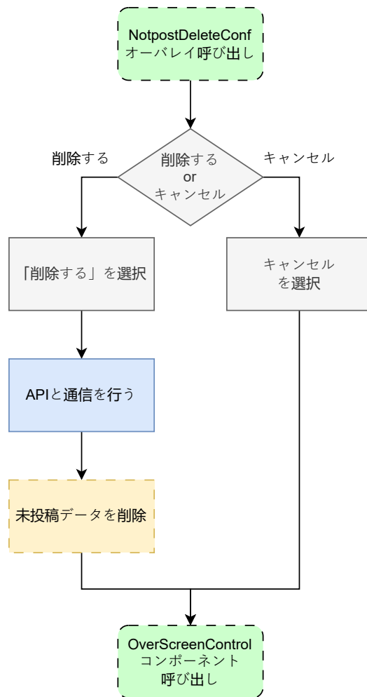
図 9: notpost_delete.conf.dart の状態遷移図
