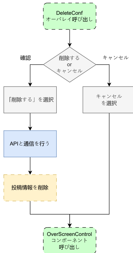
図 5: delete_conf.dart の状態遷移図
