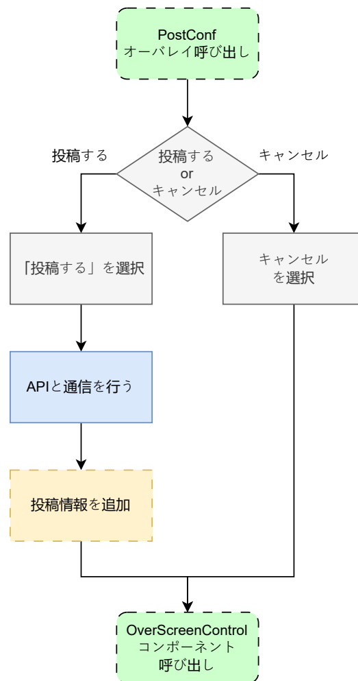
図 6: post_conf.dart の状態遷移図
