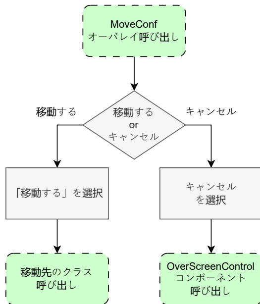
図 8: move_conf.dart の状態遷移図
