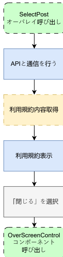
図 1: rule_screen.dart の状態遷移図
