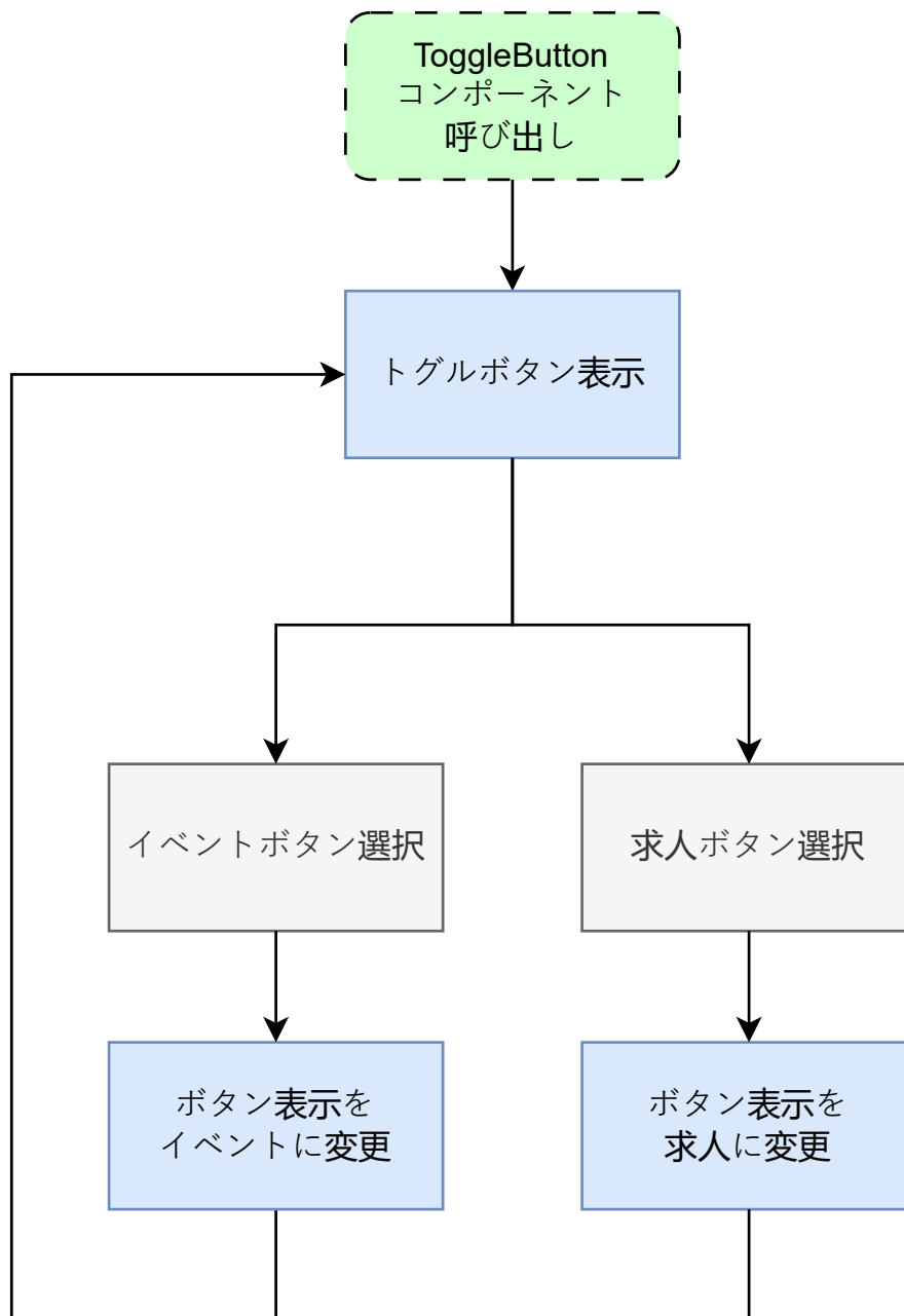
図 49: toggle.button.dart の状態遷移図
