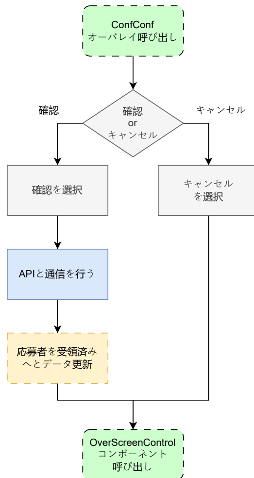
図 4: conf_conf.dart の状態遷移図
