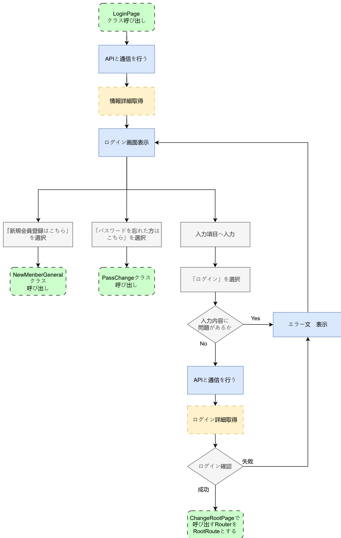
図 27: login_page.dart の状態遷移図
