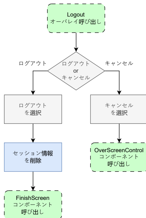
図 2: logout.dart の状態遷移図
