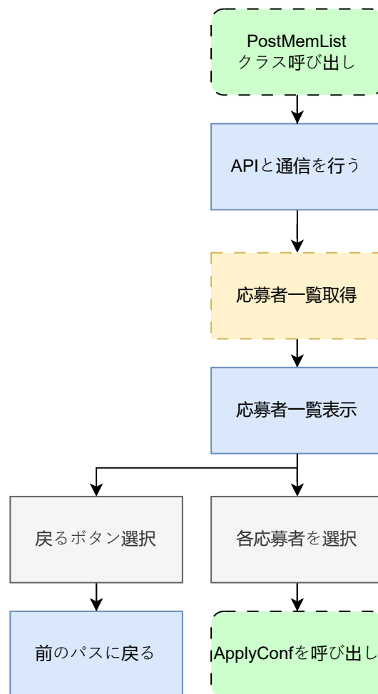
図 29: post_mem_list.dart の状態遷移図
