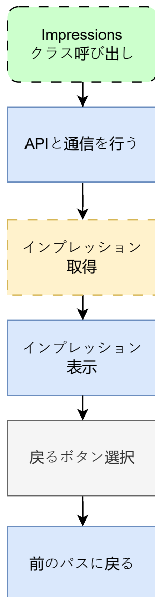
図 30: impressions.dart の状態遷移図
