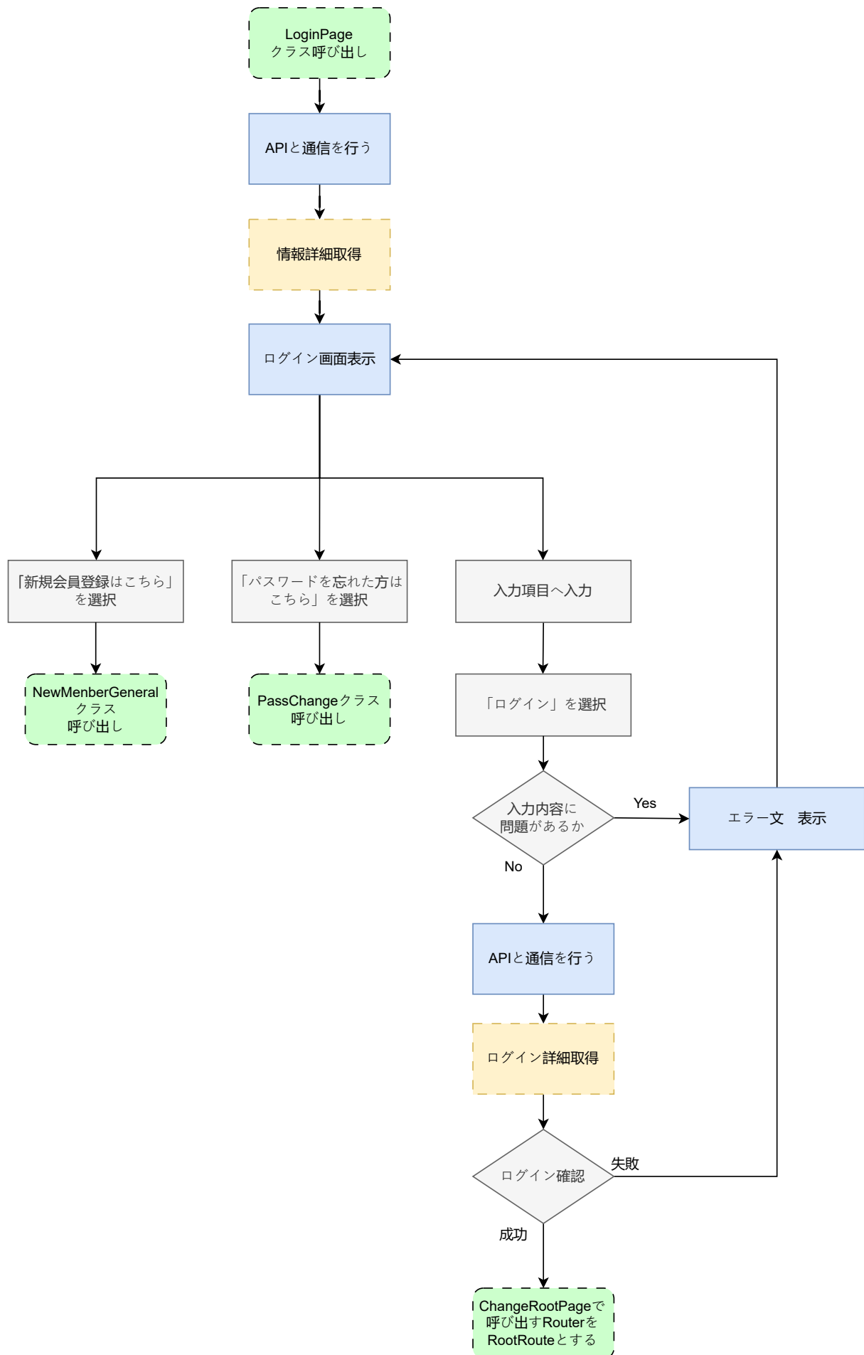
図 31: login_page.dart の状態遷移図
