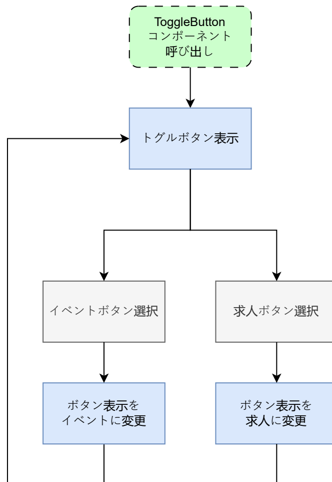
図 53: toggle_button.dart の状態遷移図
