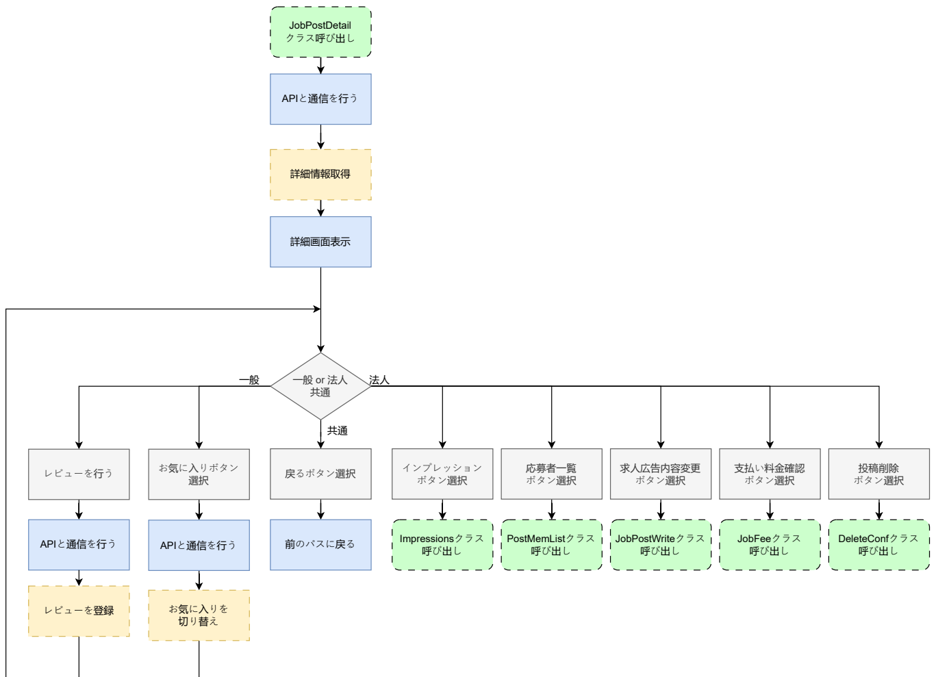
図 38: job_post_detail.dart の状態遷移図
