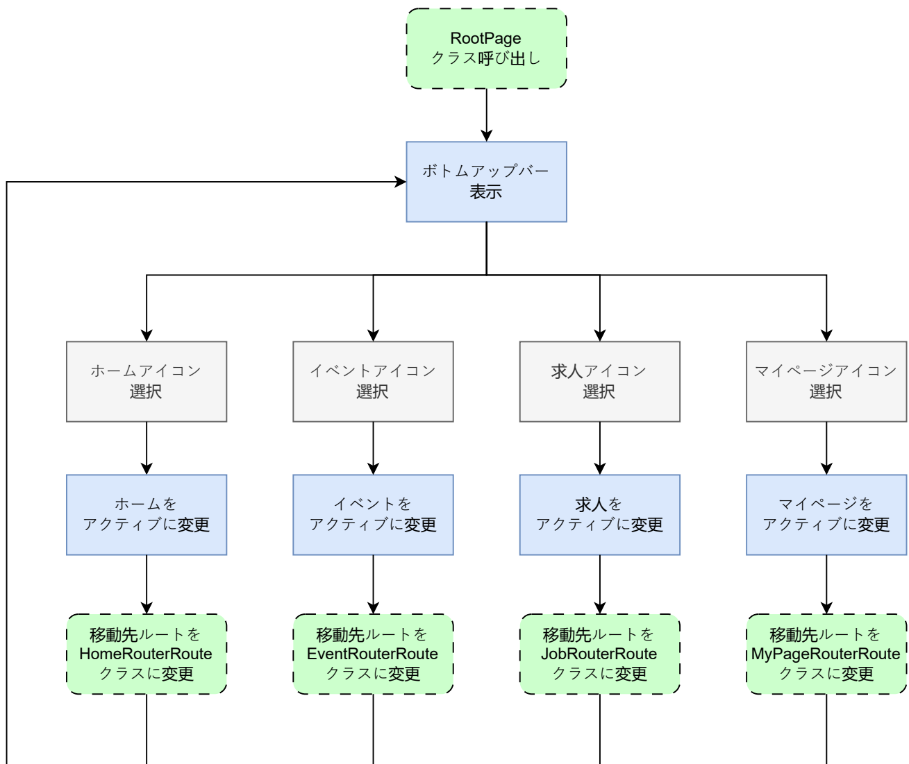
図 16: root_page.dart の状態遷移図
