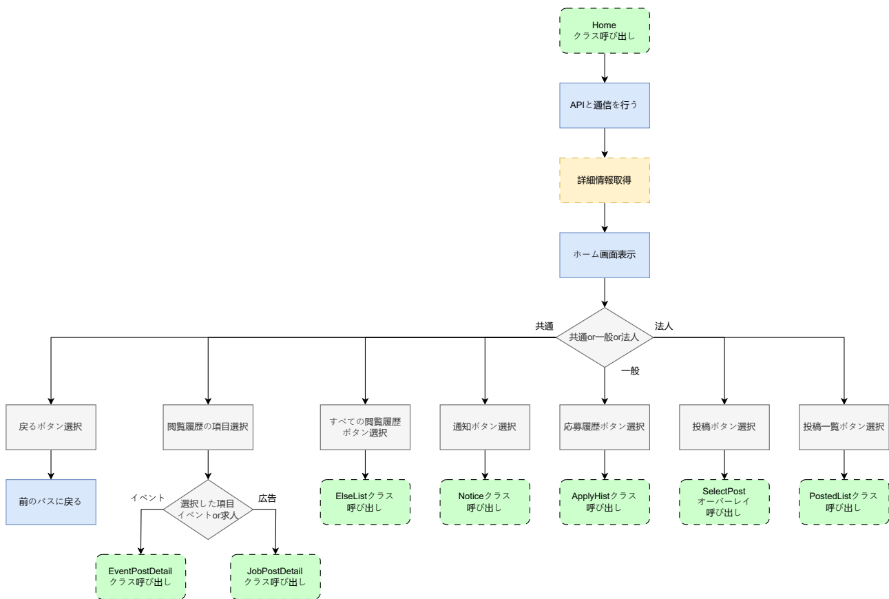
図 39: home.dart の状態遷移図
