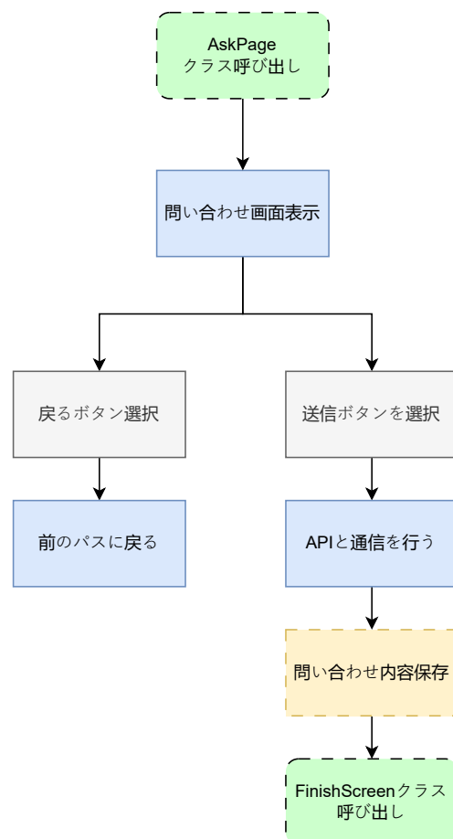
図 35: ask_page.dart の状態遷移図
