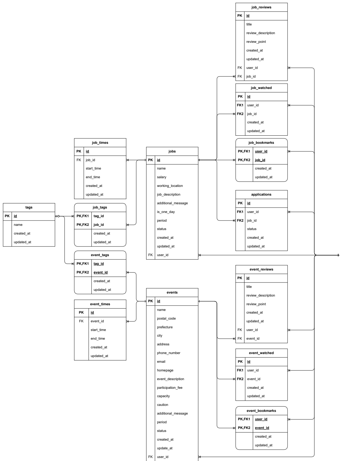
図 55: ER 図 (1)
