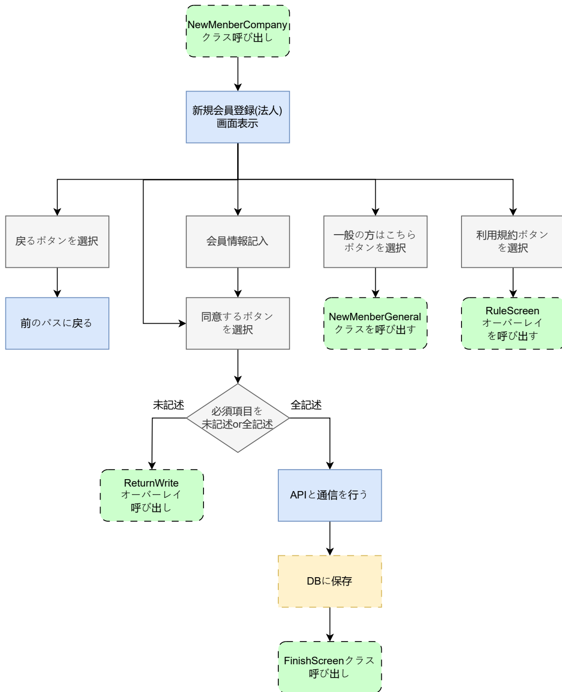
図 32: new_member_company.dart の状態遷移図
