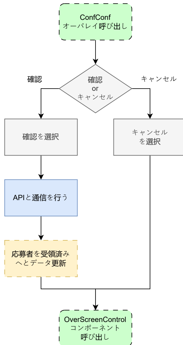
図 8: conf_conf.dart の状態遷移図
