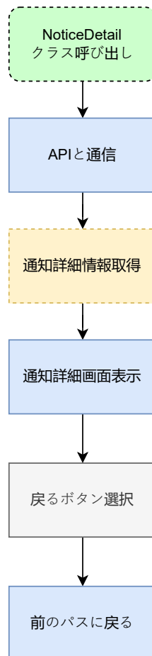
図 41: notice_detail.dart の状態遷移図
