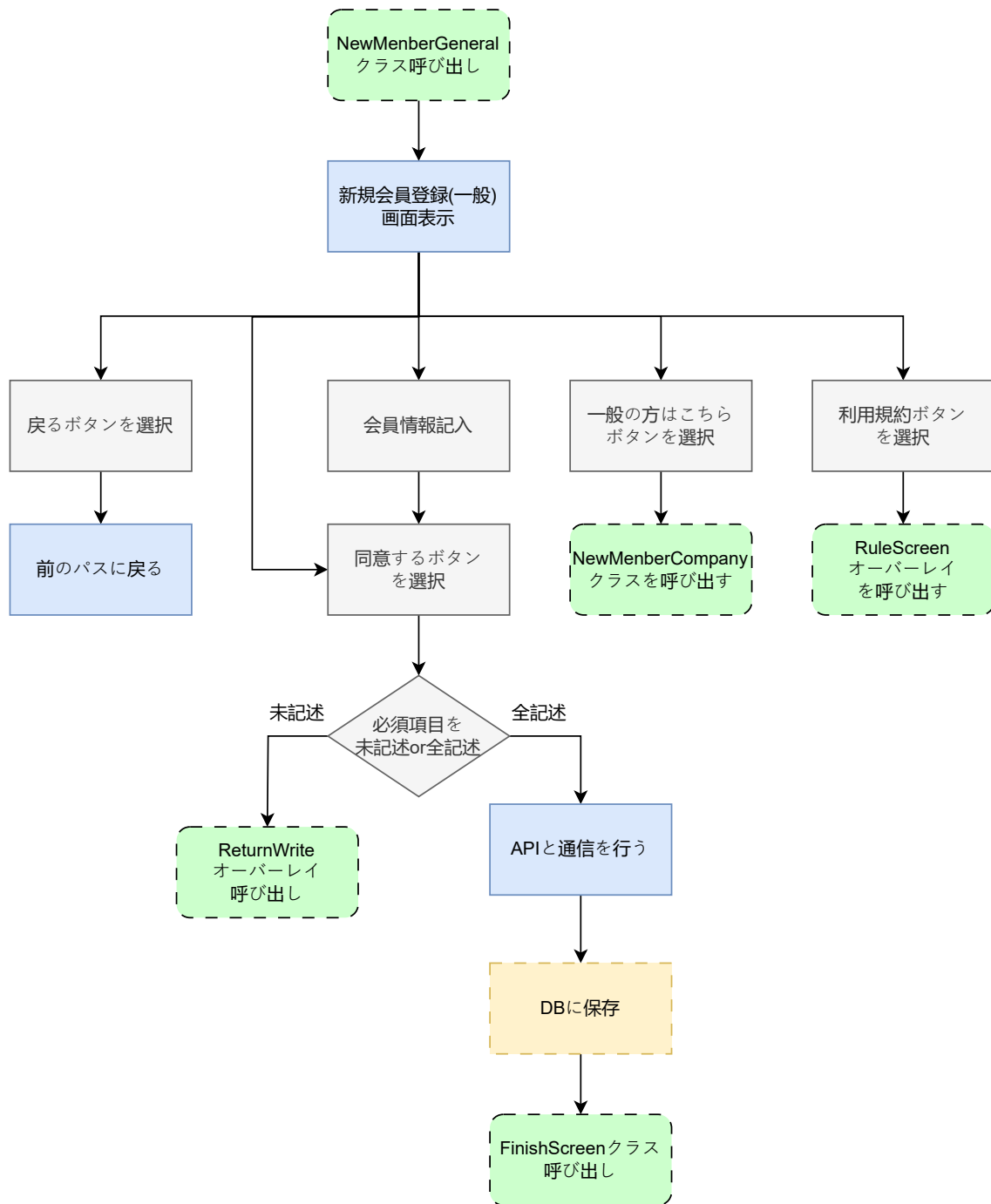
図 33: new_member_general.dart の状態遷移図
