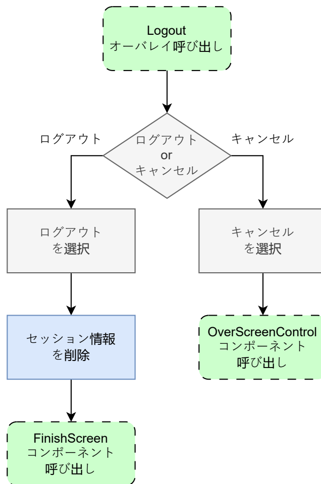
図 6: logout.dart の状態遷移図
