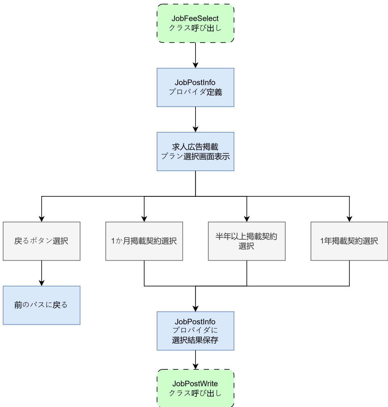
図 28: job_fee_select.dart の状態遷移図
