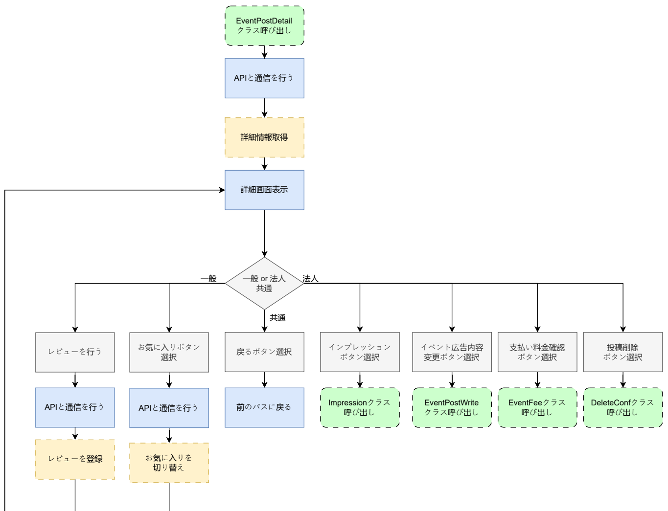
図 44: event_post_detail.dart の状態遷移図
