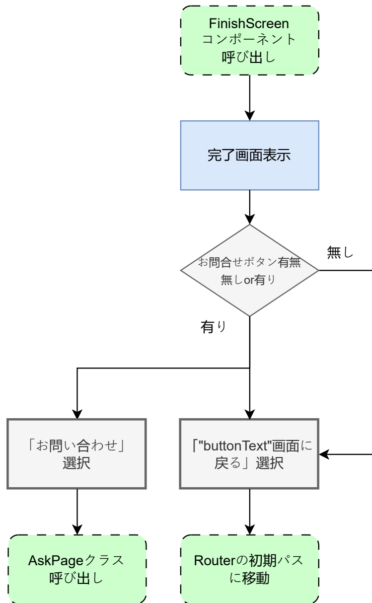
図 51: finish_screen.dart の状態遷移図
