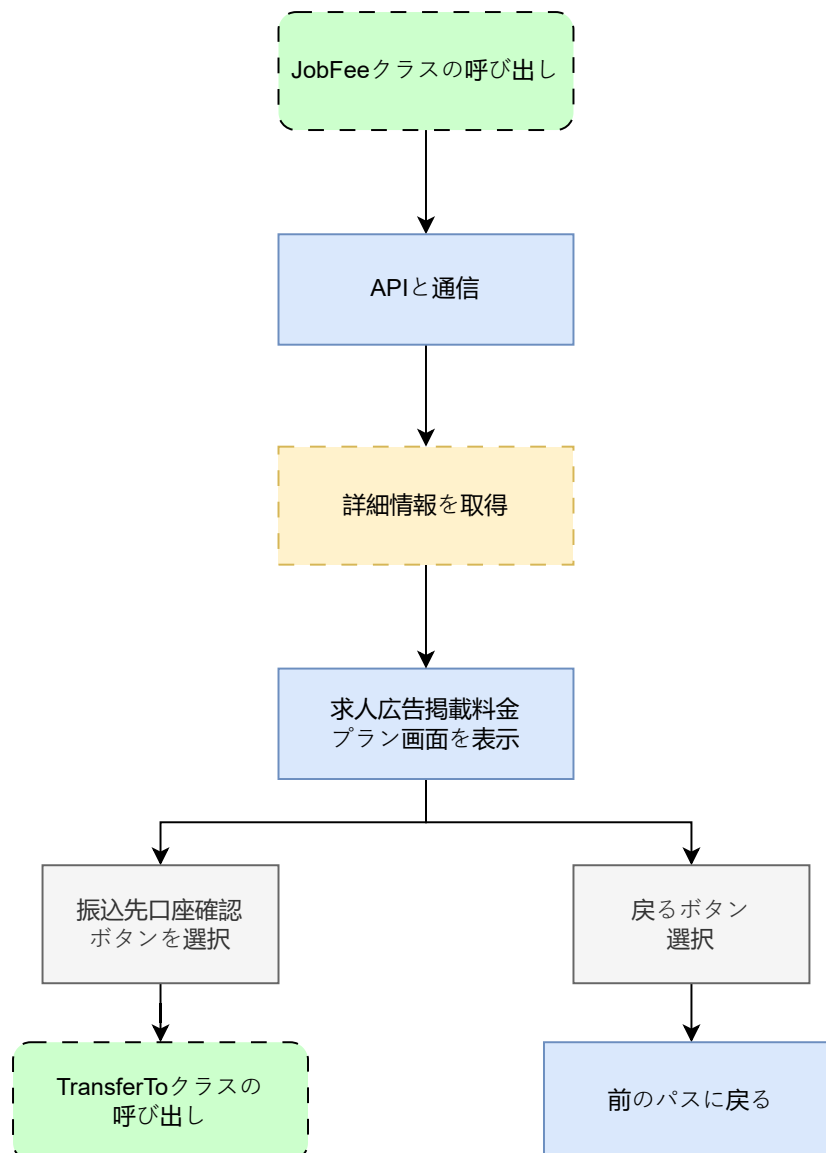
図 27: job_fee.dart の状態遷移図
