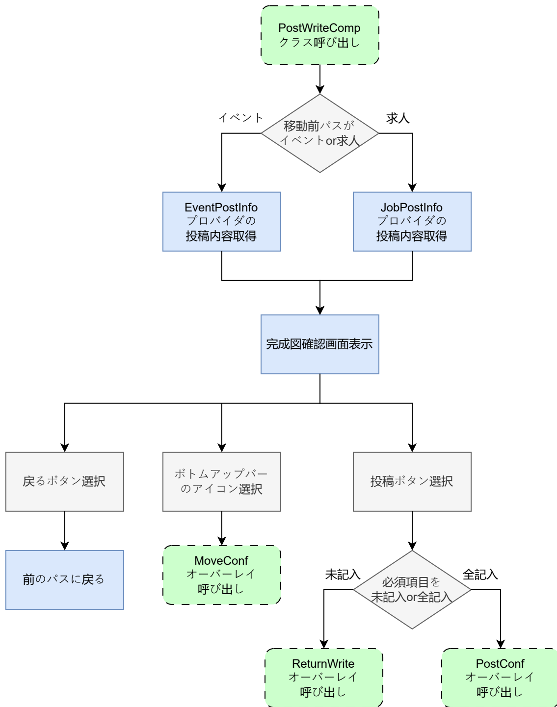
図 48: post_write_comp.dart の状態遷移図
