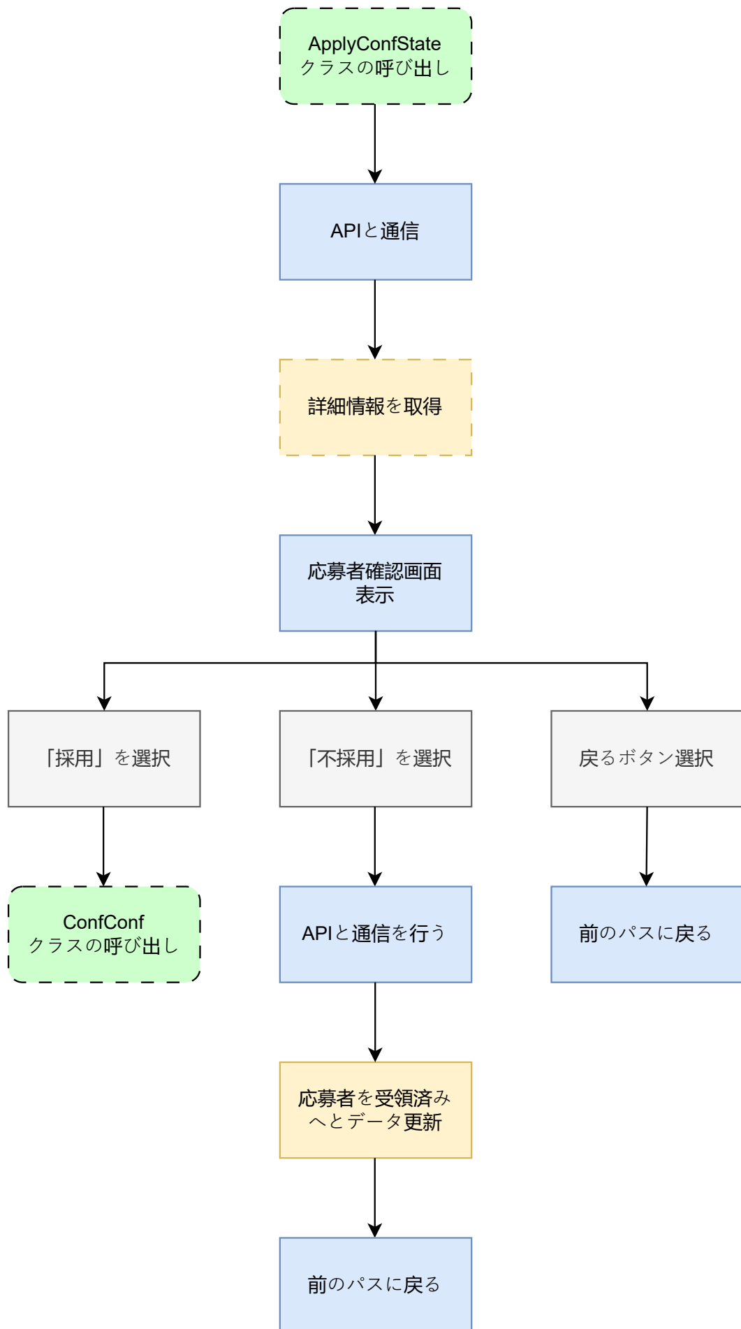
図 21: apply_conf.dart の状態遷移図
