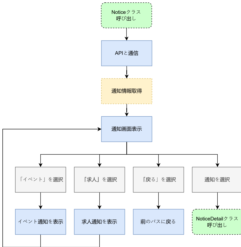
図 40: notice.dart の状態遷移図
