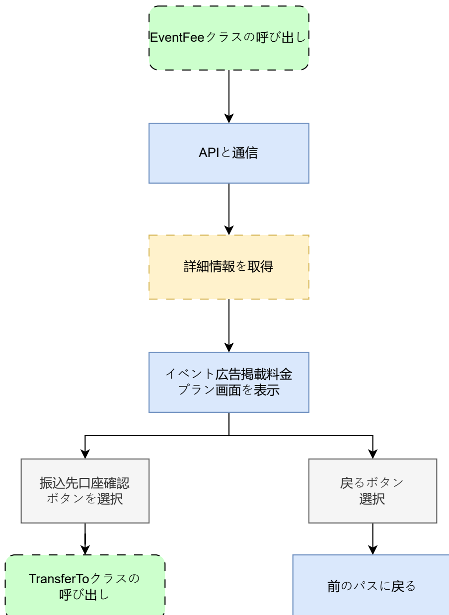
図 25: event_fee.dart の状態遷移図
