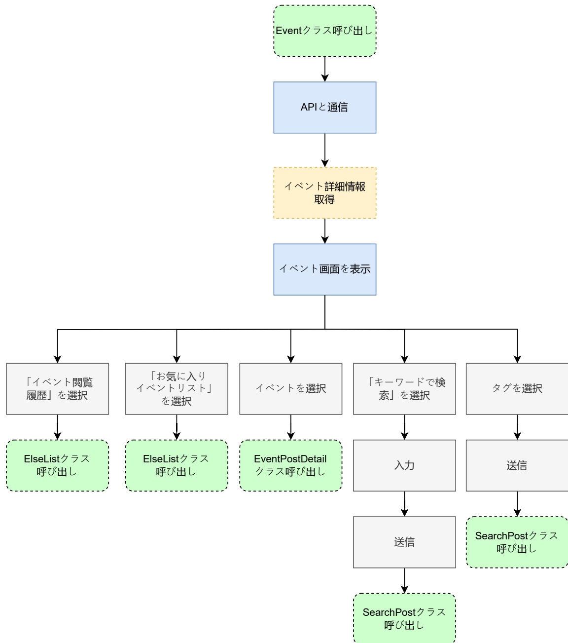
図 45: event.dart の状態遷移図
