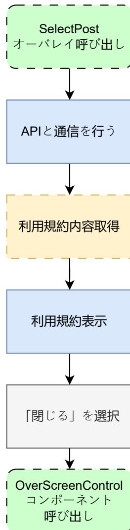
図 5: rule_screen.dart の状態遷移図
