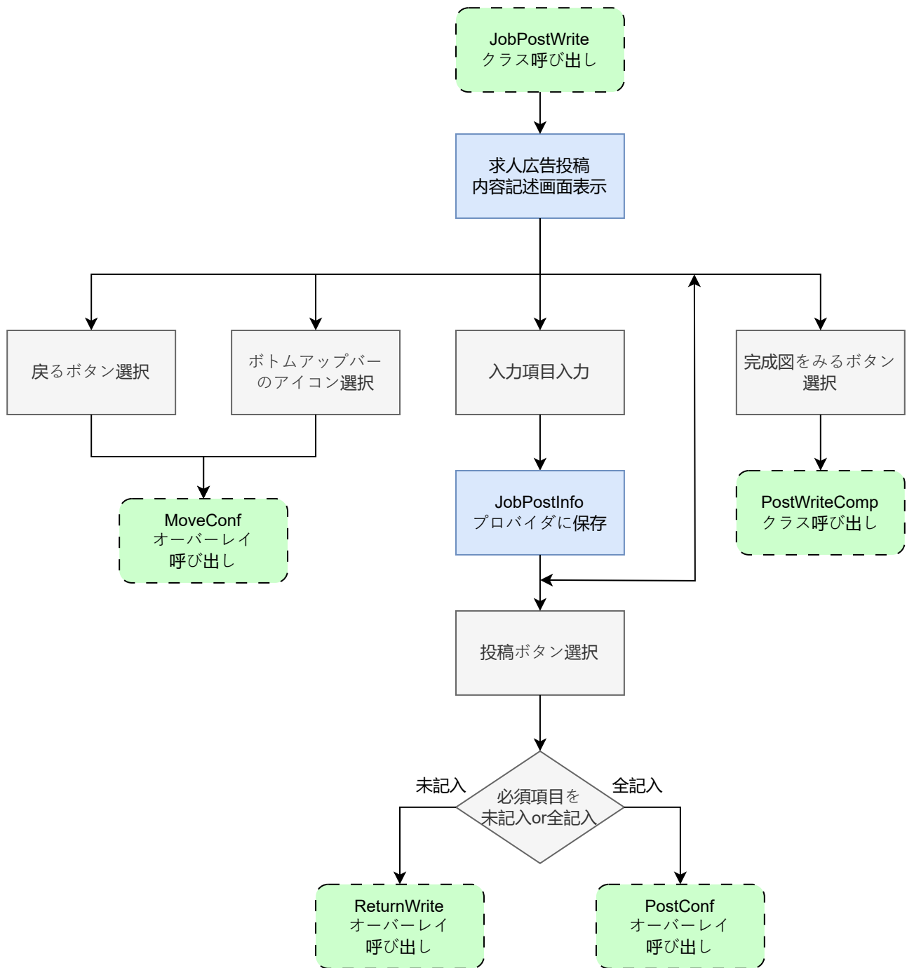
図 37: job_post_write.dart の状態遷移図
