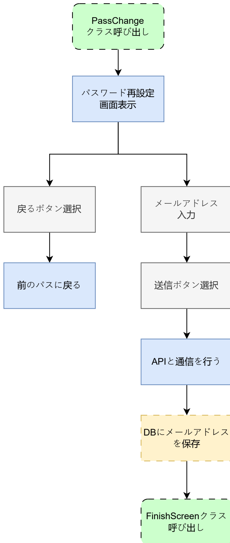
図 34: pass_change.dart の状態遷移図
