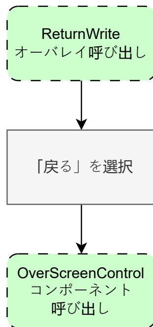
図 11: return_write.dart の状態遷移図
