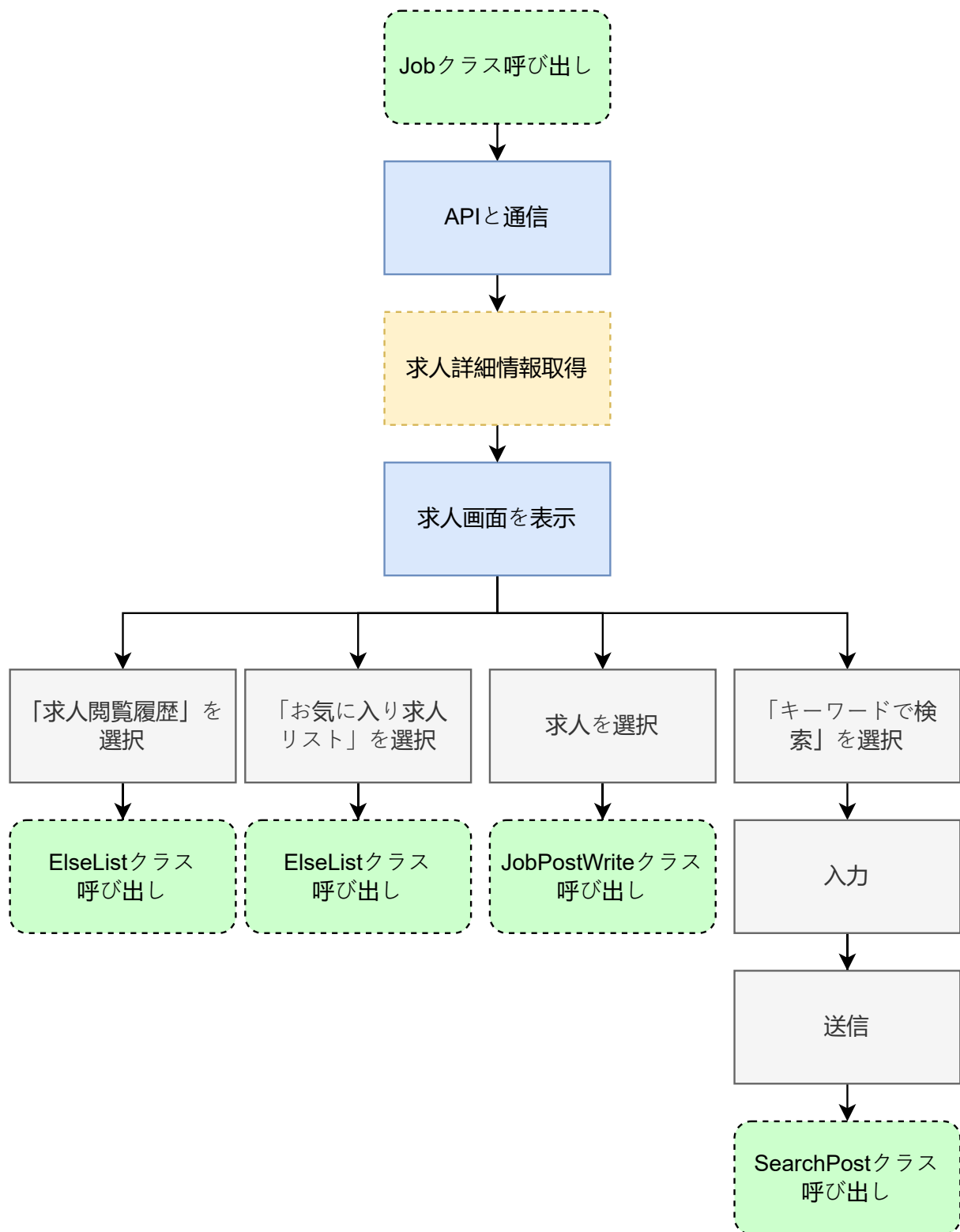
図 36: job.dart の状態遷移図
