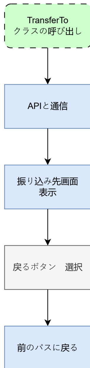
図 22: transfer_to.dart の状態遷移図
