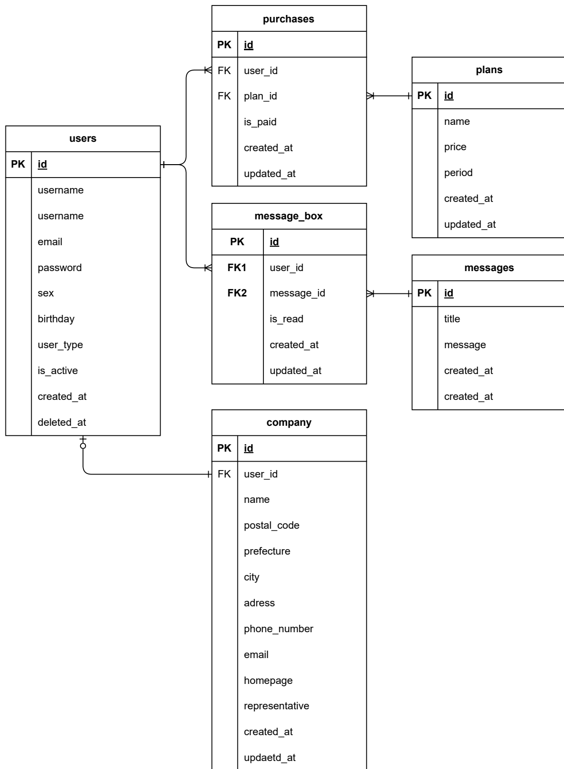
図 56: ER 図 (2)
