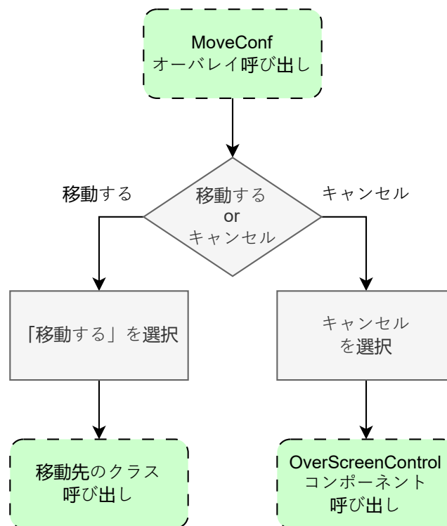
図 12: move_conf.dart の状態遷移図
