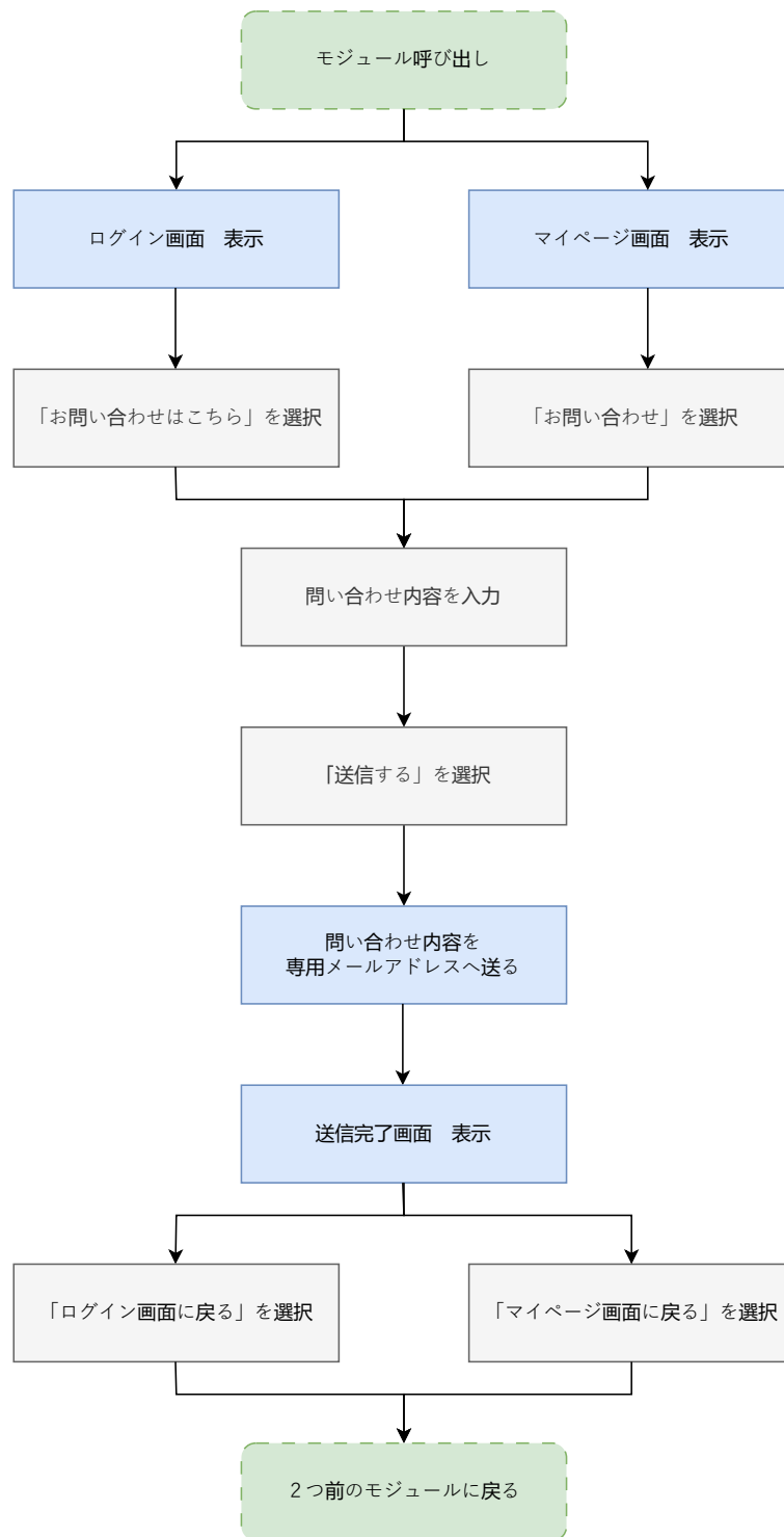
図 5: ask_page.dart の状態遷移図
