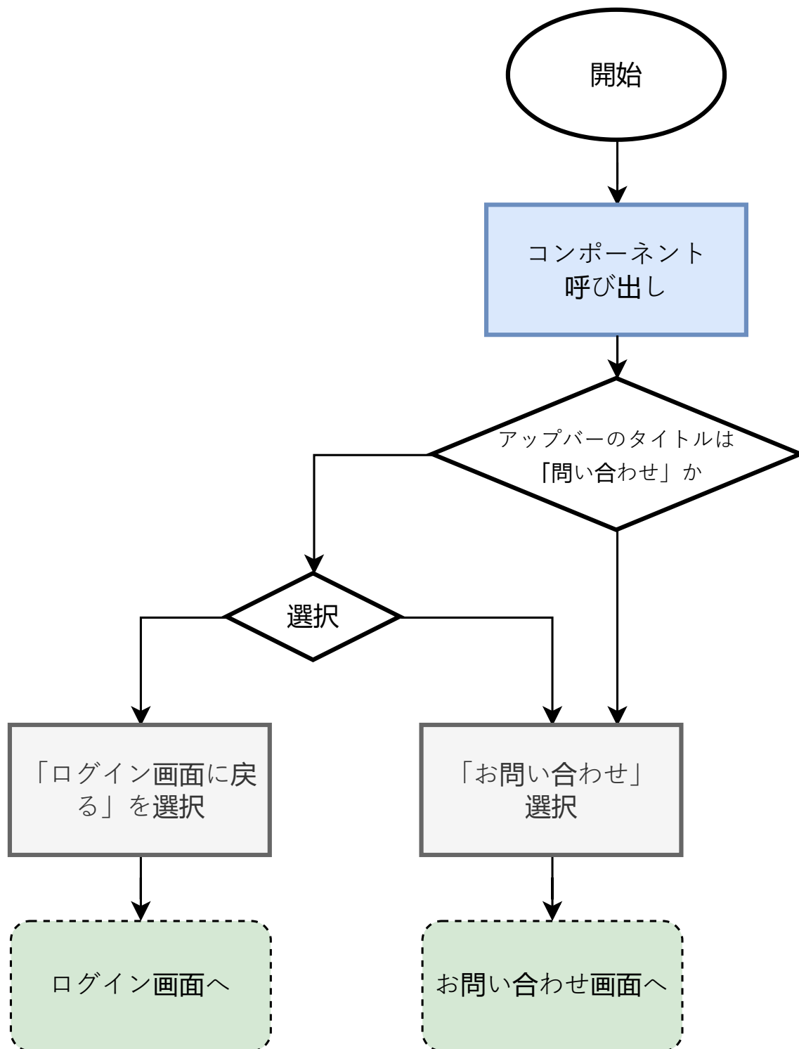
図 6: finish_screen.dart の状態遷移図
