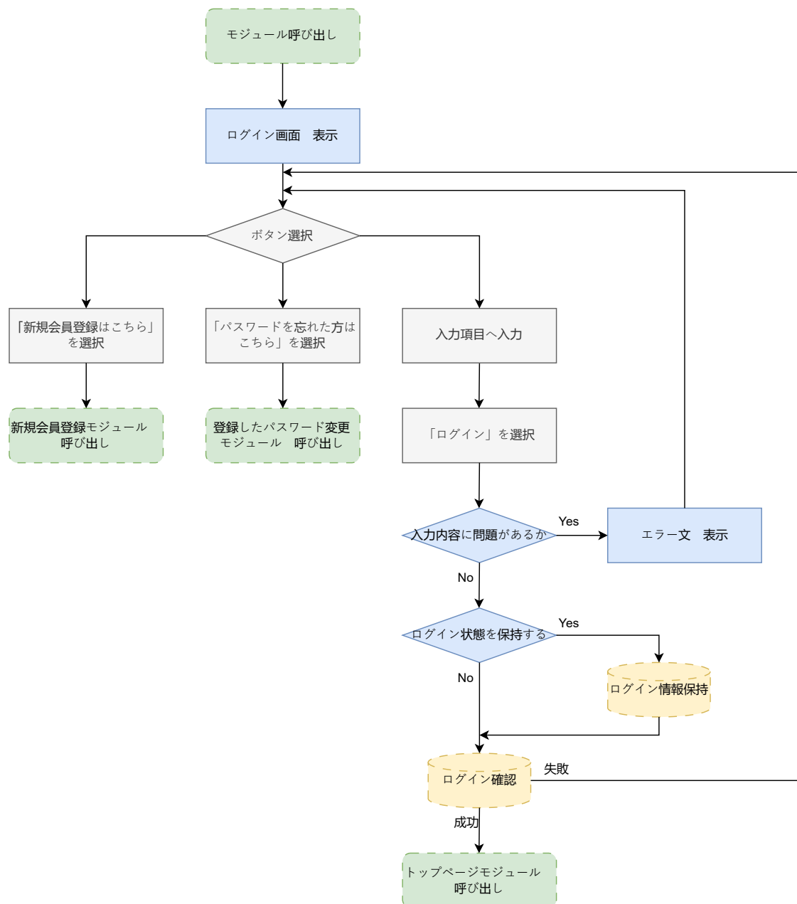
図 1: login_page.dart の状態遷移図
