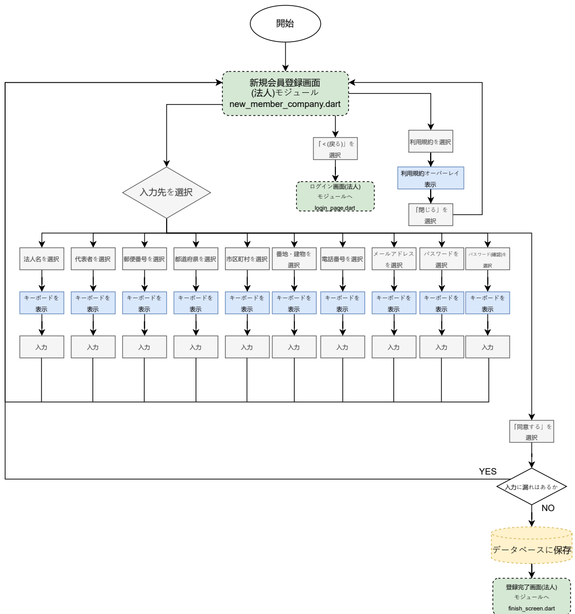
図 2: new_member_company.dart の状態遷移図
