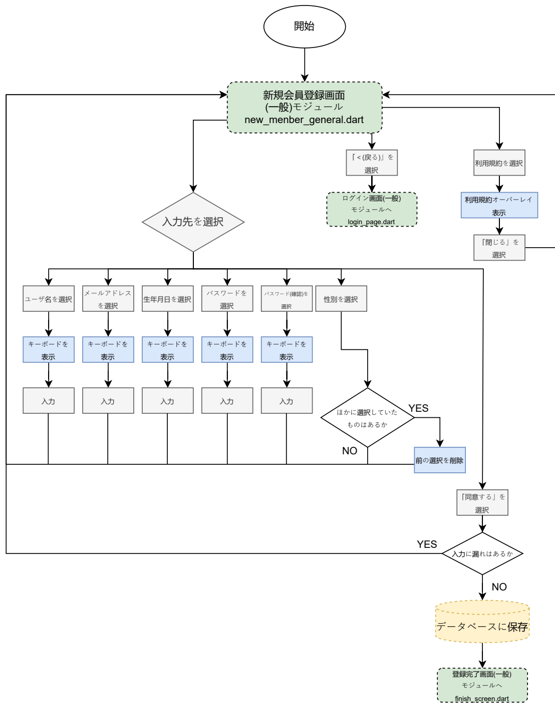
図 3: new_member_general.dart の状態遷移図
