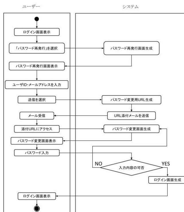
図 23: パスワード再発行機能
