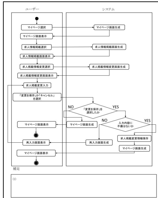
図 26: 求人情報変更機能
