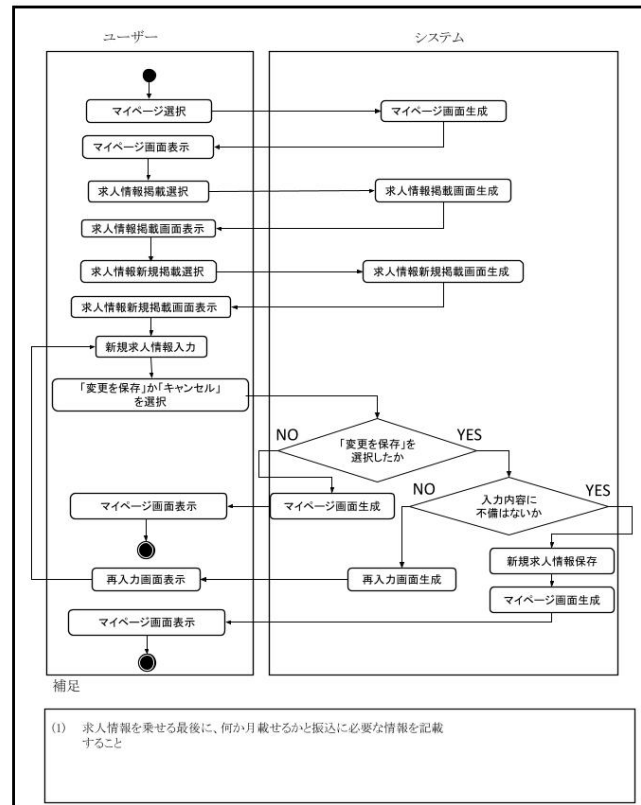
図 25: 求人情報新規掲載機能
