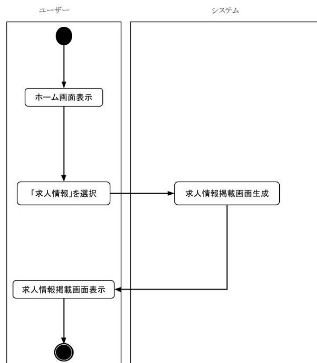
図 7: 求人情報機能
