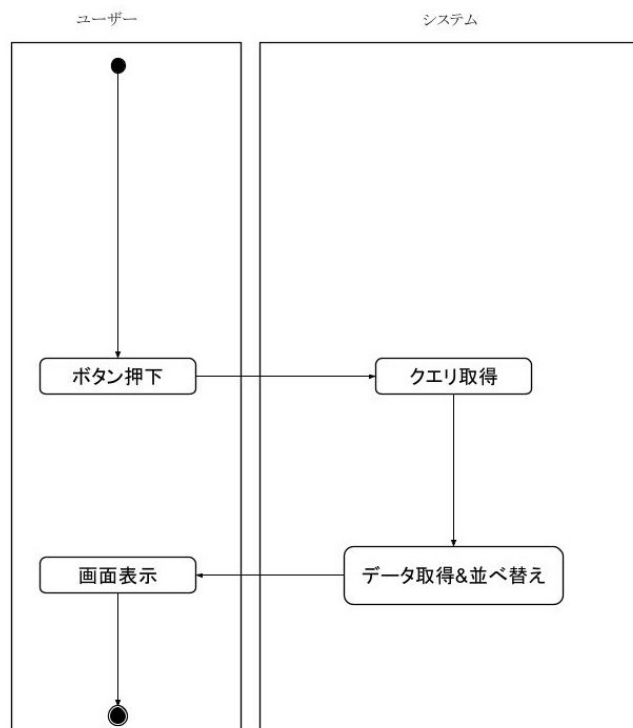
図 9: 表示順変更機能
