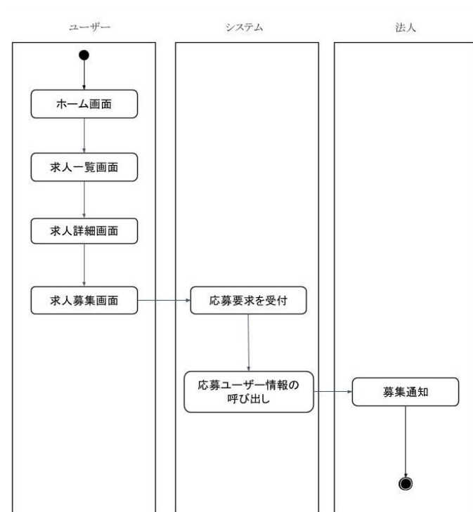
図 17: 求人応募機能
