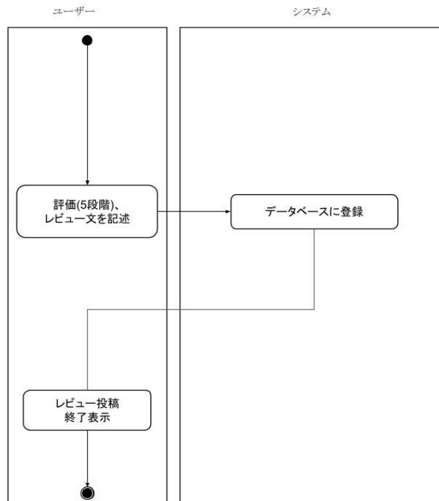
図 13: レビュー評価機能
