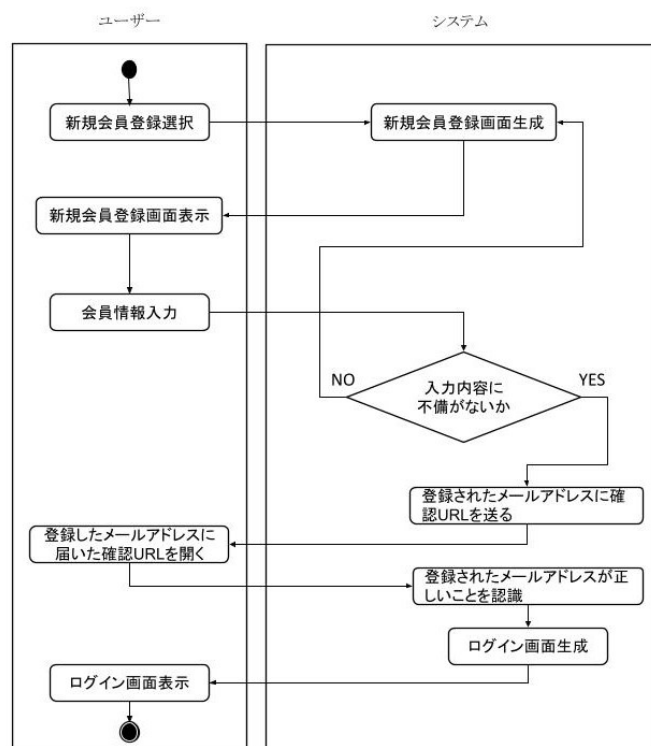
図 1: 新規会員登録機能
