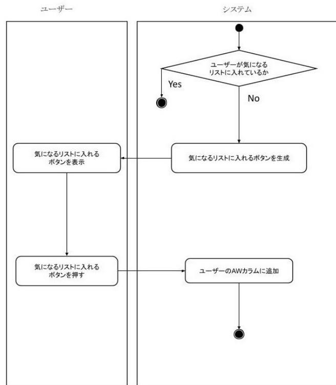
図 10: ブックマーク（登録）機能
