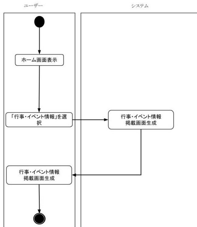
図 8: 行事・イベント情報表示機能
