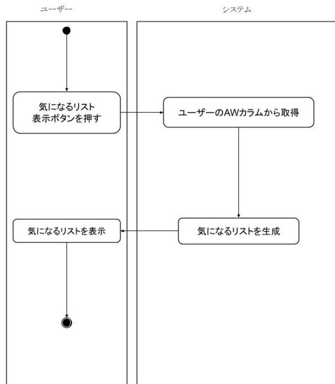
図 12: ブックマーク（表示）機能
