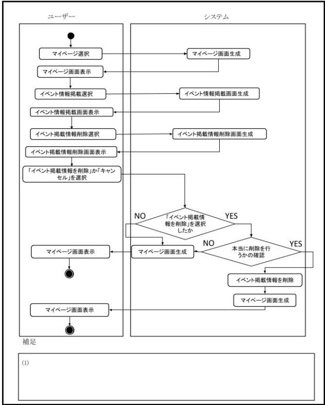
図 30: イベント・行事情報削除機能
