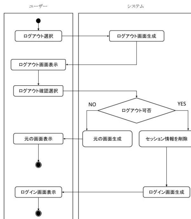
図 21: ログアウト機能
