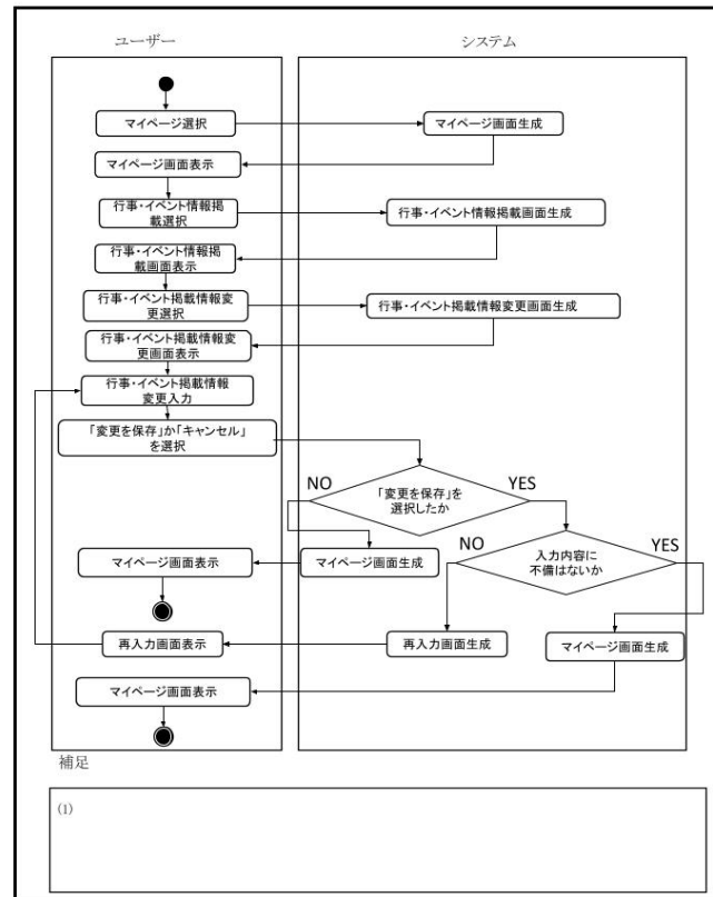
図 29: イベント・行事情報変更機能
