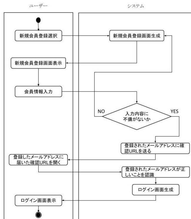
図 19: 新規会員登録機能
