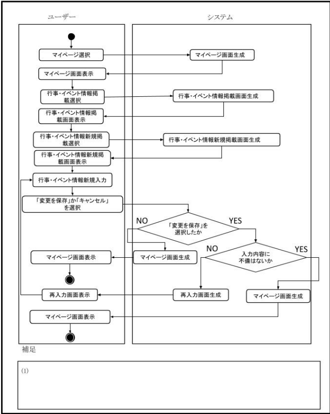
図 28: イベント・行事情報新規掲載機能
