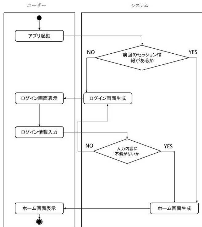
図 20: ログイン機能
