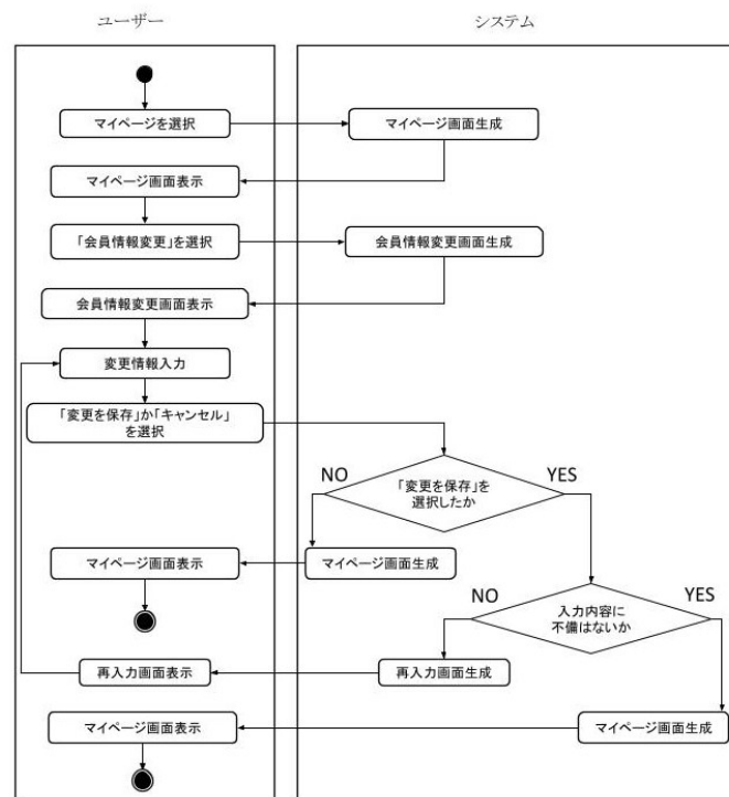
図 6: 会員情報確認・変更機能
