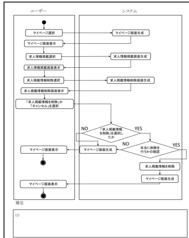
図 27: 求人情報削除機能
