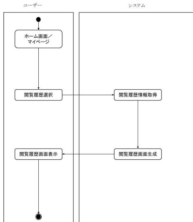
図 16: 閲覧履歴機能
