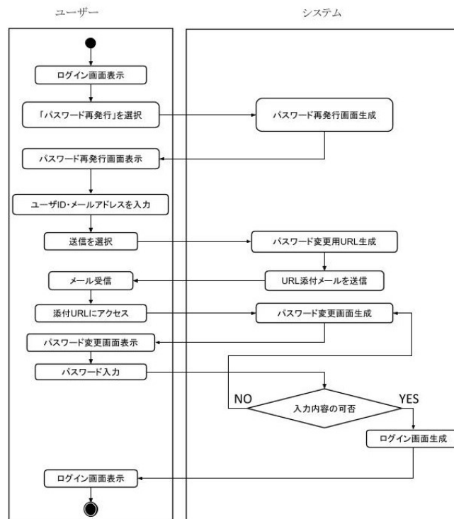
図 5: パスワード再発行機能
