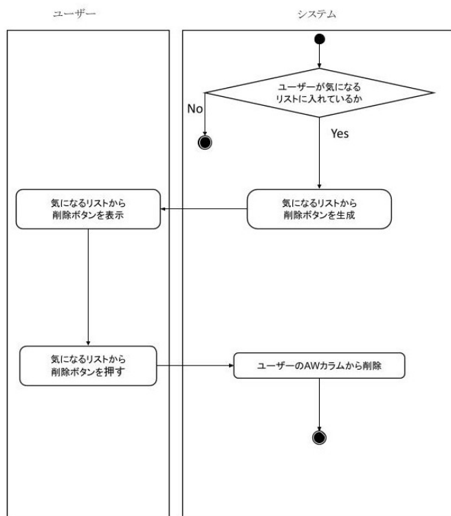
図 11: ブックマーク（削除）機能
