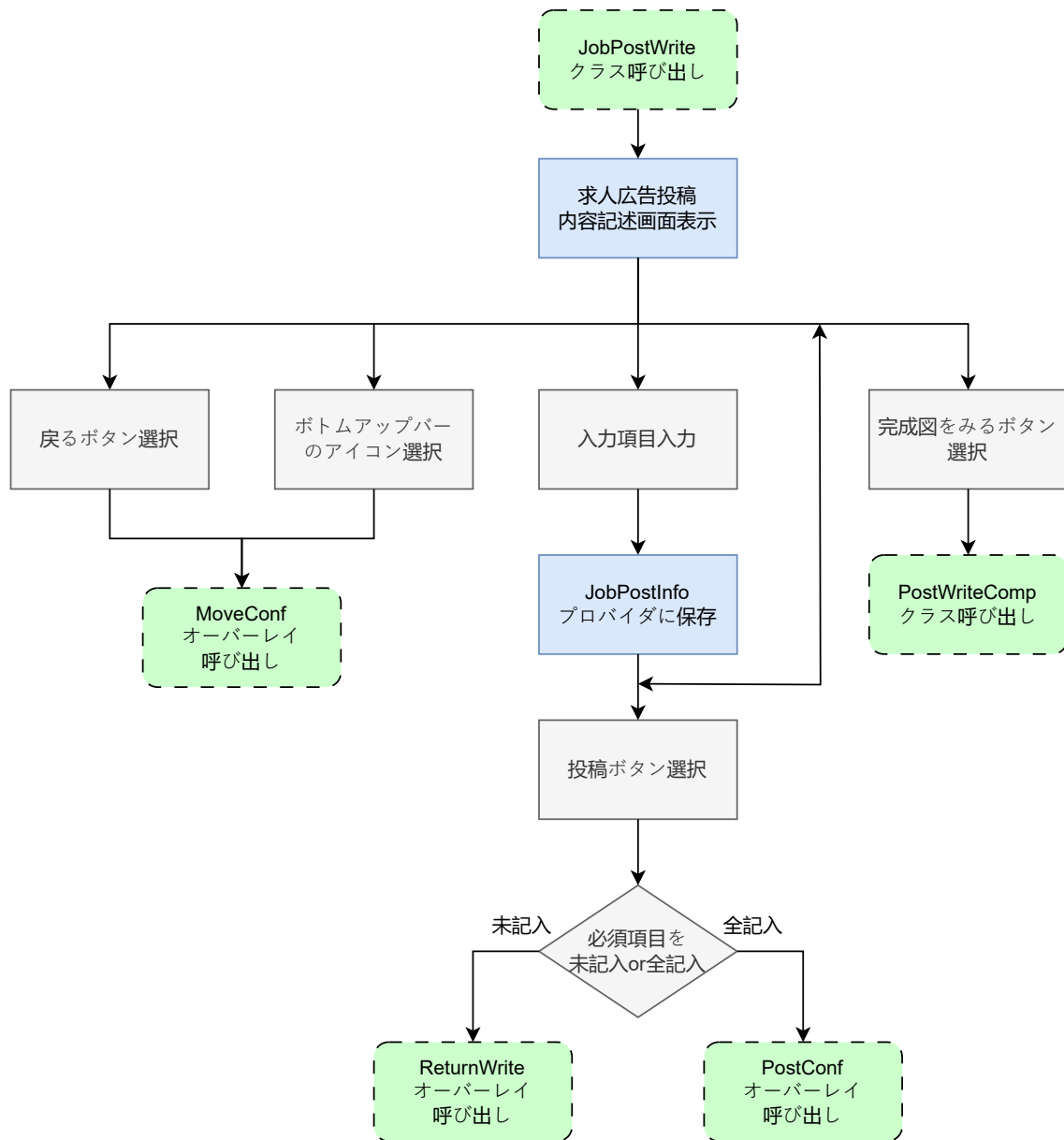
図 20: job_post_write.dart の状態遷移図
