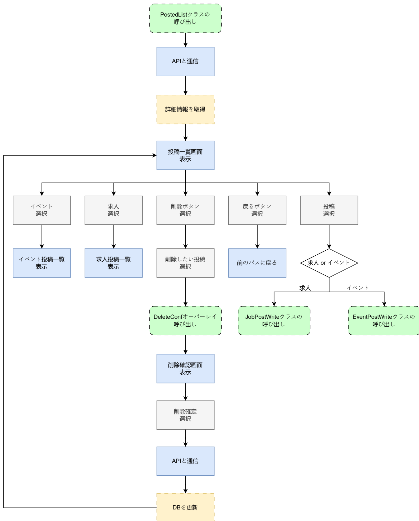
図 29: posted.list.dart の状態遷移図
