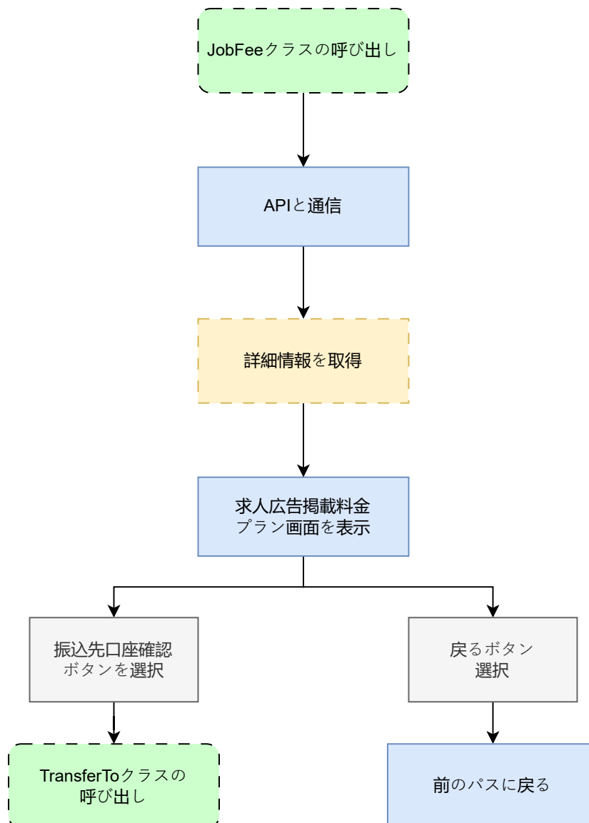
図 10: job_fee.dart の状態遷移図
