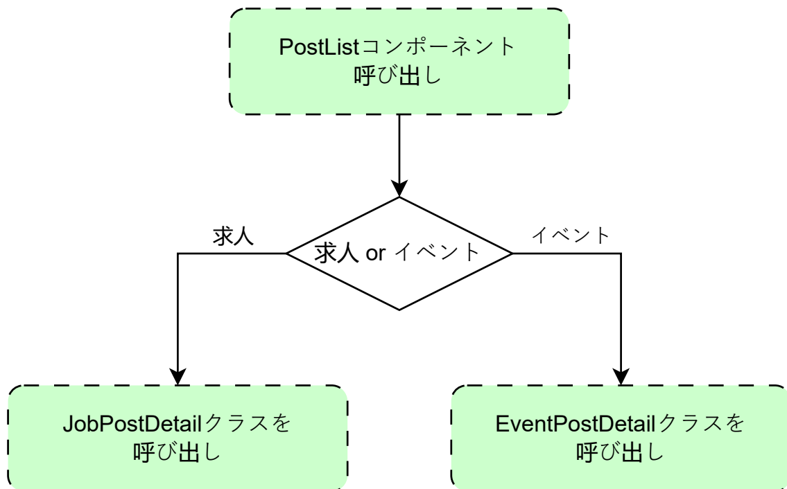
図 32: post_list.dart の状態遷移図
