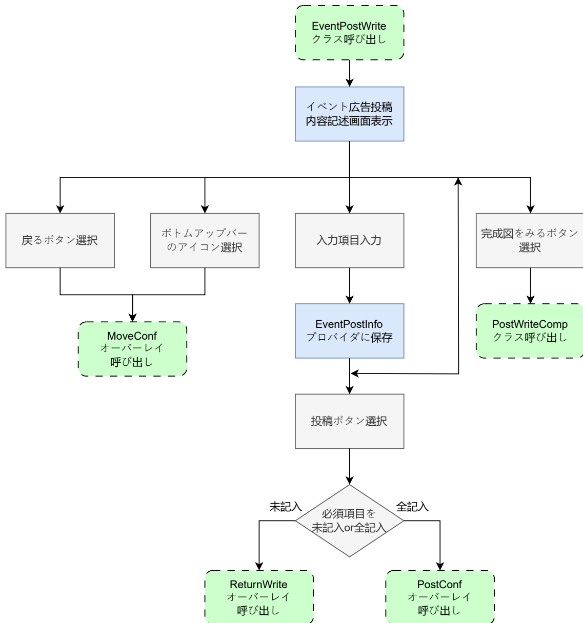
図 30: event_post_write.dart の状態遷移図
