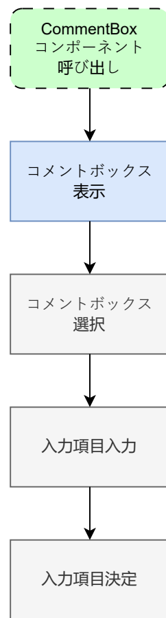
図 35: coment_box.dart の状態遷移図
