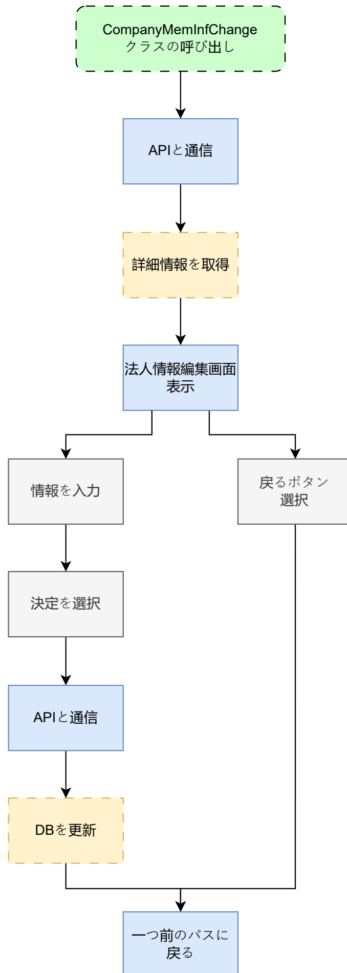
図 7: company_mem_inf_change.dart の状態遷移図
