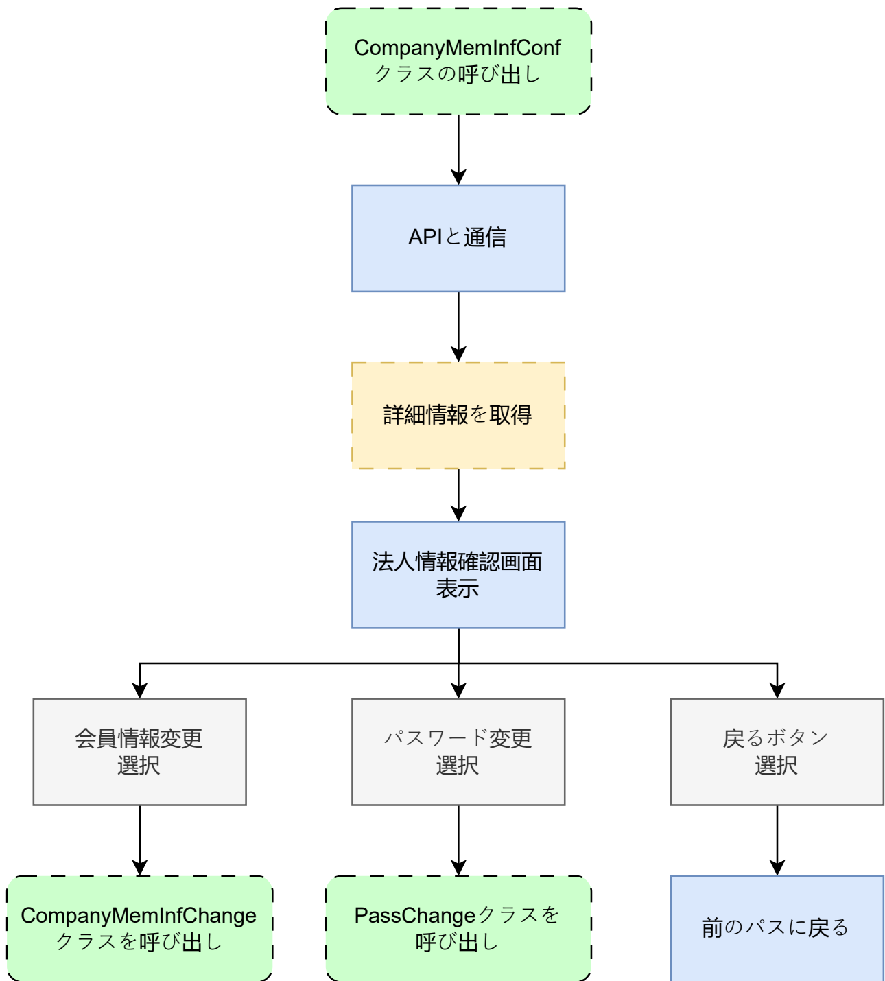
図 6: company_mem_inf_conf.dart の状態遷移図
