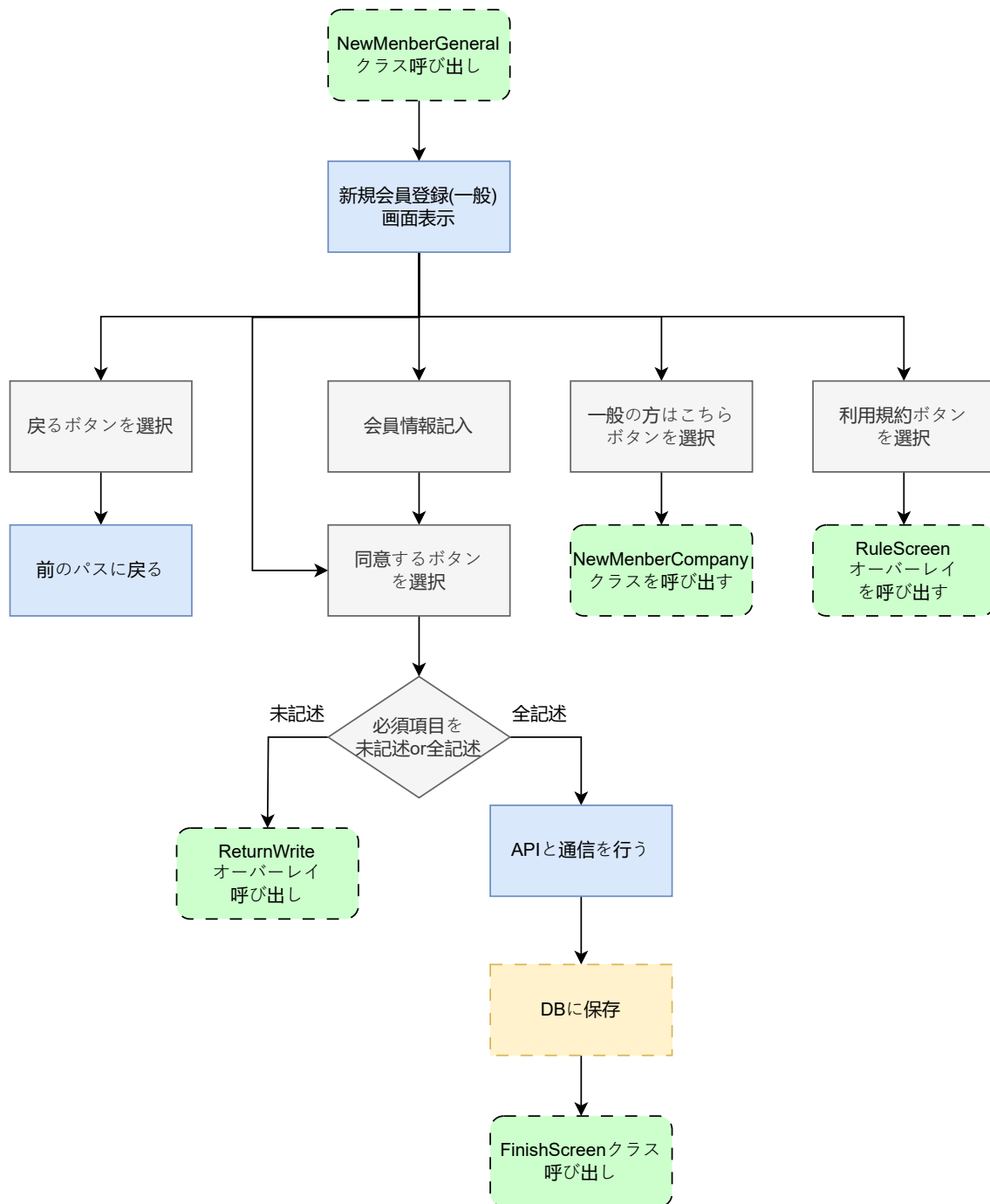
図 16: new_member_general.dart の状態遷移図
