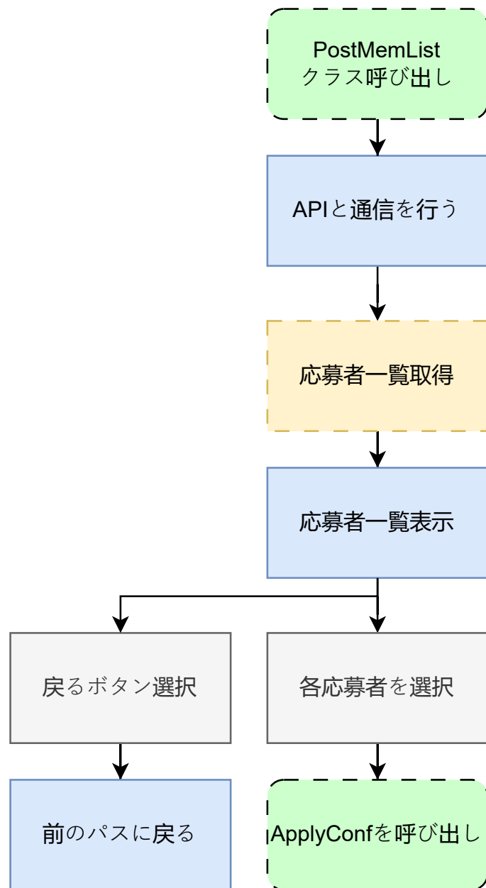
図 12: post_mem_list.dart の状態遷移図
