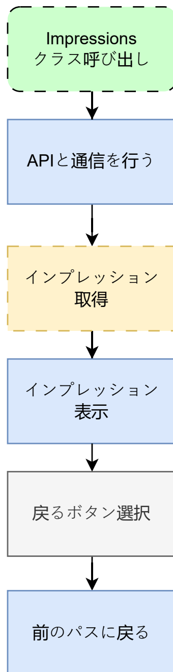
図 13: impressions.dart の状態遷移図
