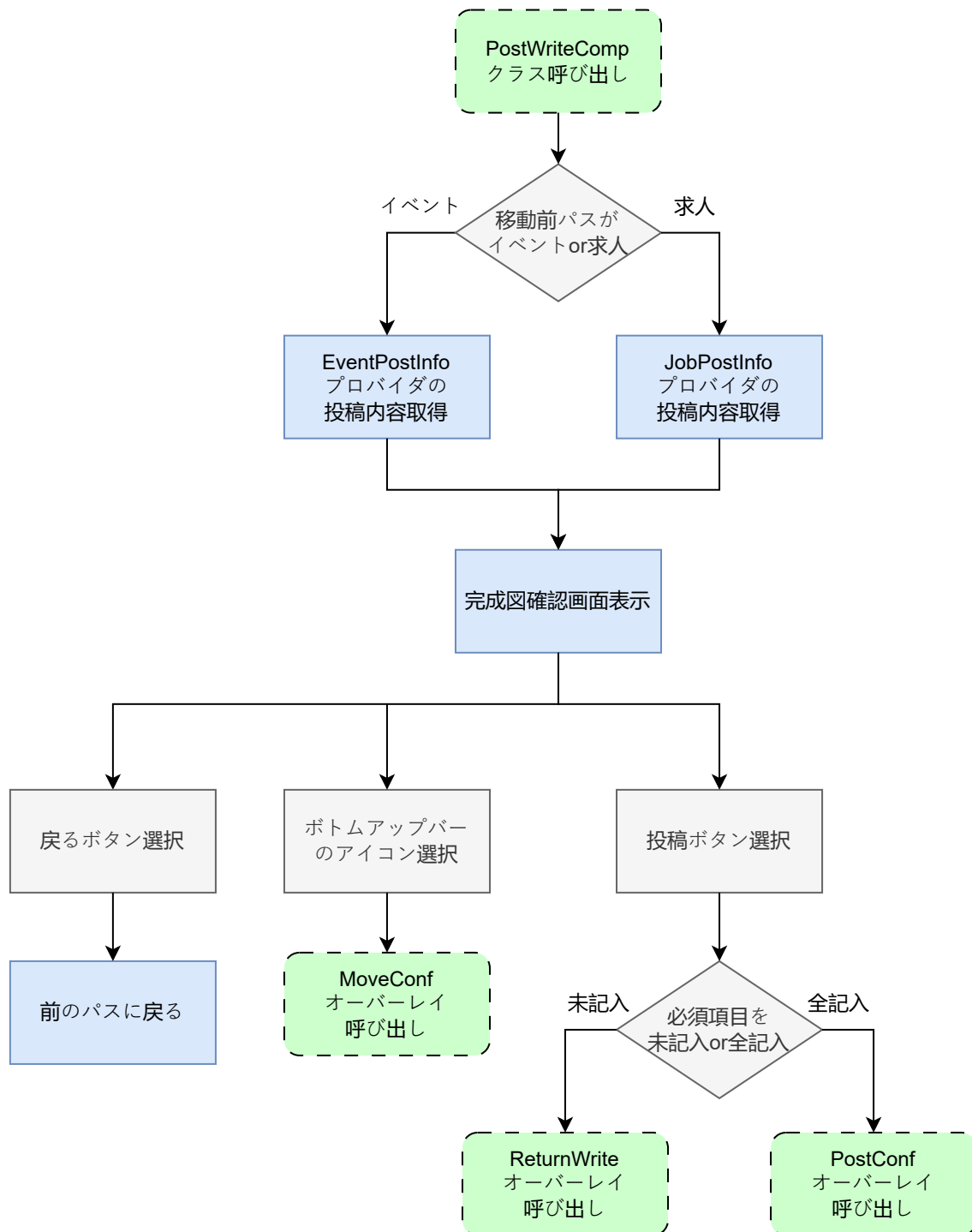
図 31: post_write_comp.dart の状態遷移図
