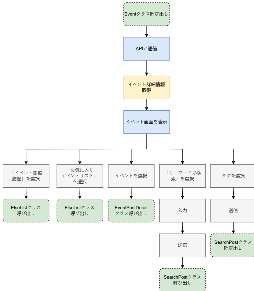
図 28: event.dart の状態遷移図
