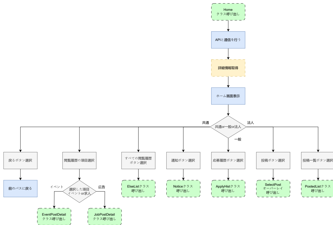
図 22: home.dart の状態遷移図
