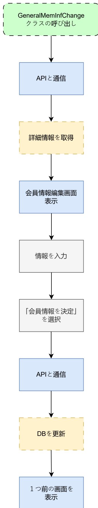
図 3: general_mem_inf_change.dart の状態遷移図
