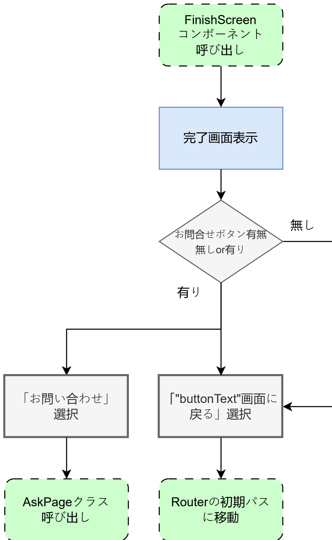
図 34: finish_screen.dart の状態遷移図
