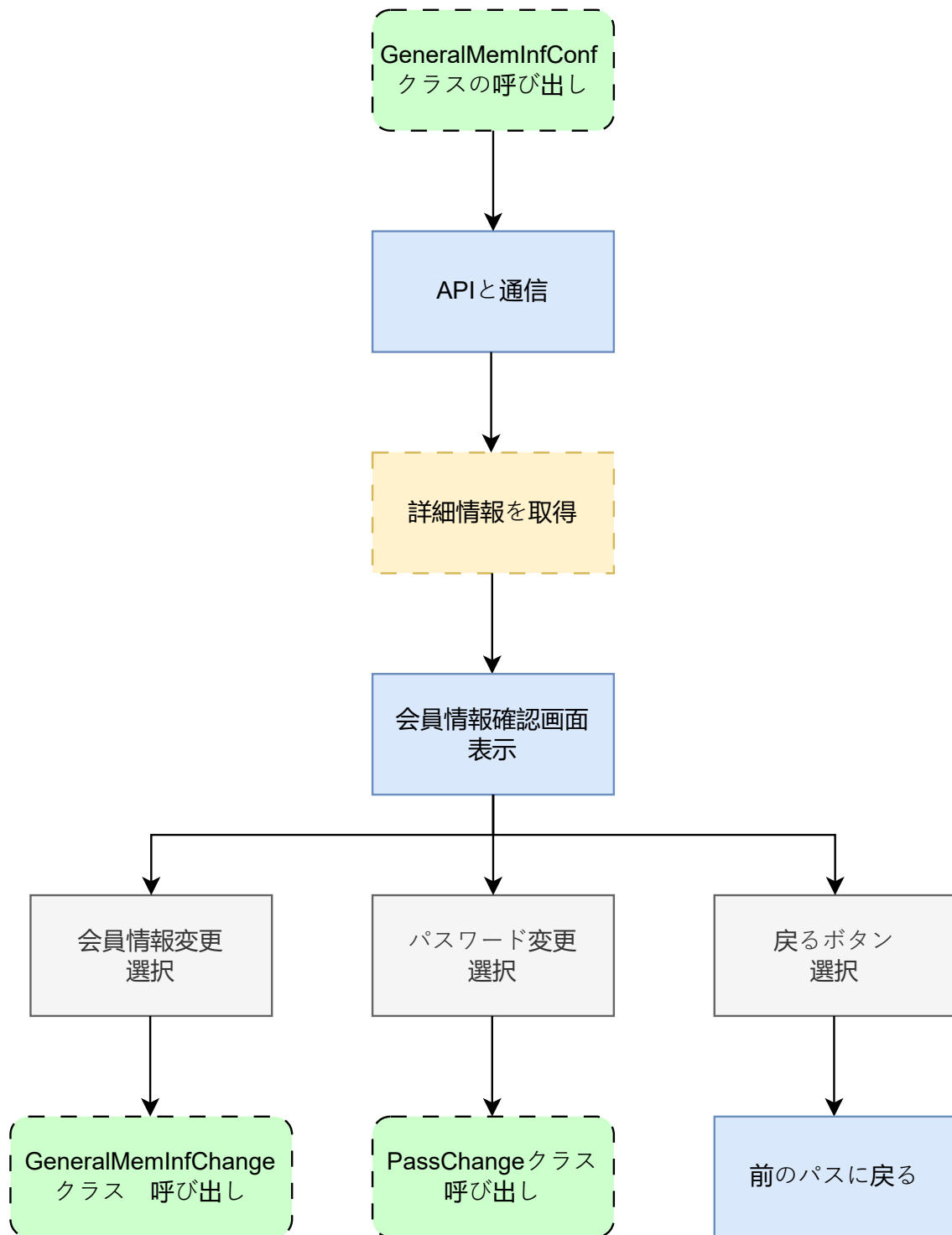
図 2: general_mem_inf_conf.dart の状態遷移図
