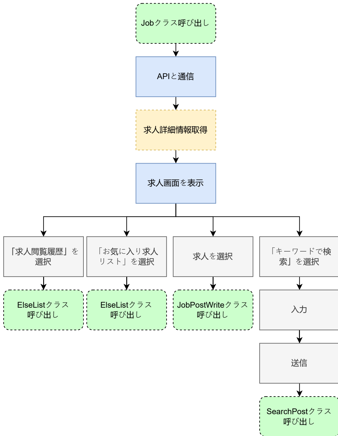
図 19: job.dart の状態遷移図
