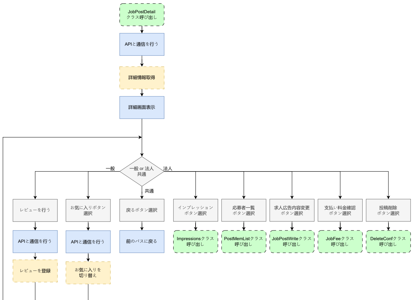
図 21: job_post_detail.dart の状態遷移図
