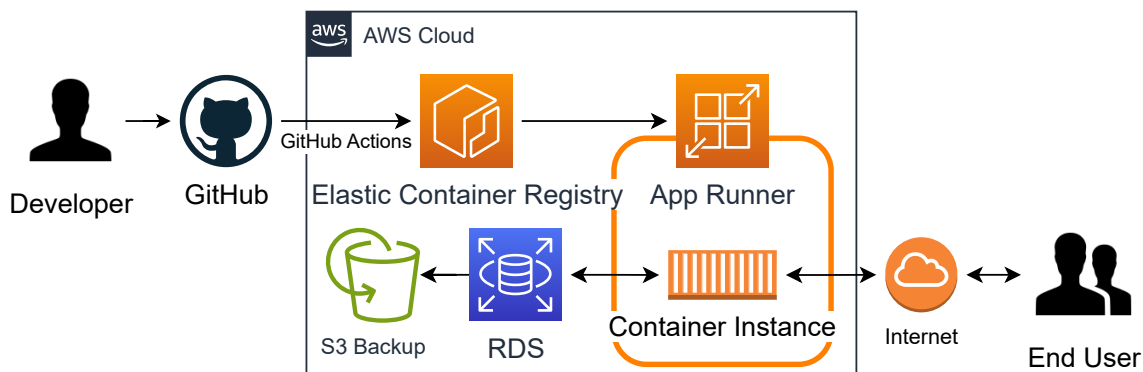
図 113: ネットワーク構成図
