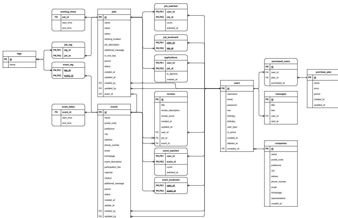
図 114: ER 図
