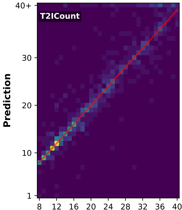
FSC-147
